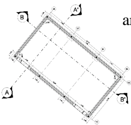
Plano de cimientos de área de mantenimiento y recepción de materia prima
