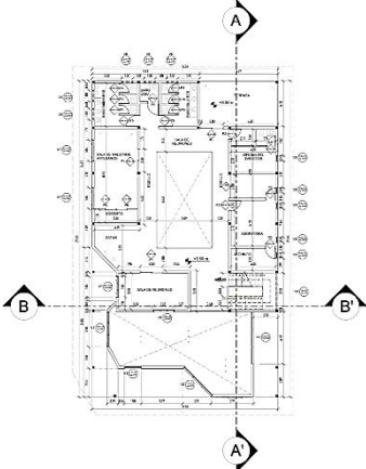
Área administrativa planta alta acotada
