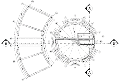
Plano de cimientos zona de aprendizaje teórico
