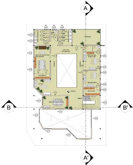
Área administrativa planta alta amoblada
