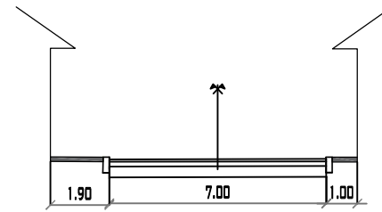
CALLE GILBERTO SAAVEDRA PROGRESIVA 0+650 MUNICIPIO DE PADCAYA ESC: 1/200
