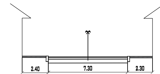
CALLE 2 PROGRESIVA 0+110 MUNICIPIO DE PADCAYA ESC: 1/200
