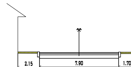
CALLE GILBERTO SAAVEDRA PROGRESIVA 1+310 MUNICIPIO DE PADCAYA ESC: 1/200
