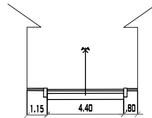
CALLE CAMPERO PROGRESIVA 0+100 MUNICIPIO DE PADCAYA ESC: 1/200
