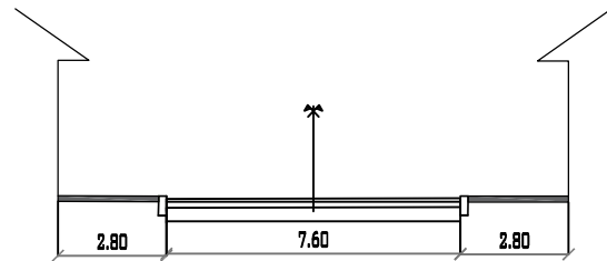
CALLE 2 PROGRESIVA 0+015 MUNICIPIO DE PADCAYA ESC: 1/200
