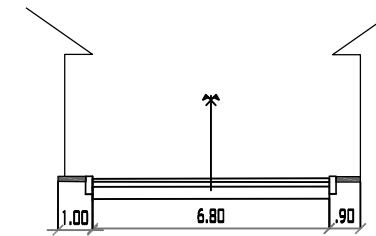
CALLE 7 PROGRESIVA 0+230 MUNICIPIO DE PADCAYA ESC: 1/200
