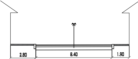
AVENIDA ANICETO ARCE PROGRESIVA 0+715 MUNICIPIO DE PADCAYA ESC: 1/200
