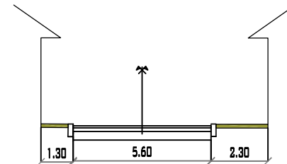
CALLE 8 PROGRESIVA 0+110 MUNICIPIO DE PADCAYA ESC:1/200
