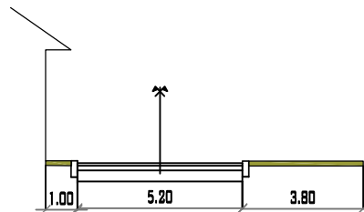
CALLE 8 PROGRESIVA 0+245 MUNICIPIO DE PADCAYA ESC:1/200
