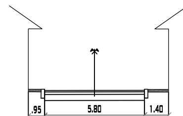
CALLE GILBERTO SAAVEDRA PROGRESIVA 1+000 MUNICIPIO DE PADCAYA ESC: 1/200
