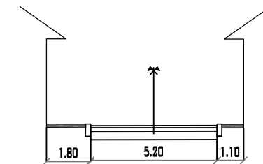
CALLE CAMPERO PROGRESIVA 0+055 MUNICIPIO DE PADCAYA ESC: 1/200
