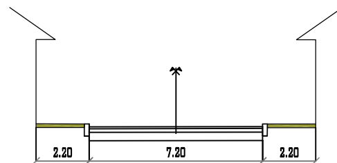
AVENIDA ANICETO ARCE PROGRESIVA 0+085 MUNICIPIO DE PADCAYA ESC: 1/200
