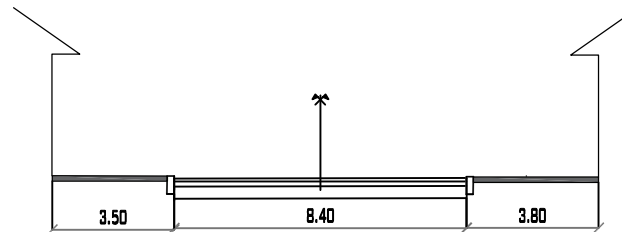
AVENIDA ANICETO ARCE PROGRESIVA 0+880 MUNICIPIO DE PADCAYA ESC: 1/200
