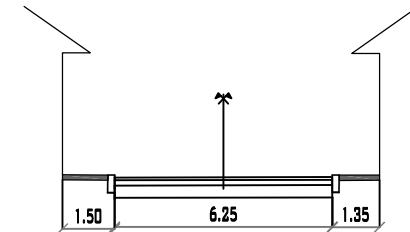
CALLE GILBERTO SAAVEDRA PROGRESIVA 1+045 MUNICIPIO DE PADCAYA ESC: 1/200
