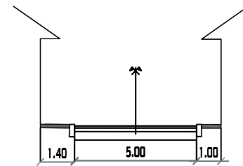
CALLE 6 PROGRESIVA 0+055 MUNICIPIO DE PADGAYA ESC:1/200
