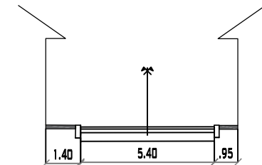
CALLE 9 PROGRESIVA 0+045 MUNICIPIO DE PADCAYA ESC:1/200
