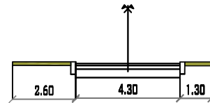
CALLE 8 PROGRESIVA 0+180 MUNICIPIO DE PADCAYA ESC:1/200
