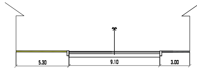
CALLE 6 PROGRESIVA 0+100 MUNICIPIO DE PADGAYA ESC:1/200
