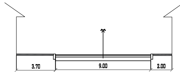
CALLE 6 PROGRESIVA 0+135 MUNICIPIO DE PADGAYA ESC:1/200
