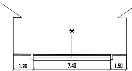
CALLE 1 PROGRESIVA 0+160 MUNICIPIO DE PADCAYA ESC: 1/200
