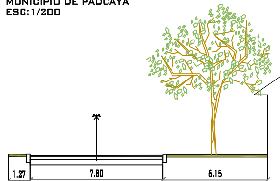
CALLE YAMPARAEZ PROGRESIVA 1+120 MUNICIPIO DE PADCAYA ESC: 1/200
