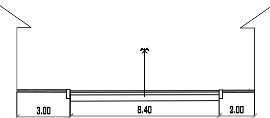
AVENIDA ANICETO ARCE PROGRESIVA 0+765 MUNICIPIO DE PADCAYA ESC: 1/200
