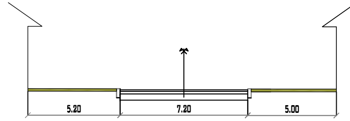
CALLE 6 PROGRESIVA 0+070 MUNICIPIO DE PADGAYA ESC:1/200
