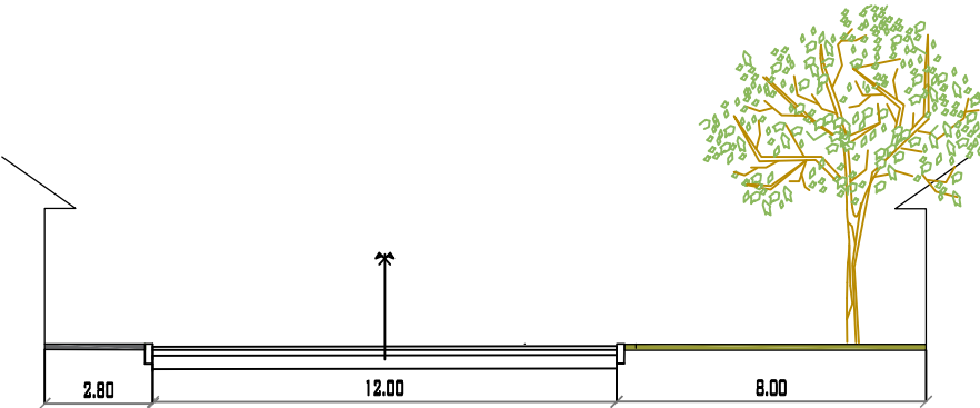
AVENIDA ANICETO ARCE PROGRESIVA 0+855 MUNICIPIO DE PADCAYA ESC: 1/200
