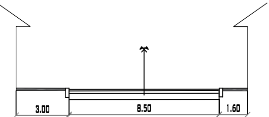
AVENIDA ANICETO ARCE PROGRESIVA 0+830 MUNICIPIO DE PADCAYA ESC: 1/200
