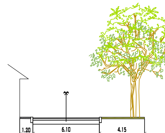
CALLE ANTONIO JOSE DE SUCRE PROGRESIVA 0+300 MUNICIPIO DE PADCAYA ESC: 1/200
