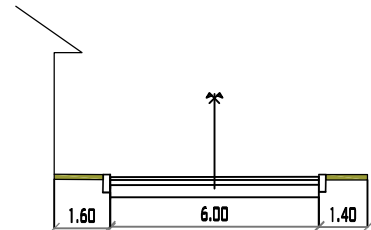
CALLE ANTONIO JOSE DE SUCRE PROGRESIVA 0+000 MUNICIPIO DE PADCAYA ESC: 1/200
