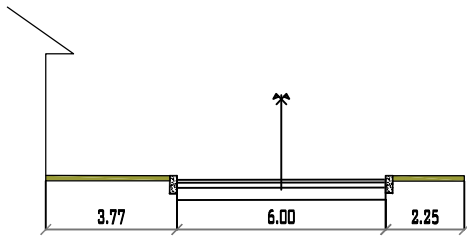
AVENIDA TARIJA PROGRESIVA 0+050 MUNICIPIO DE PADCAYA ESC: 1/200
