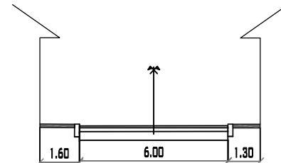
CALLE ANTONIO JOSE DE SUCRE PROGRESIVA 0+145 MUNICIPIO DE PADCAYA ESC: 1/200
