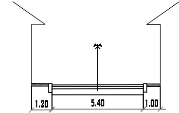
CALLE 9 PROGRESIVA 0+005 MUNICIPIO DE PADCAYA ESC:1/200
