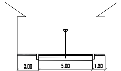
CALLE 10 PROGRESIVA 0+045 MUNICIPIO DE PADCAYA ESC:1/200
