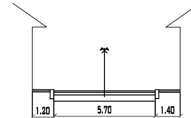
CALLE ANTONIO JOSE DE SUCRE PROGRESIVA 0+255 MUNICIPIO DE PADCAYA ESC: 1/200
