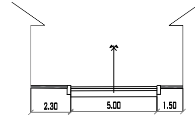
CALLE 10 PROGRESIVA 0+005 MUNICIPIO DE PADCAYA ESC:1/200
