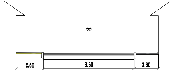
AVENIDA ANICETO ARCE PROGRESIVA 0+565 MUNICIPIO DE PADCAYA ESC: 1/200
