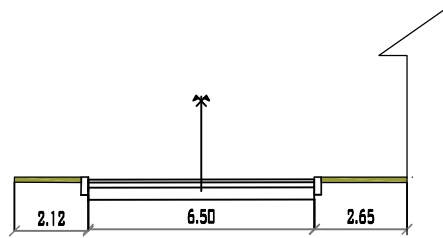
AVENIDA TARIJA PROGRESIVA 0+195 MUNICIPIO DE PADCAYA ESC: 1/200
