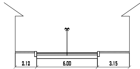
AVENIDA TARIJA PROGRESIVA 0+150 MUNICIPIO DE PADCAYA ESC: 1/200
