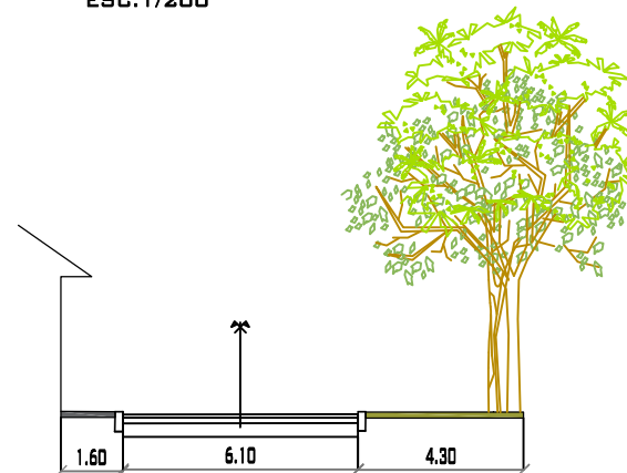
CALLE CAMPERO PROGRESIVA 0+160 MUNICIPIO DE PADCAYA ESC: 1/200
