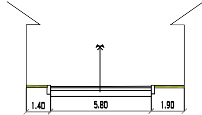
CALLE 8 PROGRESIVA 0+080 MUNICIPIO DE PADCAYA ESC:1/200
