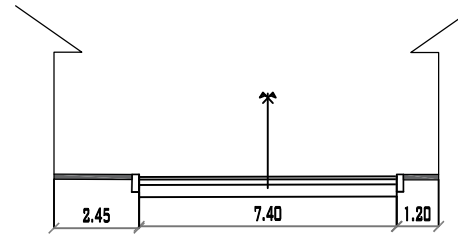
CALLE GILBERTO SAAVEDRA PROGRESIVA 0+600 MUNICIPIO DE PADCAYA ESC: 1/200
