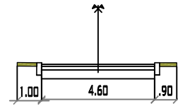
CALLE 8 PROGRESIVA 0+225 MUNICIPIO DE PADCAYA ESC:1/200
