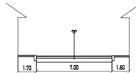
CALLE 1 PROGRESIVA 0+075 MUNICIPIO DE PADCAYA ESC: 1/200
