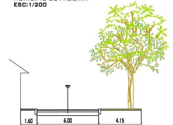
CALLE ANTONIO JOSE DE SUCRE PROGRESIVA 0+350 MUNICIPIO DE PADCAYA
