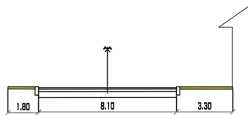
AVENIDA ANICETO ARCE PROGRESIVA 0+040 MUNICIPIO DE PADCAYA ESC: 1/200
