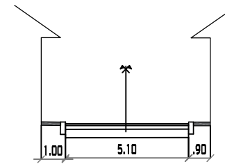
CALLE 5 PROGRESIVA 0+010 MUNICIPIO DE PADGAYA ESC:1/200
