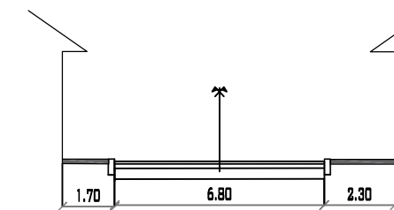
CALLE 4 PROGRESIVA 0+115 MUNICIPIO DE PADCAYA ESC: 1/200
