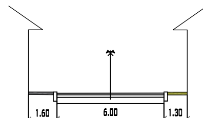
CALLE ANTONIO JOSE DE SUCRE PROGRESIVA 0+100 MUNICIPIO DE PADCAYA ESC: 1/200
