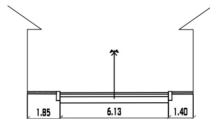
CALLE GILBERTO SAAVEDRA PROGRESIVA 0+970 MUNICIPIO DE PADCAYA ESC: 1/200
