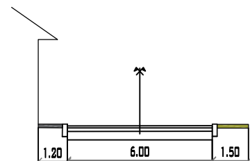
CALLE ANTONIO JOSE DE SUCRE PROGRESIVA 0+175 MUNICIPIO DE PADCAYA ESC: 1/200
