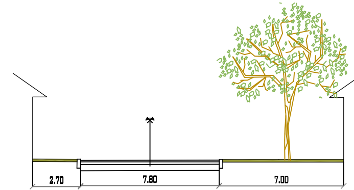
CALLE YAMPARAEZ PROGRESIVA 1+170 MUNICIPIO DE PADCAYA ESC: 1/200
