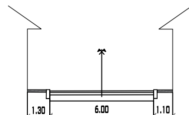
CALLE ANTONIO JOSE DE SUCRE PROGRESIVA 0+215 MUNICIPIO DE PADCAYA ESC: 1/200
