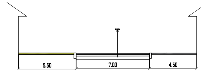
AVENIDA ANICETO ARCE PROGRESIVA 0+390 MUNICIPIO DE PADCAYA ESC: 1/200
