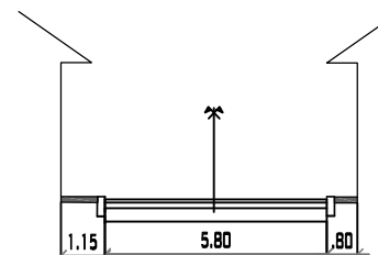
CALLE ANTONIO JOSE DE SUCRE PROGRESIVA 0+275 MUNICIPIO DE PADCAYA ESC: 1/200
