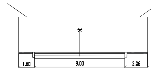
CALLE 7 PROGRESIVA 0+320 MUNICIPIO DE PADCAYA ESC: 1/200
