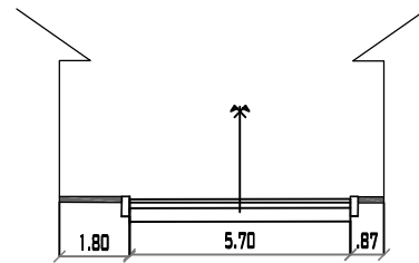
CALLE CAMPERO PROGRESIVA 0+000 MUNICIPIO DE PADCAYA ESC: 1/200
