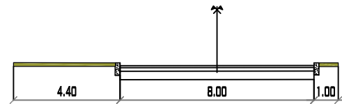
AVENIDA ANICETO ARCE PROGRESIVA 0+000 MUNICIPIO DE PADCAYA ESC: 1/200
