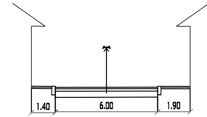
CALLE GILBERTO SAAVEDRA PROGRESIVA 0+830 MUNICIPIO DE PADCAYA ESC: 1/200
