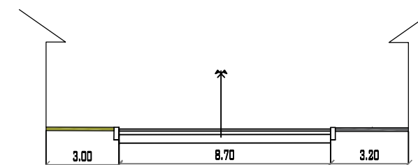
CALLE ANICETO ARCE PROGRESIVA 0+470 MUNICIPIO DE PADCAYA ESC: 1/200
