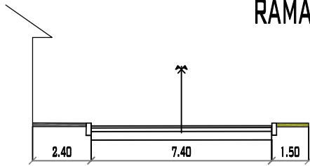
AVENIDA TARIJA PROGRESIVA 0+305 MUNICIPIO DE PADCAYA ESC: 1/200
