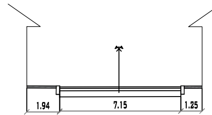
CALLE GILBERTO SAAVEDRA PROGRESIVA 0+685 MUNICIPIO DE PADCAYA ESC: 1/200
