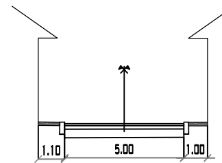
CALLE 5 PROGRESIVA 0+085 MUNICIPIO DE PADGAYA ESC:1/200
