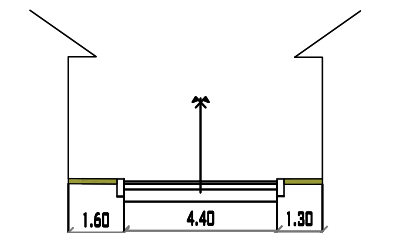
CALLE 8 PROGRESIVA 0+155 MUNICIPIO DE PADCAYA ESC:1/200
