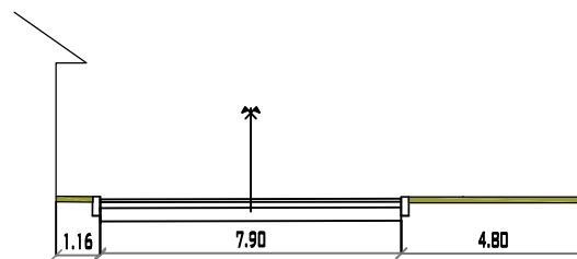
AVENIDA TARIJA PROGRESIVA 0+555 MUNICIPIO DE PADCAYA ESC: 1/200
