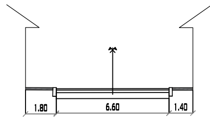
AVENIDA TARIJA PROGRESIVA 0+505 MUNICIPIO DE PADCAYA ESC: 1/200
