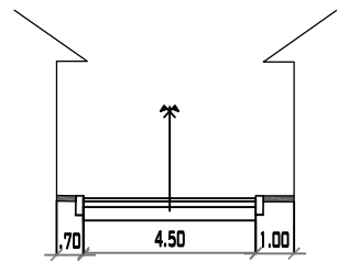
CALLE 6 PROGRESIVA 0+030 MUNICIPIO DE PADGAYA ESC:1/200
