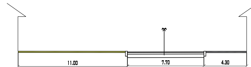
AVENIDA ANICETO ARCE PROGRESIVA 0+435 MUNICIPIO DE PADCAYA ESC: 1/200
