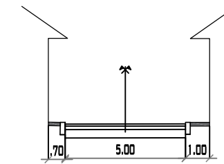
CALLE 5 PROGRESIVA 0+055 MUNICIPIO DE PADGAYA ESC:1/200
