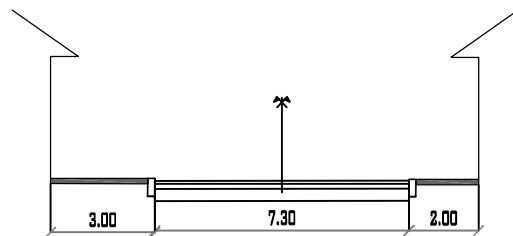
CALLE 2 PROGRESIVA 0+055 MUNICIPIO DE PADCAYA ESC: 1/200
