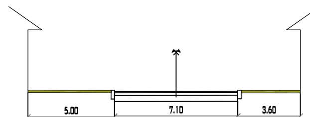
AVENIDA ANICETO ARCE PROGRESIVA 0+285 MUNICIPIO DE PADCAYA ESC: 1/200
