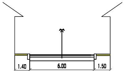
CALLE 8 PROGRESIVA 0+140 MUNICIPIO DE PADCAYA ESC:1/200
