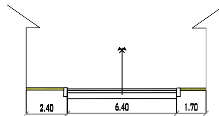
CALLE 4 PROGRESIVA 0+045 MUNICIPIO DE PADCAYA ESC: 1/200
