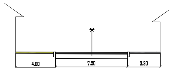
AVENIDA ANICETO ARCE PROGRESIVA 0+230 MUNICIPIO DE PADCAYA ESC: 1/200
