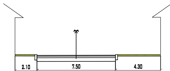
AVENIDA ANICETO ARCE PROGRESIVA 0+120 MUNICIPIO DE PADCAYA ESC: 1/200
