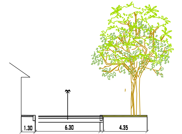
CALLE ANTONIO JOSE DE SUCRE PROGRESIVA 0+335 MUNICIPIO DE PADCAYA ESC: 1/200
