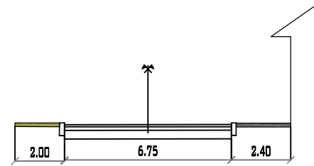
CALLE GILBERTO SAAVEDRA PROGRESIVA 0+875 MUNICIPIO DE PADCAYA ESC: 1/200
