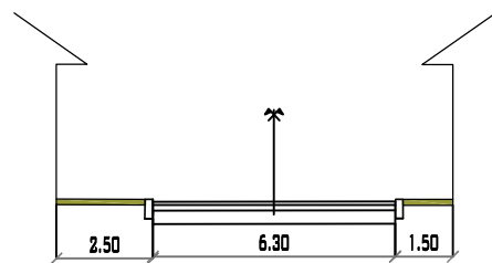
CALLE 4 PROGRESIVA 0+070 MUNICIPIO DE PADCAYA ESC: 1/200
