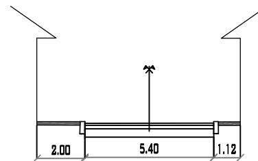
CALLE CAMPERO PROGRESIVA 0+025 MUNICIPIO DE PADCAYA ESC: 1/200
