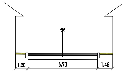
AVENIDA TARIJA PROGRESIVA 0+470 MUNICIPIO DE PADCAYA ESC: 1/200
