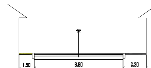
AVENIDA ANICETO ARCE PROGRESIVA 0+525 MUNICIPIO DE PADCAYA ESC: 1/200
