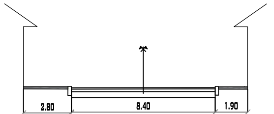
AVENIDA ANICETO ARCE PROGRESIVA 0+830 MUNICIPIO DE PADCAYA
