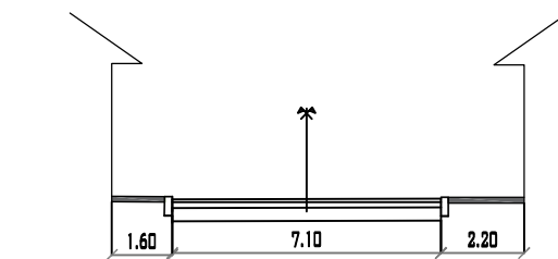
CALLE 2 PROGRESIVA 0+065 MUNICIPIO DE PADCAYA ESC: 1/200
