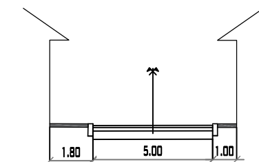
CALLE CAMPERO PROGRESIVA 0+085 MUNICIPIO DE PADCAYA ESC: 1/200
