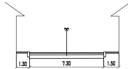
CALLE 4 PROGRESIVA 0+015 MUNICIPIO DE PADCAYA ESC: 1/200
