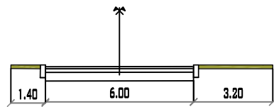
AVENIDA TARIJA PROGRESIVA 0+110 MUNICIPIO DE PADCAYA ESC: 1/200
