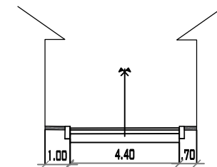
CALLE CAMPERO PROGRESIVA 0+135 MUNICIPIO DE PADCAYA ESC: 1/200
