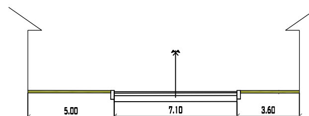
AVENIDA ANICETO ARCE PROGRESIVA 0+345 MUNICIPIO DE PADCAYA ESC: 1/200
