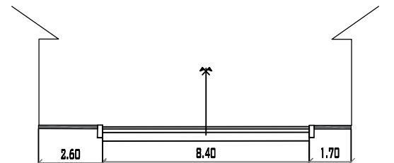
AVENIDA ANICETO ARCE PROGRESIVA 0+645 MUNICIPIO DE PADCAYA ESC: 1/200
