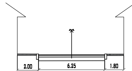
CALLE GILBERTO SAAVEDRA PROGRESIVA 1+085 MUNICIPIO DE PADCAYA ESC: 1/200
