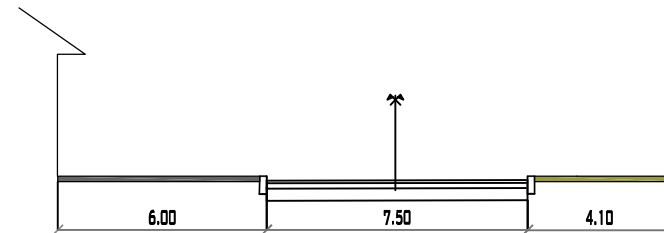
AVENIDA ANICETO ARCE PROGRESIVA 0+170 MUNICIPIO DE PADCAYA ESC: 1/200
