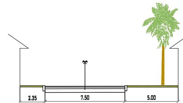
CALLE YAMPARAEZ PROGRESIVA 1+255 MUNICIPIO DE PADCAYA ESC: 1/200
