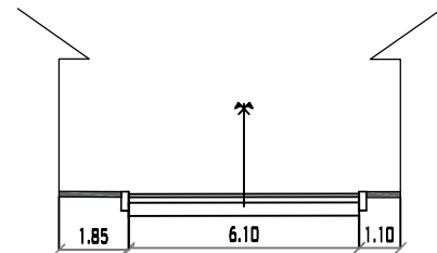
CALLE GILBERTO SAAVEDRA PROGRESIVA 0+920 MUNICIPIO DE PADCAYA ESC: 1/200
