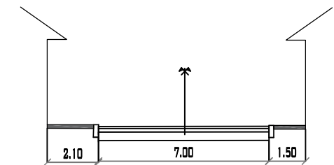
CALLE 1 PROGRESIVA 0+201 MUNICIPIO DE PADCAYA ESC: 1/200
