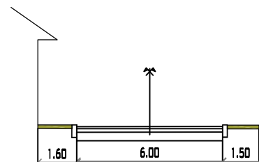
CALLE ANTONIO JOSE DE SUCRE PROGRESIVA 0+055 MUNICIPIO DE PADCAYA ESC: 1/200
