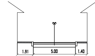
CALLE 10 PROGRESIVA 0+030 MUNICIPIO DE PADCAYA ESC:1/200
