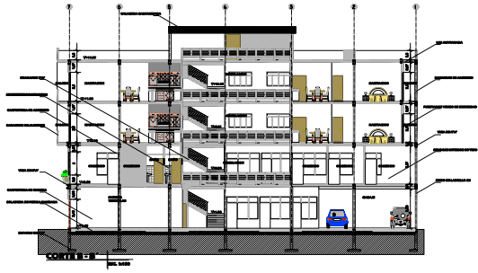
CORTA B-B
