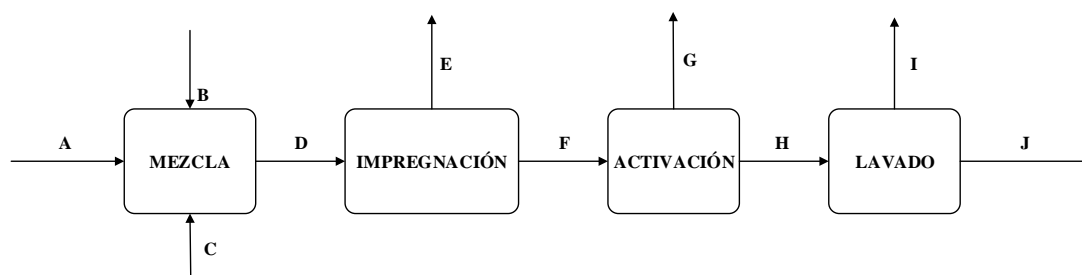
Figura ¡Error! No hay texto con el estilo especificado en el documento.-8: Diagrama de Flujo General de la Activación Química con Cloruro de Calcio.
