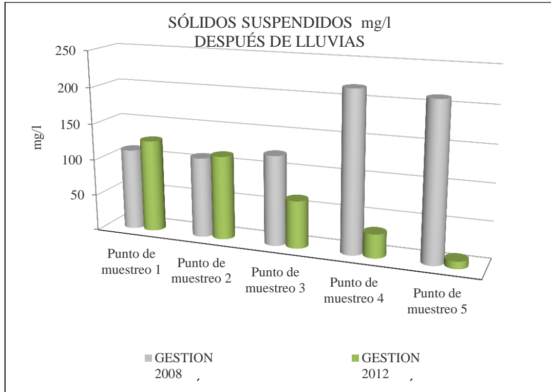
Gráfico 12. Sólidos suspendidos (mg/l) después de lluvias
