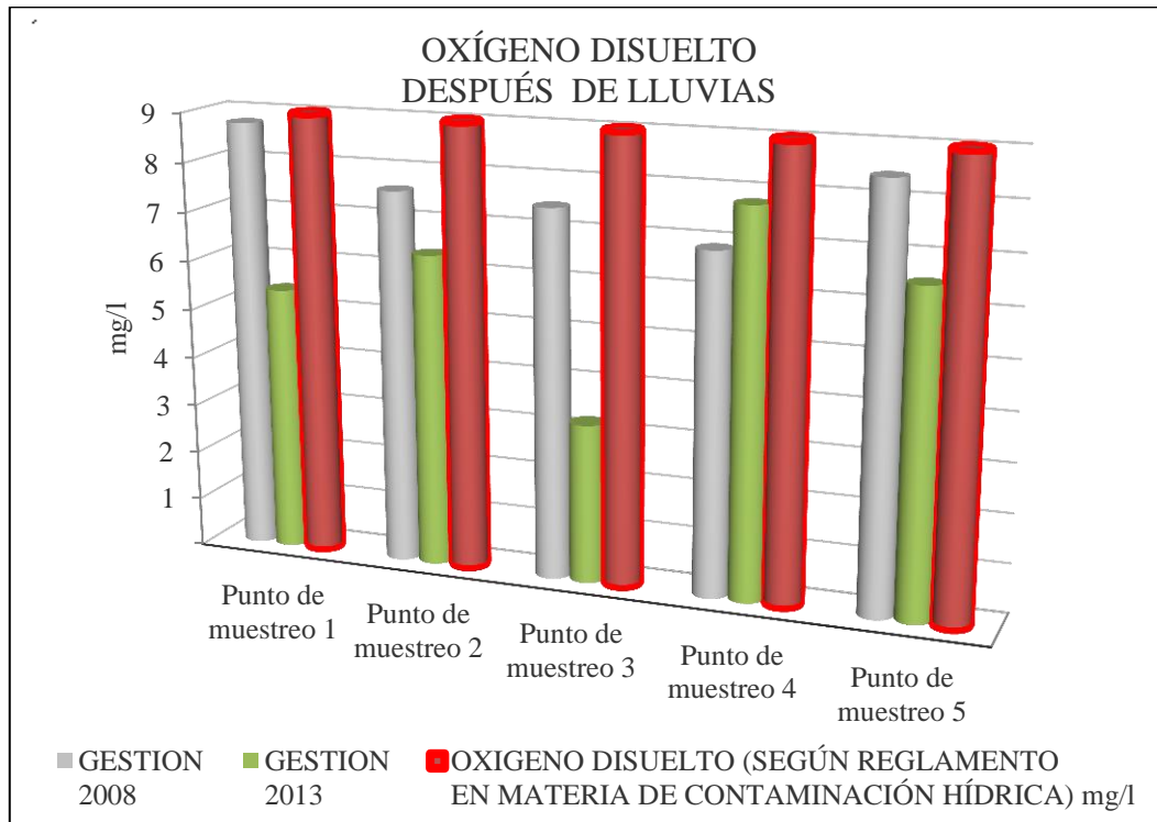
Gráfico 3. Oxígeno disuelto después de lluvias
