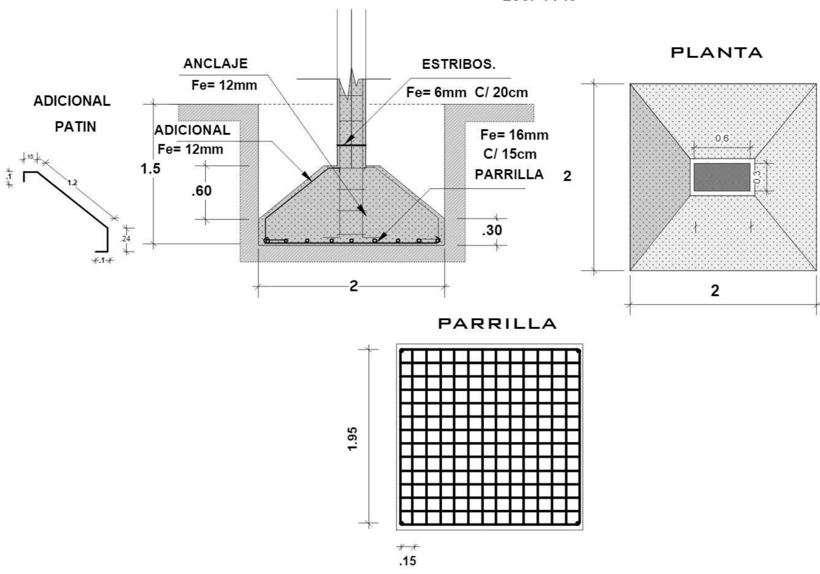
DETALLE ZAPATA ESC. 1:25
