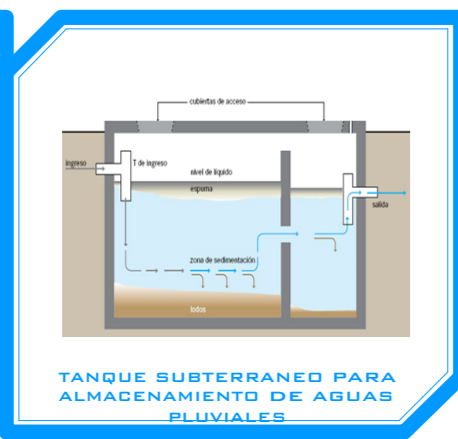
TANQUE SUBTERRANEO PARA ALMACENAMIENTO DE AGUAS PLUVIALES
