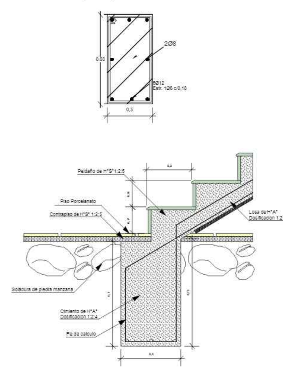
Encadenado de Fundación 0,60x0,30 ESC. 1:15
