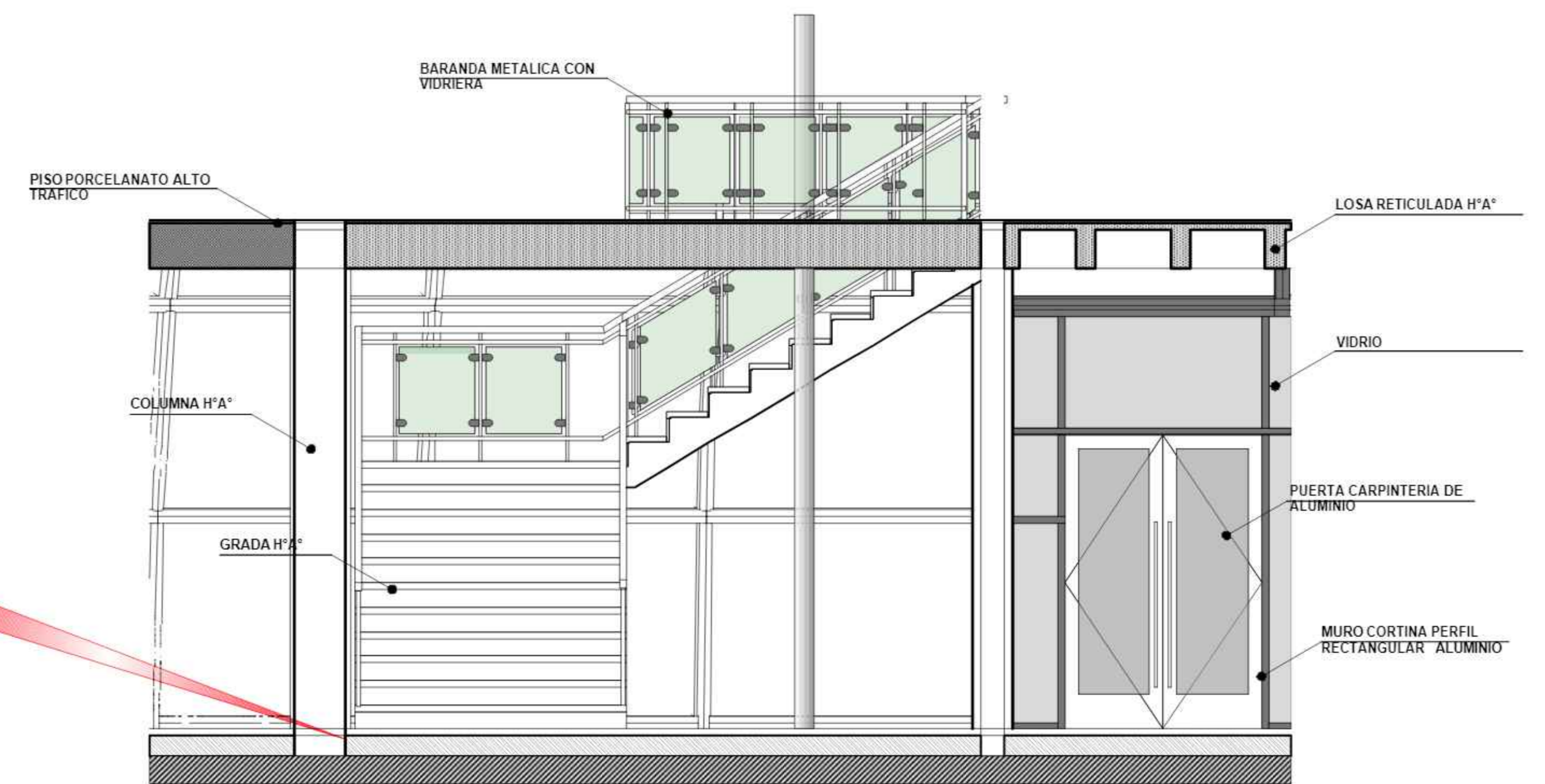
DETALLE DE GRADA ESC. 1:30
