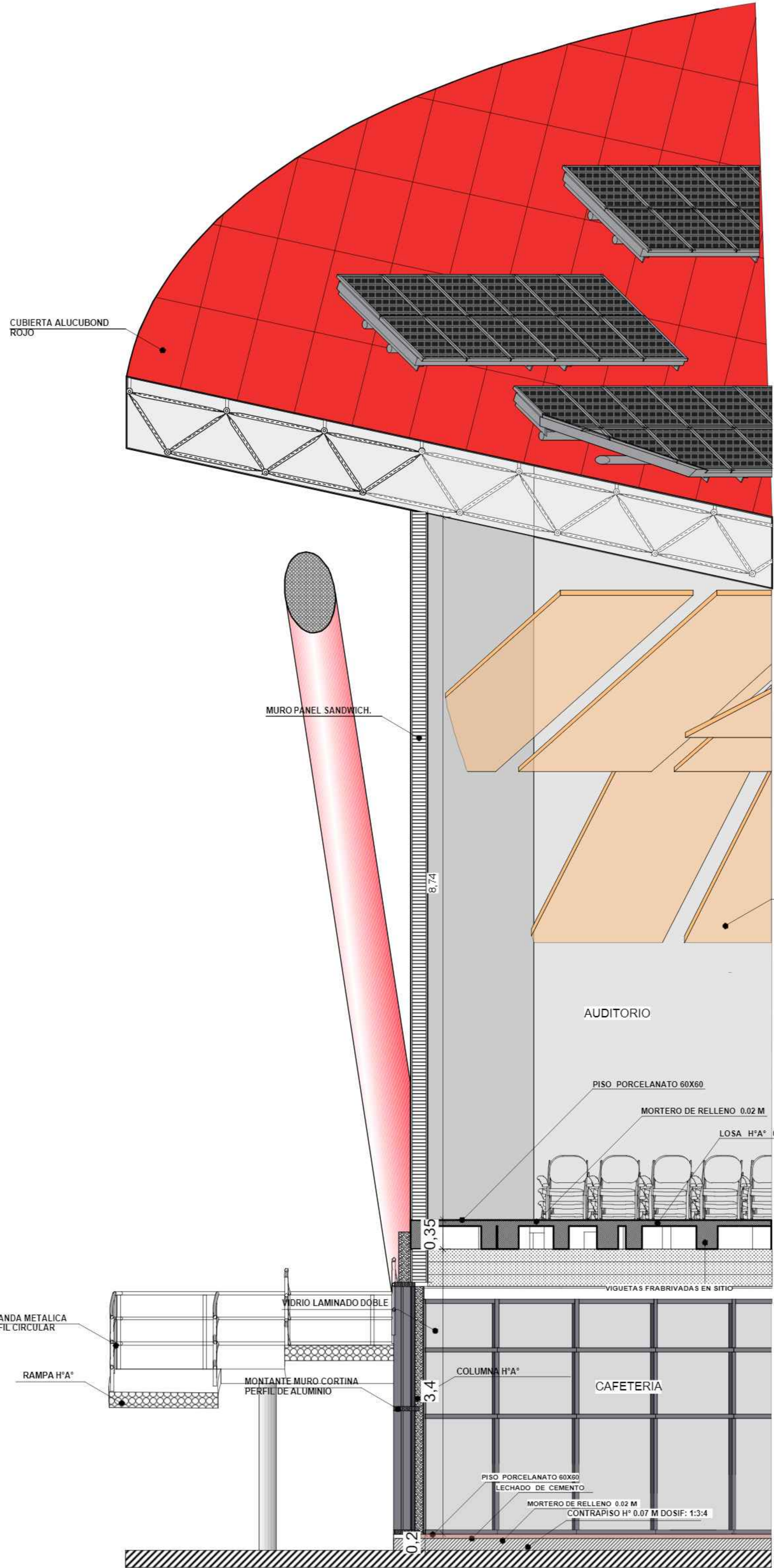
CORTE DE BORDE ESC. 1:30
