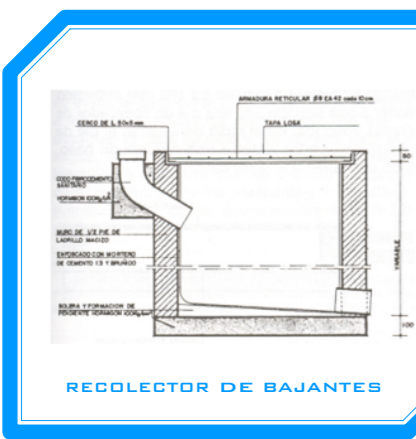
RECOLECTOR DE BAJANTES
