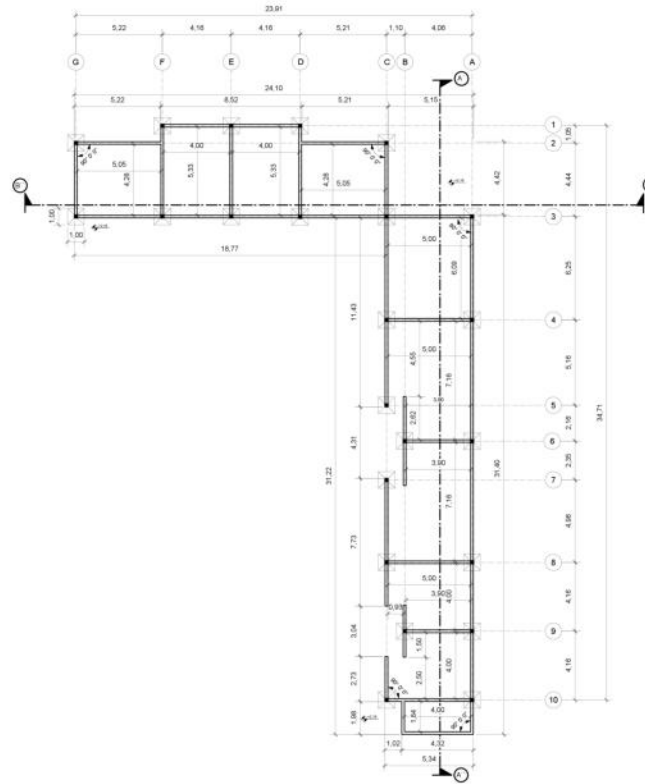
● CIMENTOS - BLOQUE DE RELAJACIÓN ESC. 1:100
