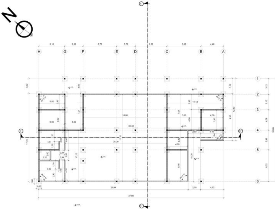
● CIMENTOS - BLOQUE DE GASTRONOMÍA ESC. 1:100
