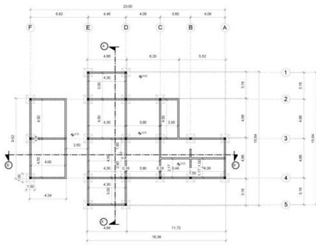
● CIMENTOS - BLOQUE DE SERVICIOS ESC. 1:100
