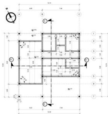
● CIMENTOS - CABAÑA FAMILIAR ESC. 1:100
