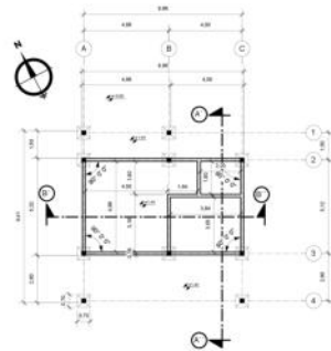
● CIMENTOS - CABAÑA SIMPLE ESC. 1:100
