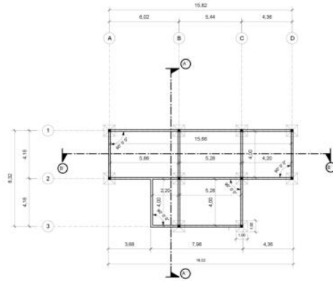
● CIMENTOS - BLOQUE DE DESINFECCIÓN ESC. 1:100
