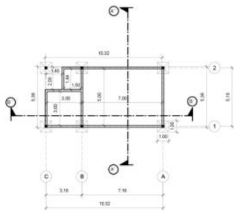
● CIMENTOS - BLOQUE DE TALLERES ESC. 1:100
