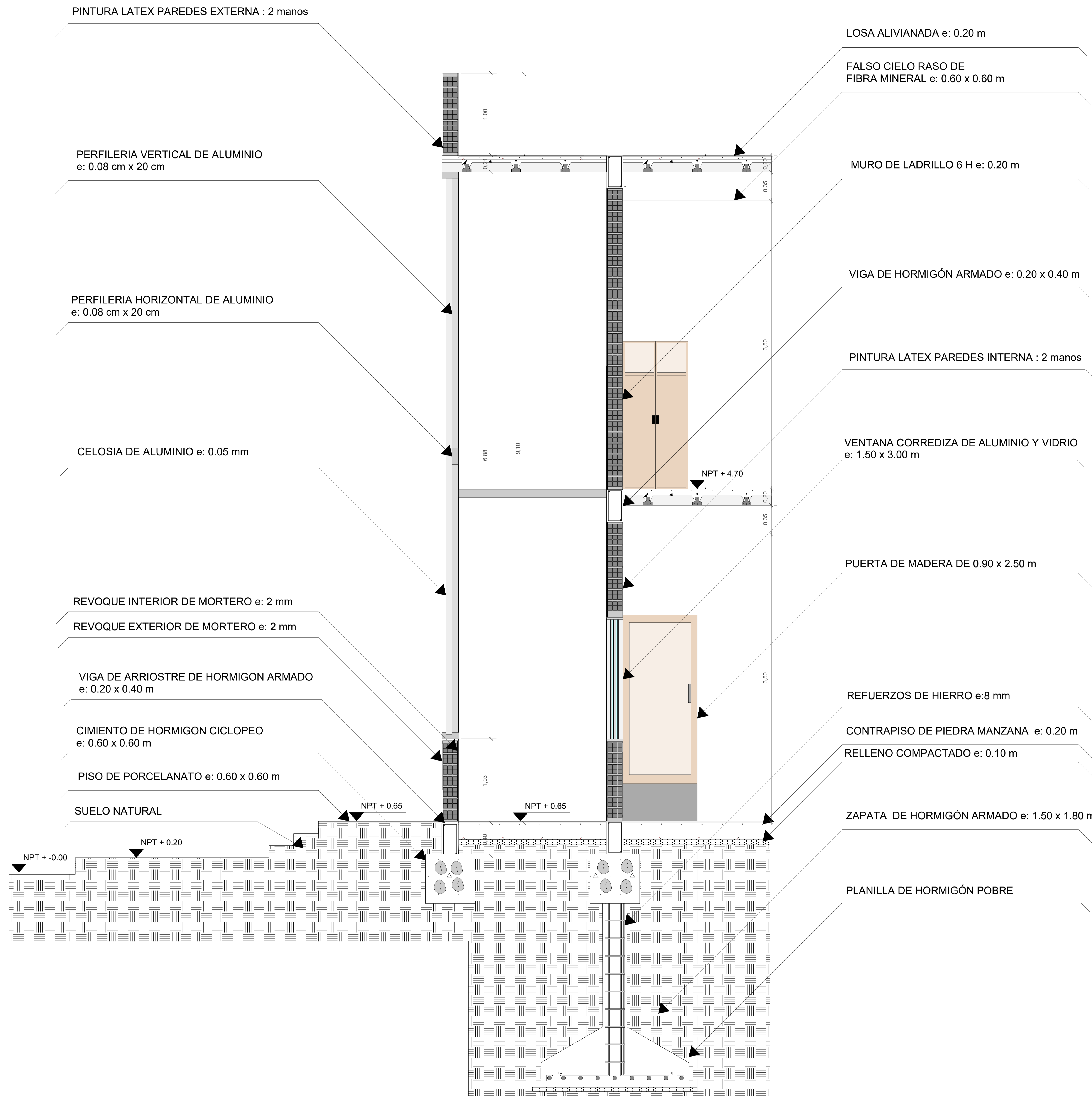
CORTE DE BORDE ESCALA:1:20
