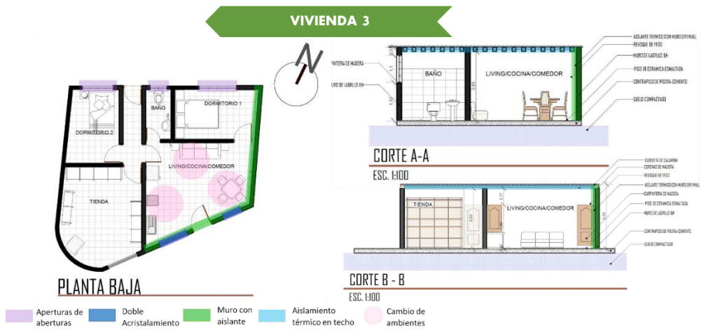
Imagen 29 Planos arquitectónicos de las viviendas 3 (Intervenido)
