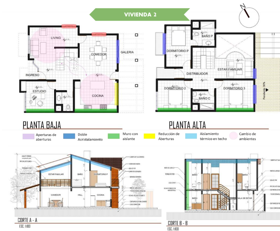
Imagen 28 Planos arquitectónicos de la vivienda 2 (Intervenido)
