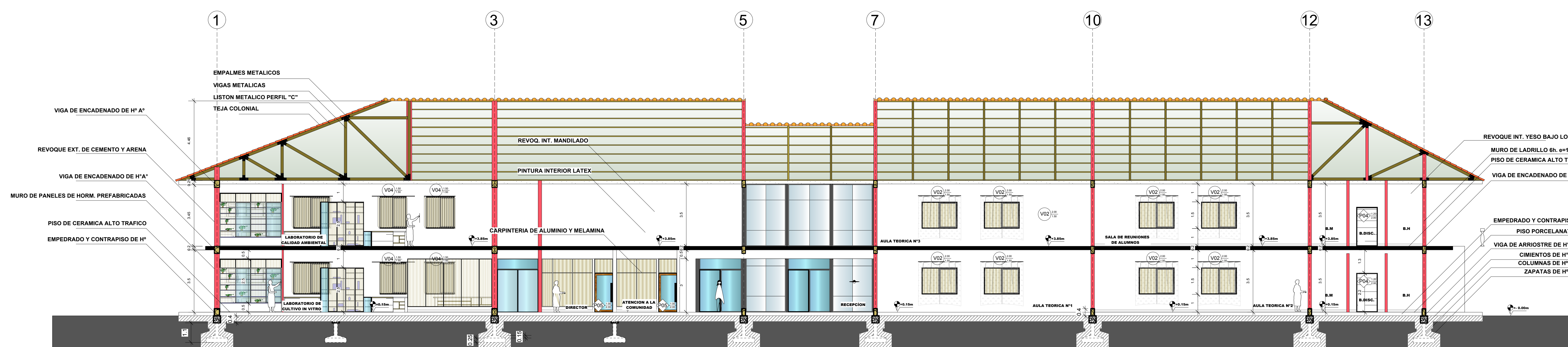
.....CORTE A1 - A1.....
