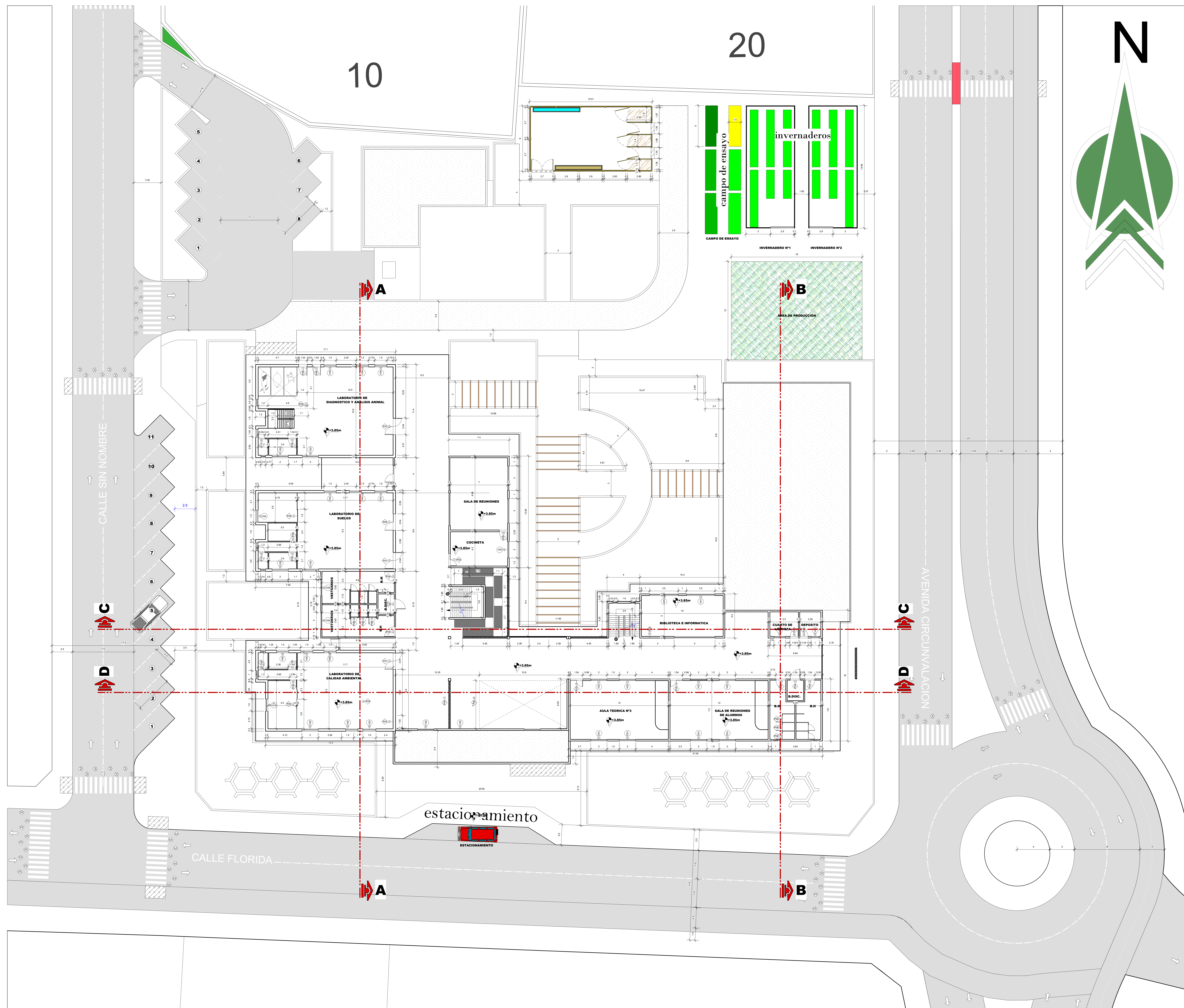
.....PLANTA ALTA ACOTADA..... Esc. 1:100
