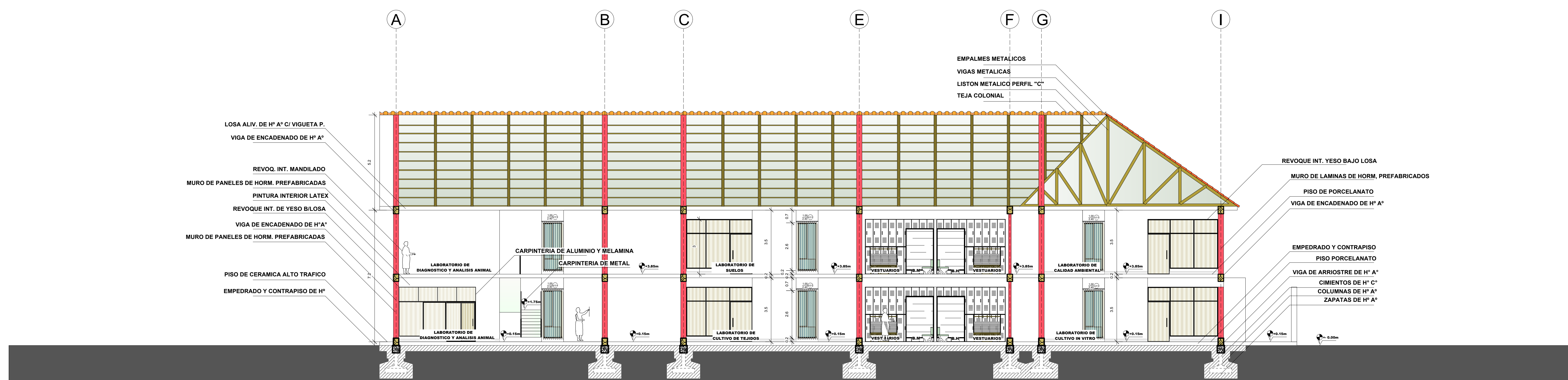
.....CORTE B1 - B1.....
