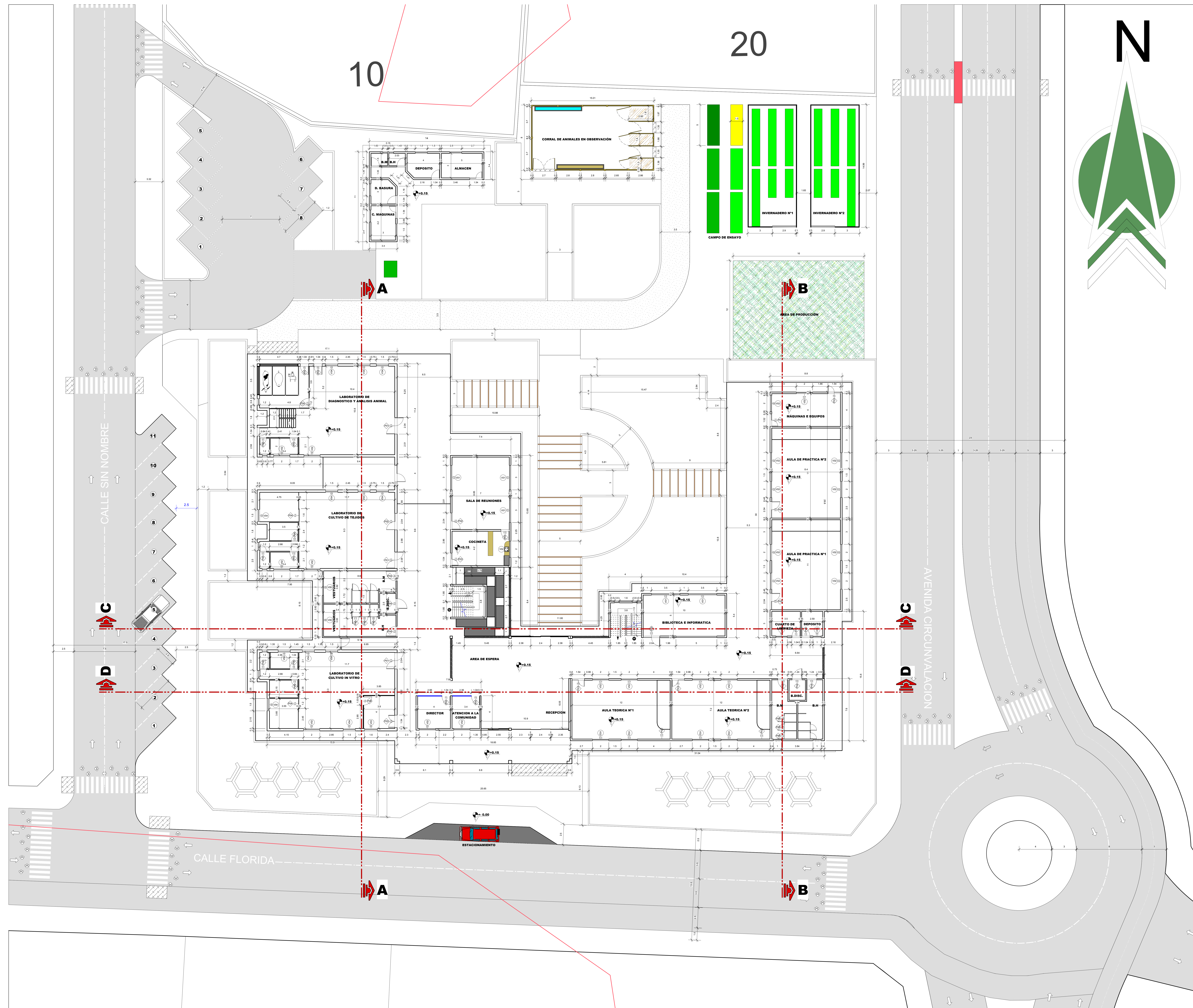
-----PLANTA BAJA ACOTADA,----- Esc. 1:100
