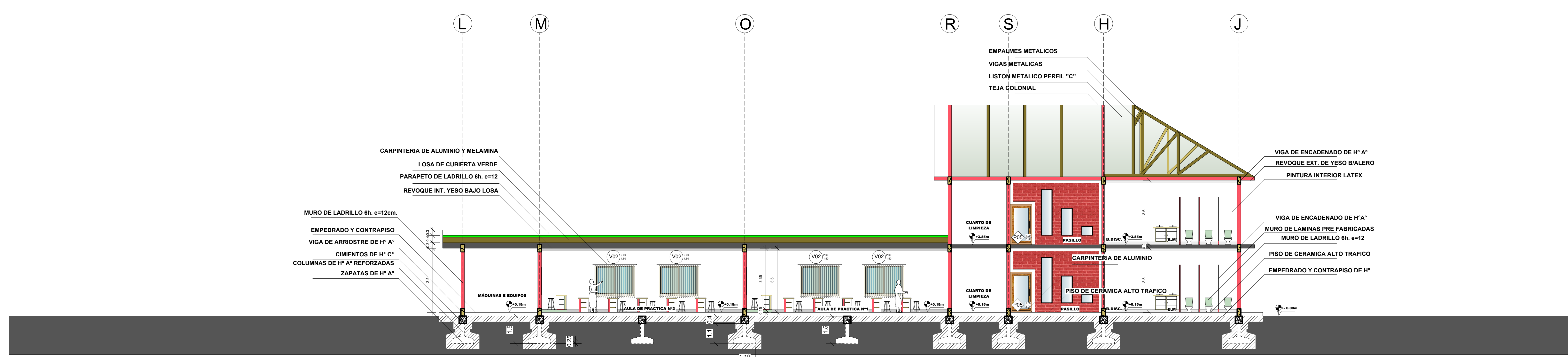
.....CORTE B2 - B2.....
