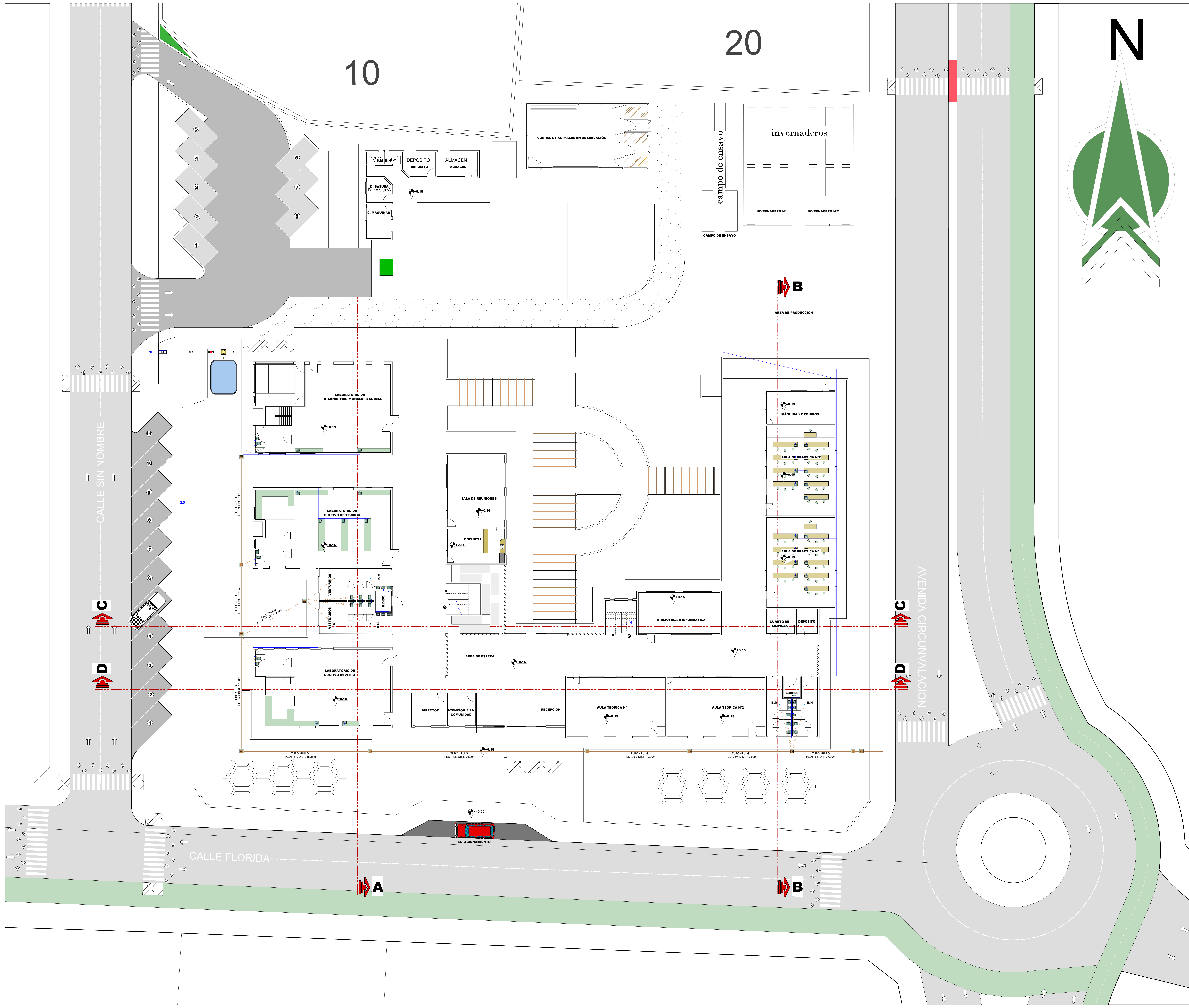
-----..INSTALACIONES SANITARIAS PLANTA BAJA.----- Esc. 1:100
