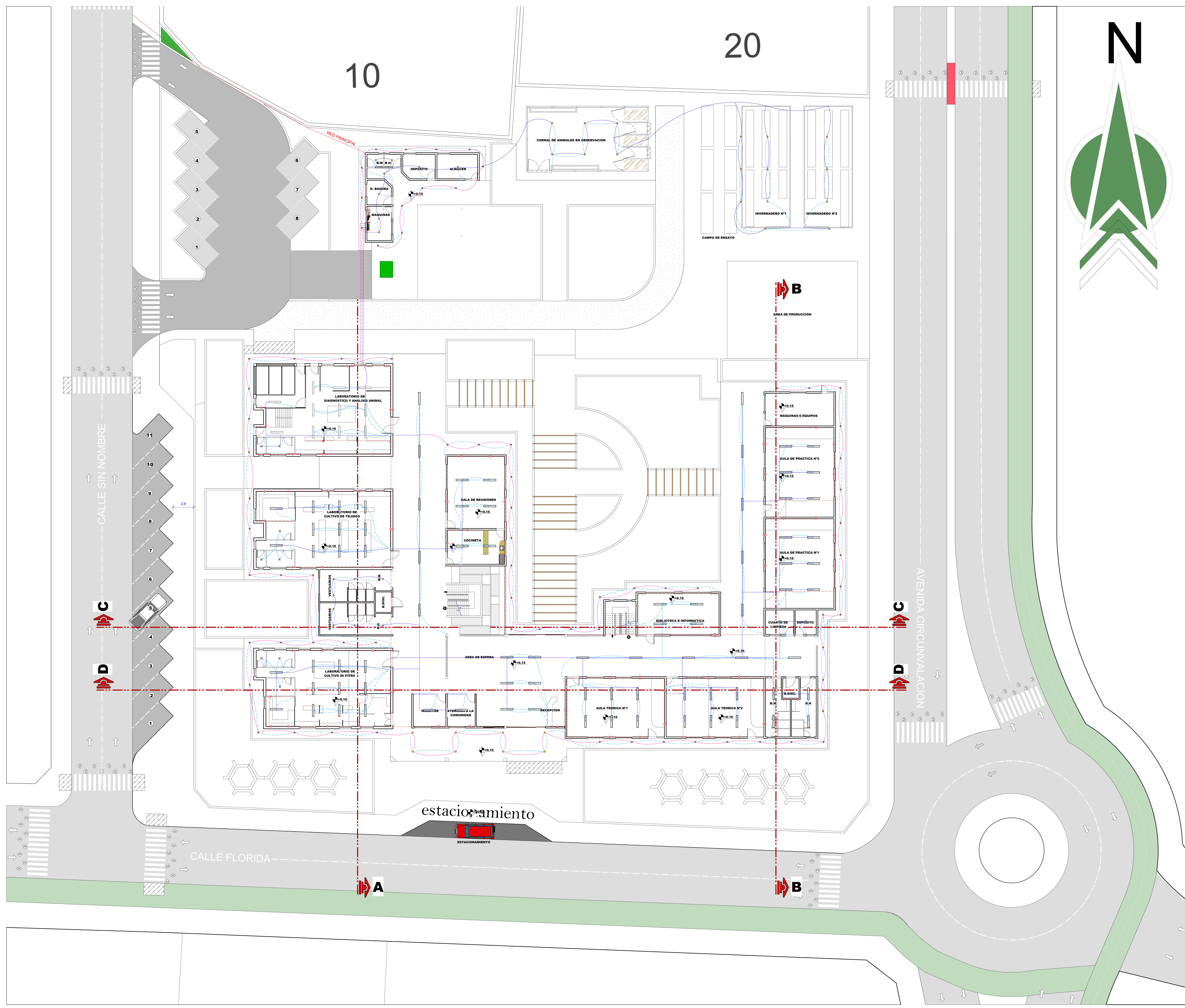
.....INSTALACIONES ELECTRICAS PLANTA BAJA ..... Esc. 1:100
