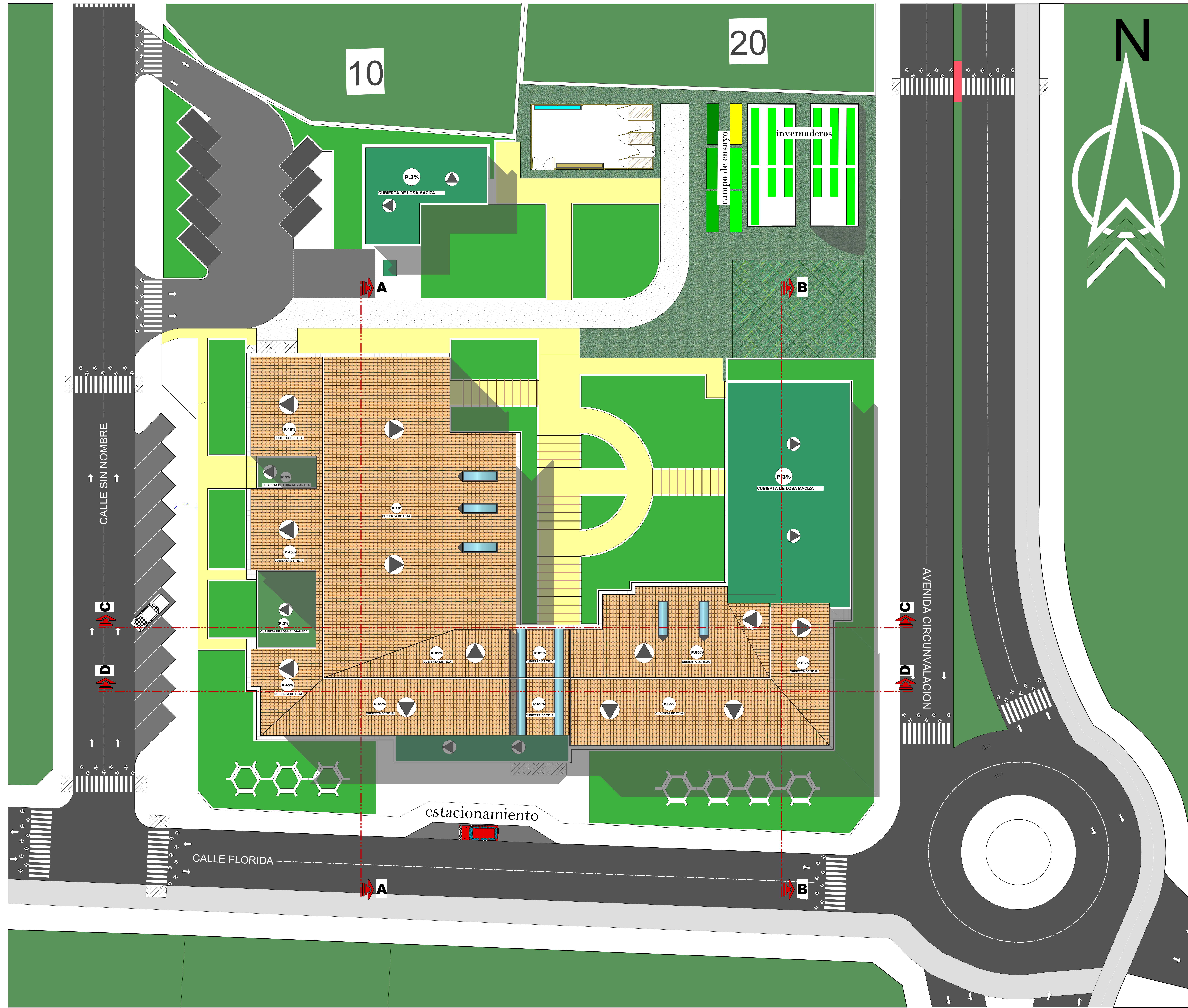
..... PLANO DE SITIO Y TECHOS ..... Esc. 1:100
