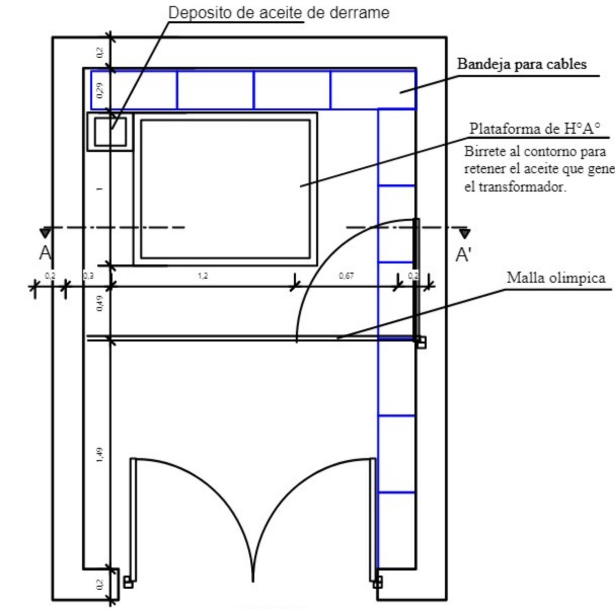
PLANTA Esc. 1:25
