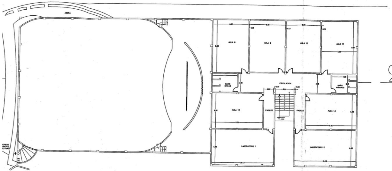
... PLANTA PRIMER PISO ...
