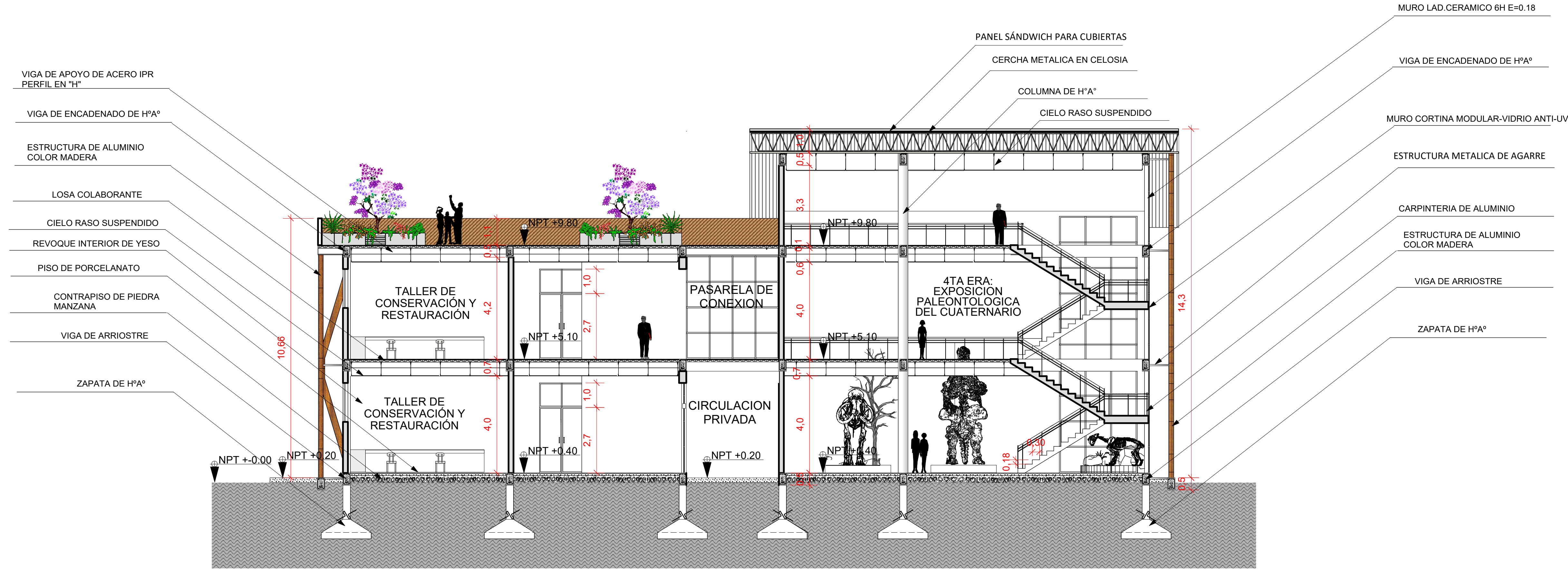
CORTE C - C' ESC. 1:100
