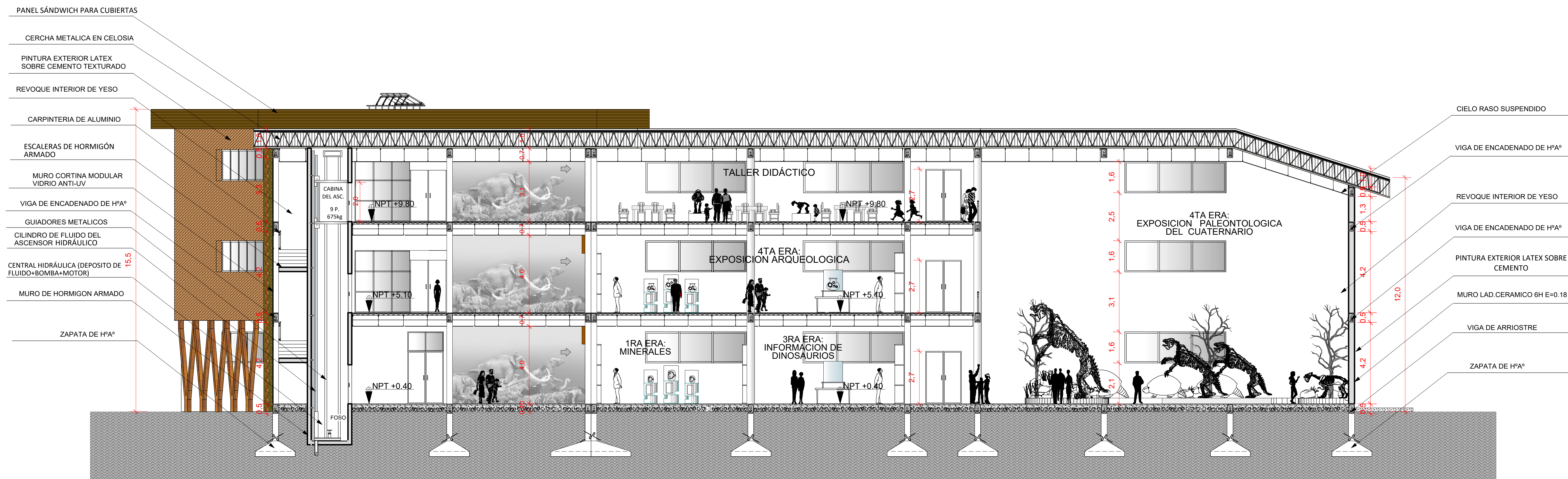
CORTE D - D' ESC. 1:100
