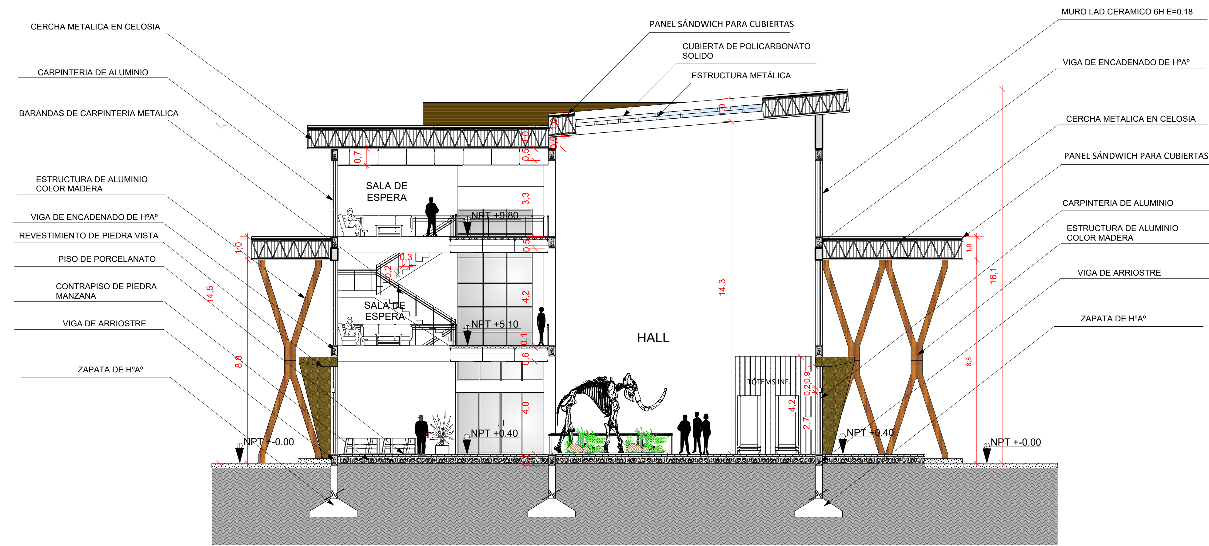
CORTE A - A' ESC. 1:100
