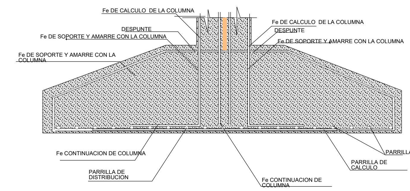
DETALLE DE ZAPATAS EN JUNTA DE DILATACION
