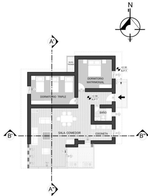
1 PLANO AMOBLADO CABAÑA TIPOLOGIA 3 ESCALA : 1.100
