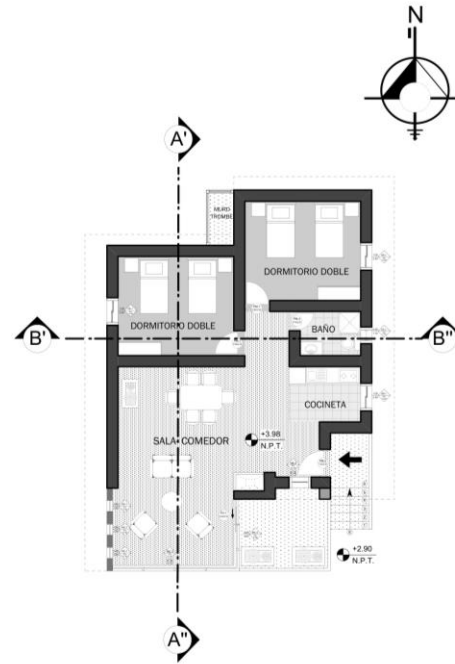
2 PLANO AMOBLADO CABAÑA TIPOLOGIA 2 ESCALA : 1.100
