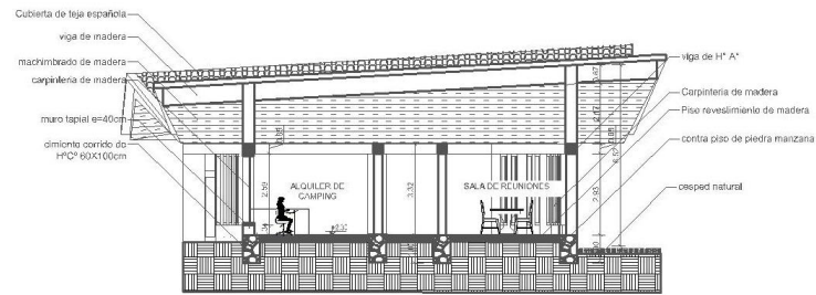
CORTE TRANSVERSAL BLOQUE A ESC. 1:100
