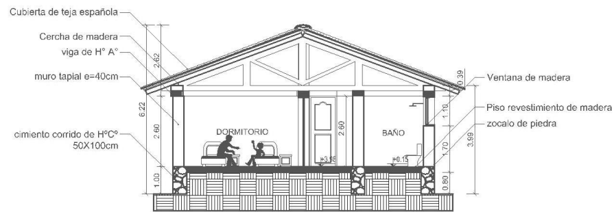
CABAÑA T2 CORTE B-B ESC. 1:100
