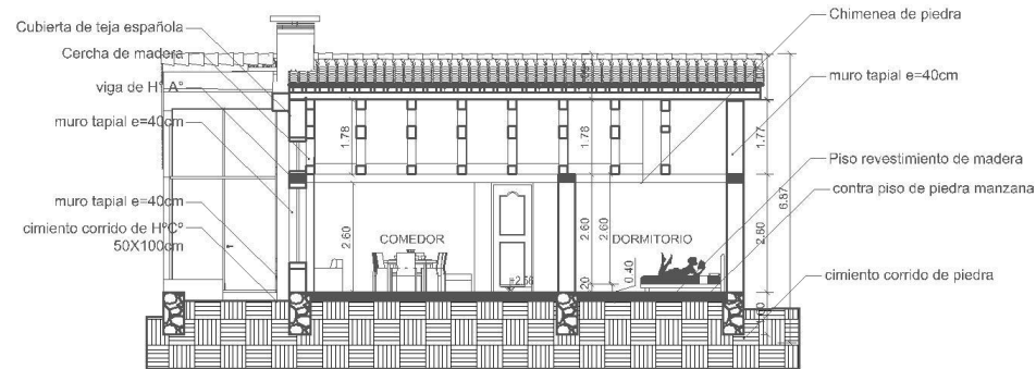
CABAÑA T3 CORTE A-A ESC. 1:100
