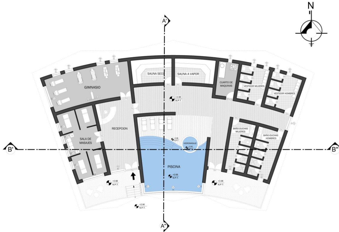
4 PLANO AMOBLADO BLOQUE B ESCALA : 1.100
