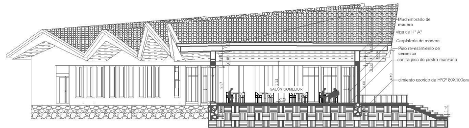
CORTE TRANSVERSAL BLOQUE A ESC. 1:100
