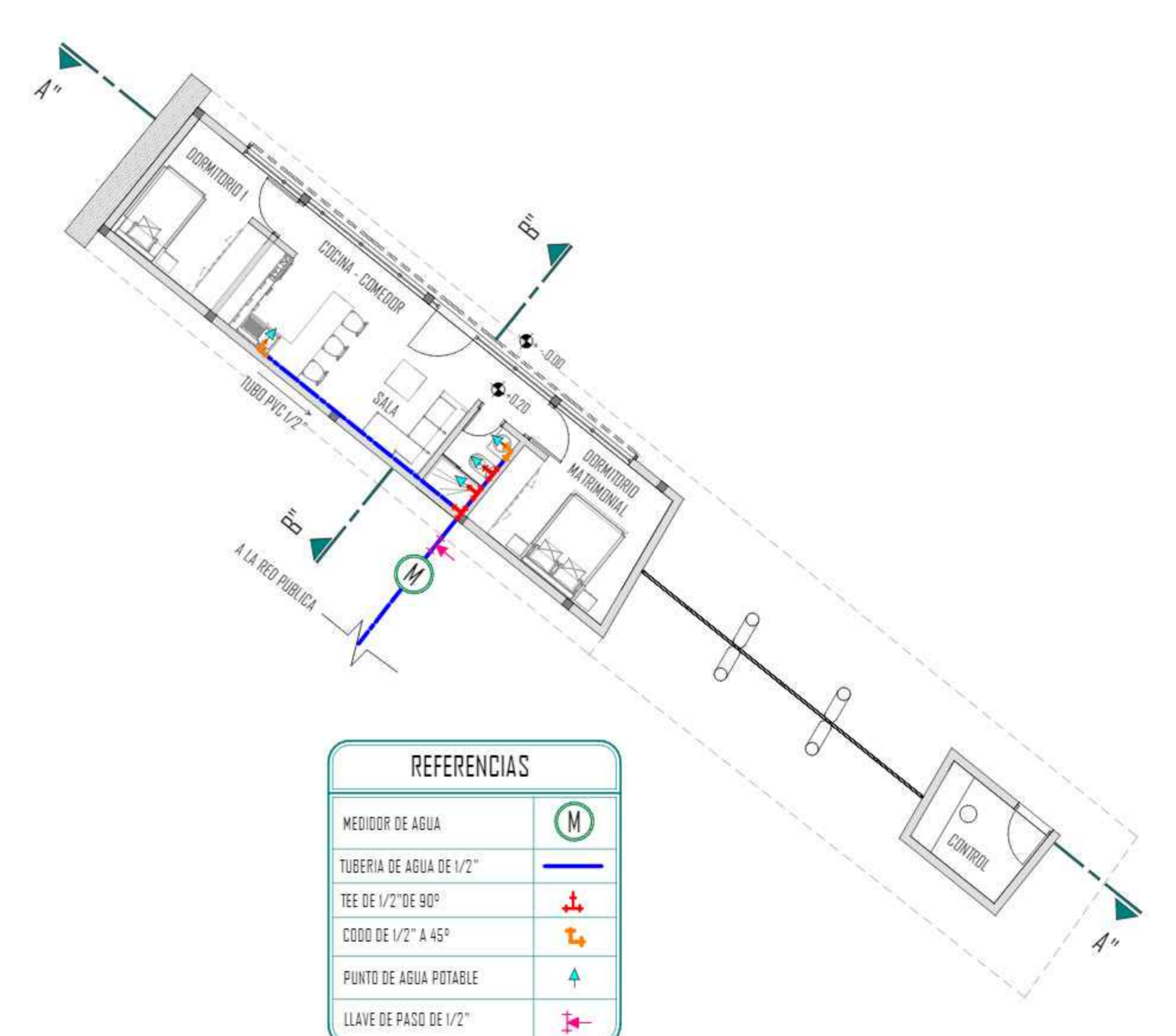
INSTALACION DE AGUA POTABLE VIVIENDA SERENO ESC. 1:100
