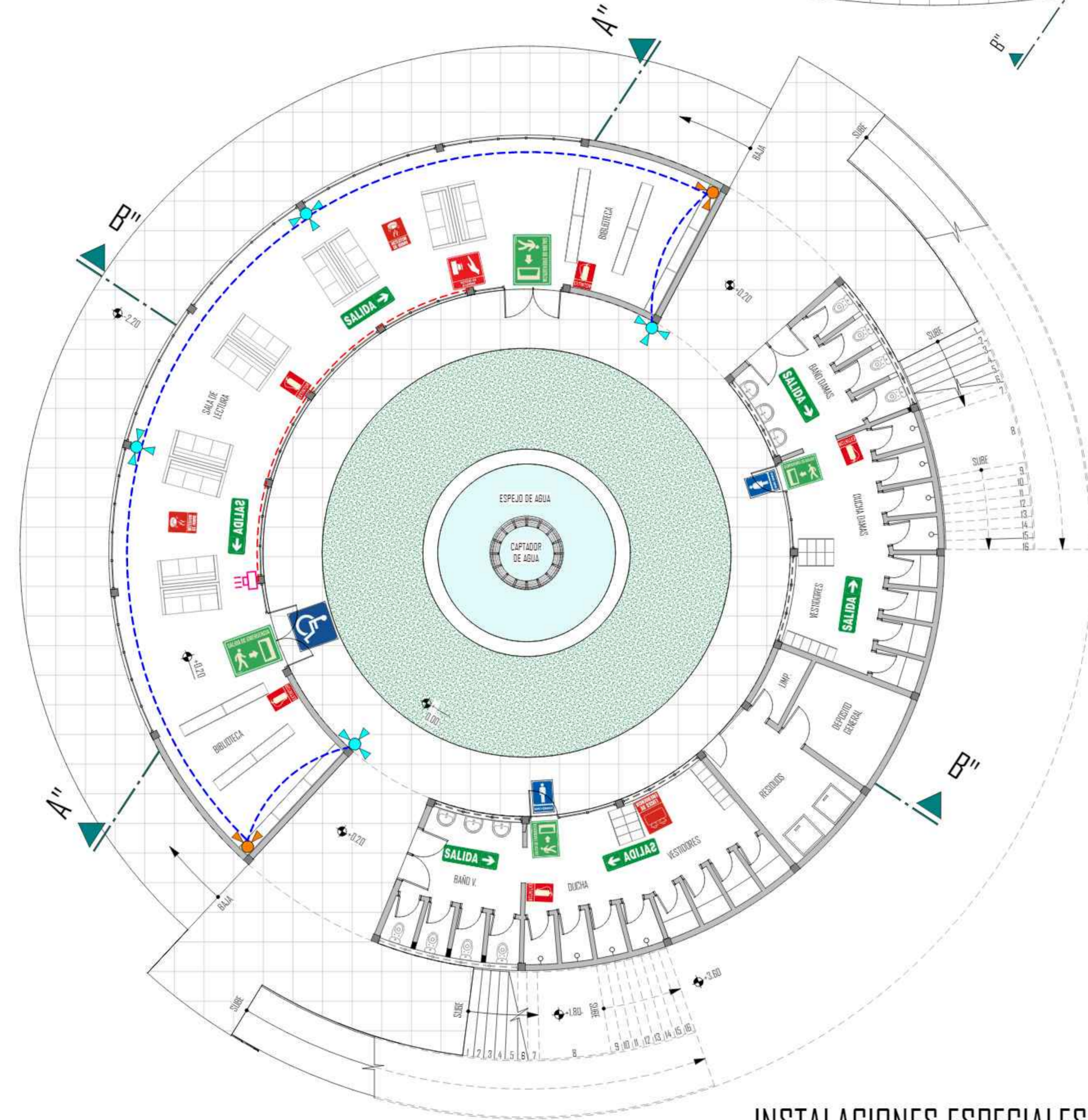
INSTALACIONES ESPECIALES SALA DE LECTURA - BAÑOS ESC. 1:100
