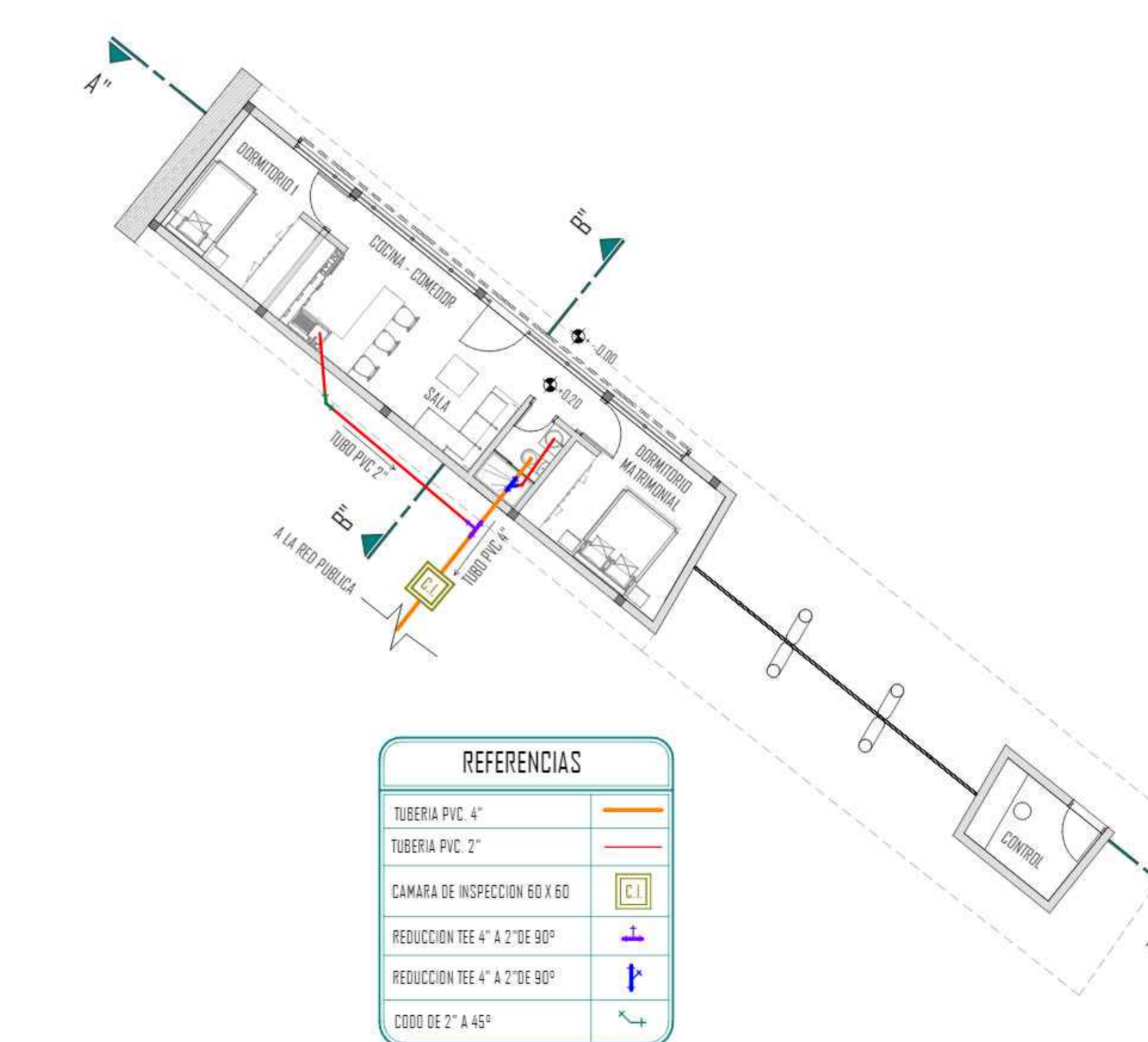
INSTALACION SANITARIA VIVIENDA DEL SERENO ESC. 1:100
