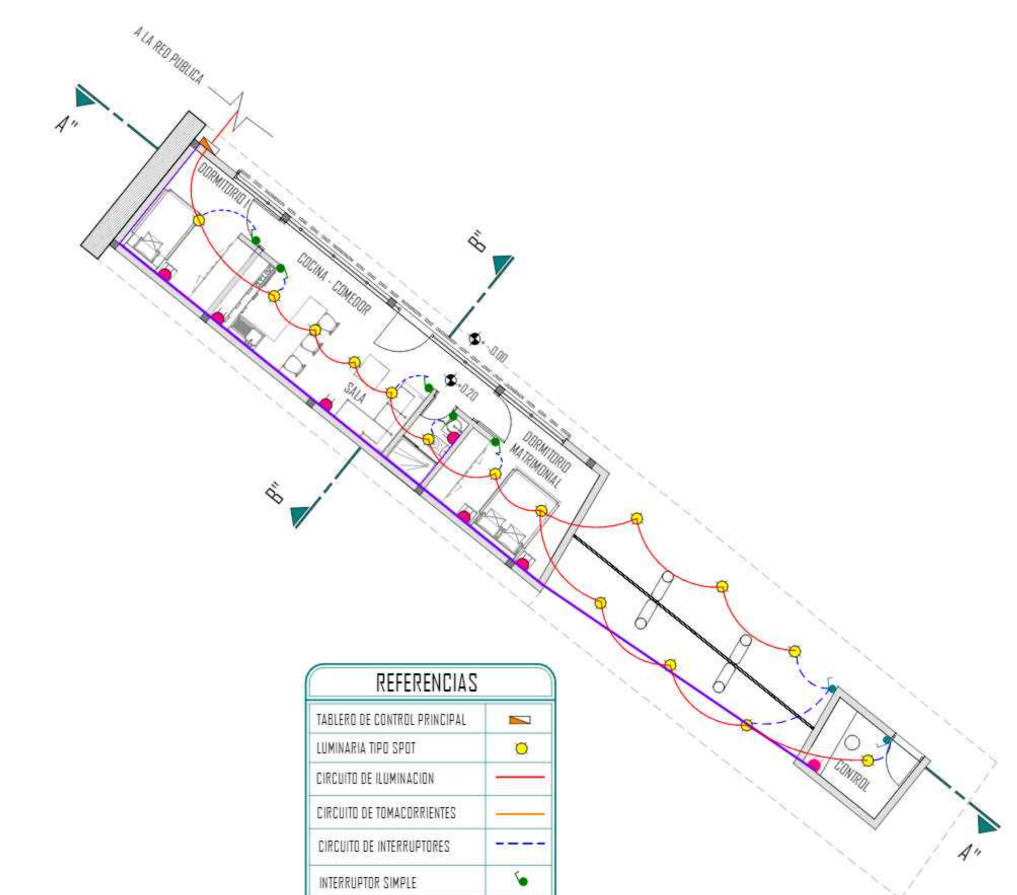
INSTALACION ELECTRICA VIVIENDA SERENO ESC. 1:100
