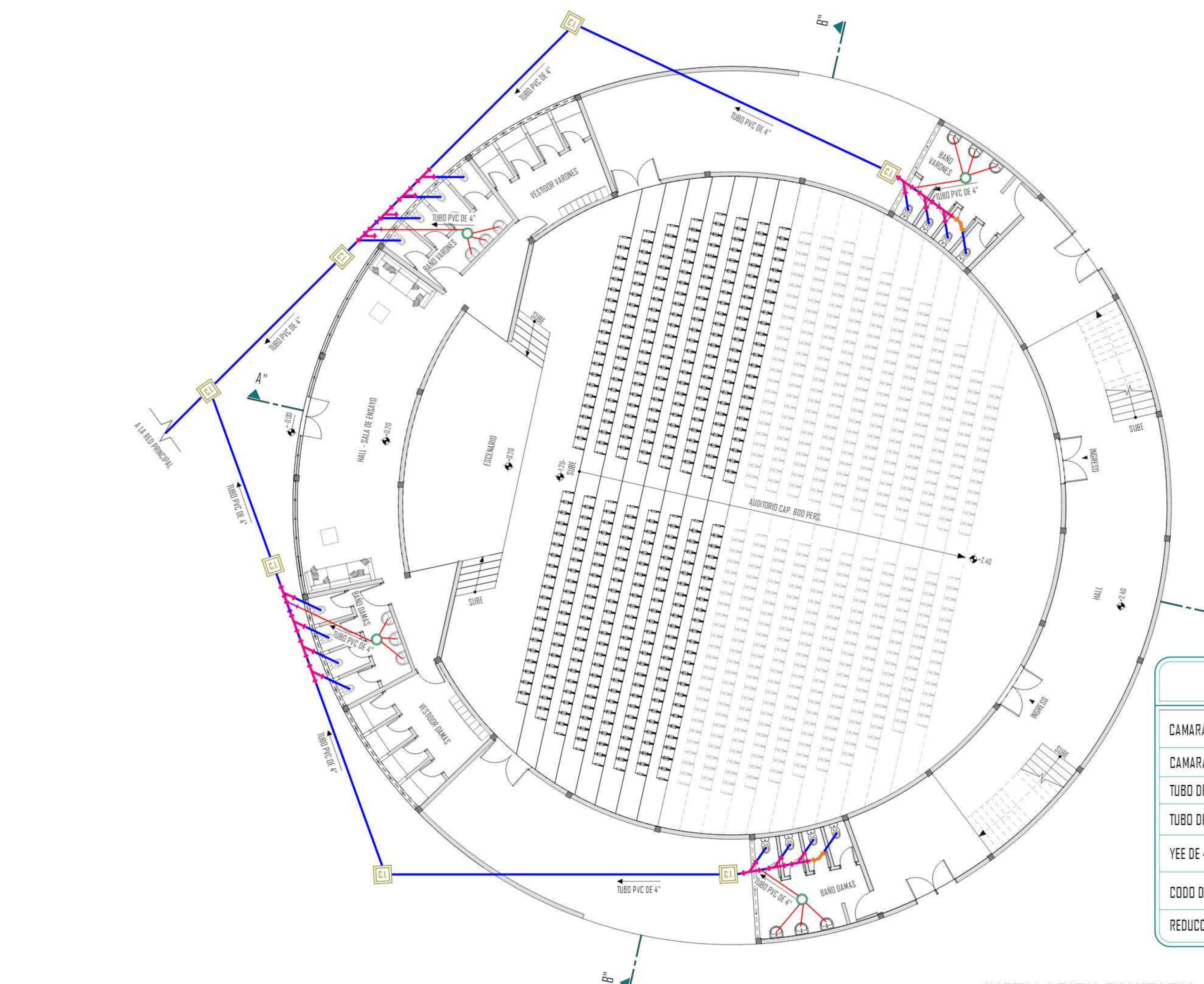
INSTALACION SANITARIA AUDITORIO ESC. 1:100
