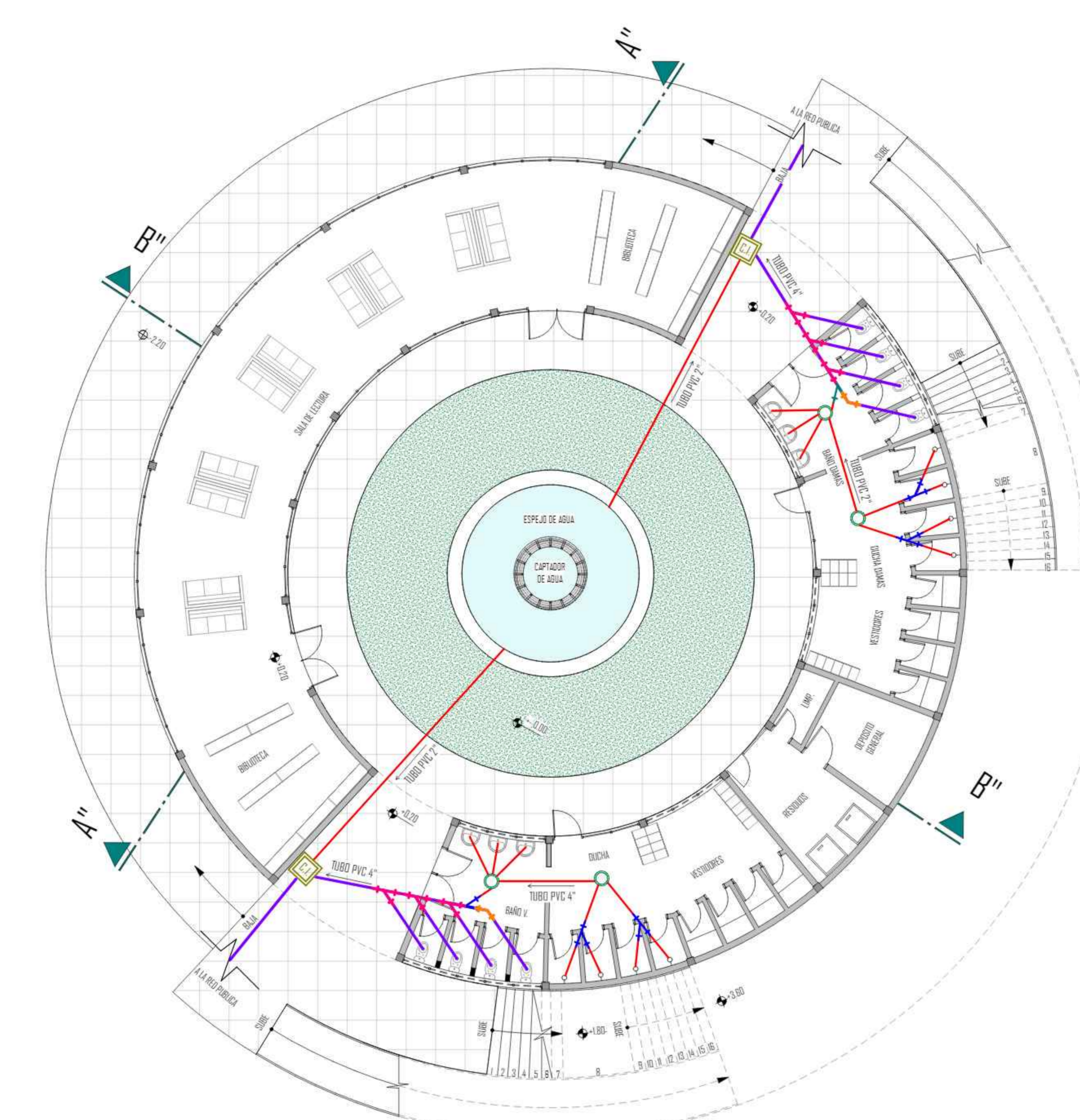
INSTALACION SANITARIA SALA DE LECTURA - BAÑOS ESC. 1:100
