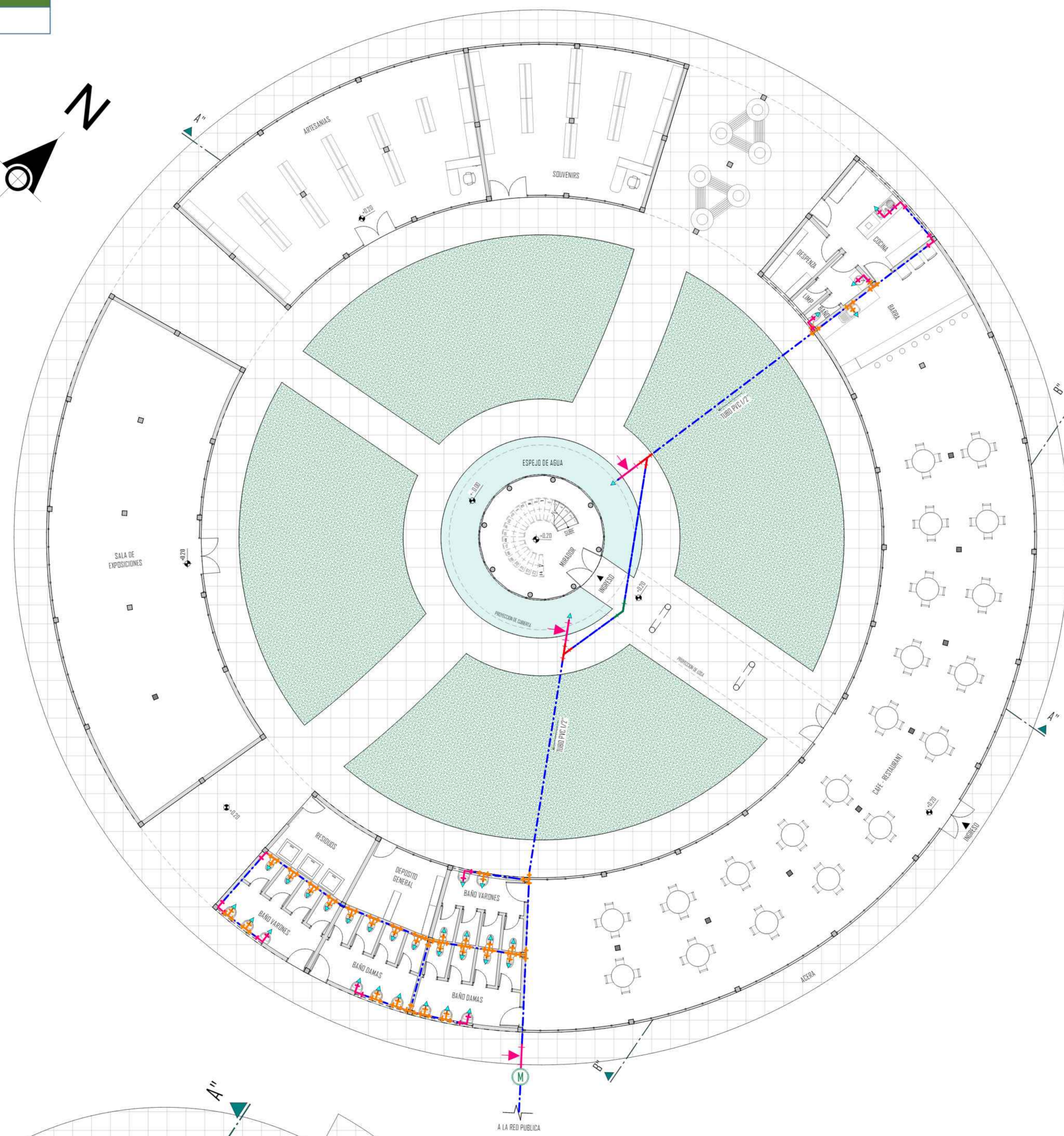
INSTALACION DE AGUA POTABLE CAFETERIA - MIRADOR ESC. 1:100
