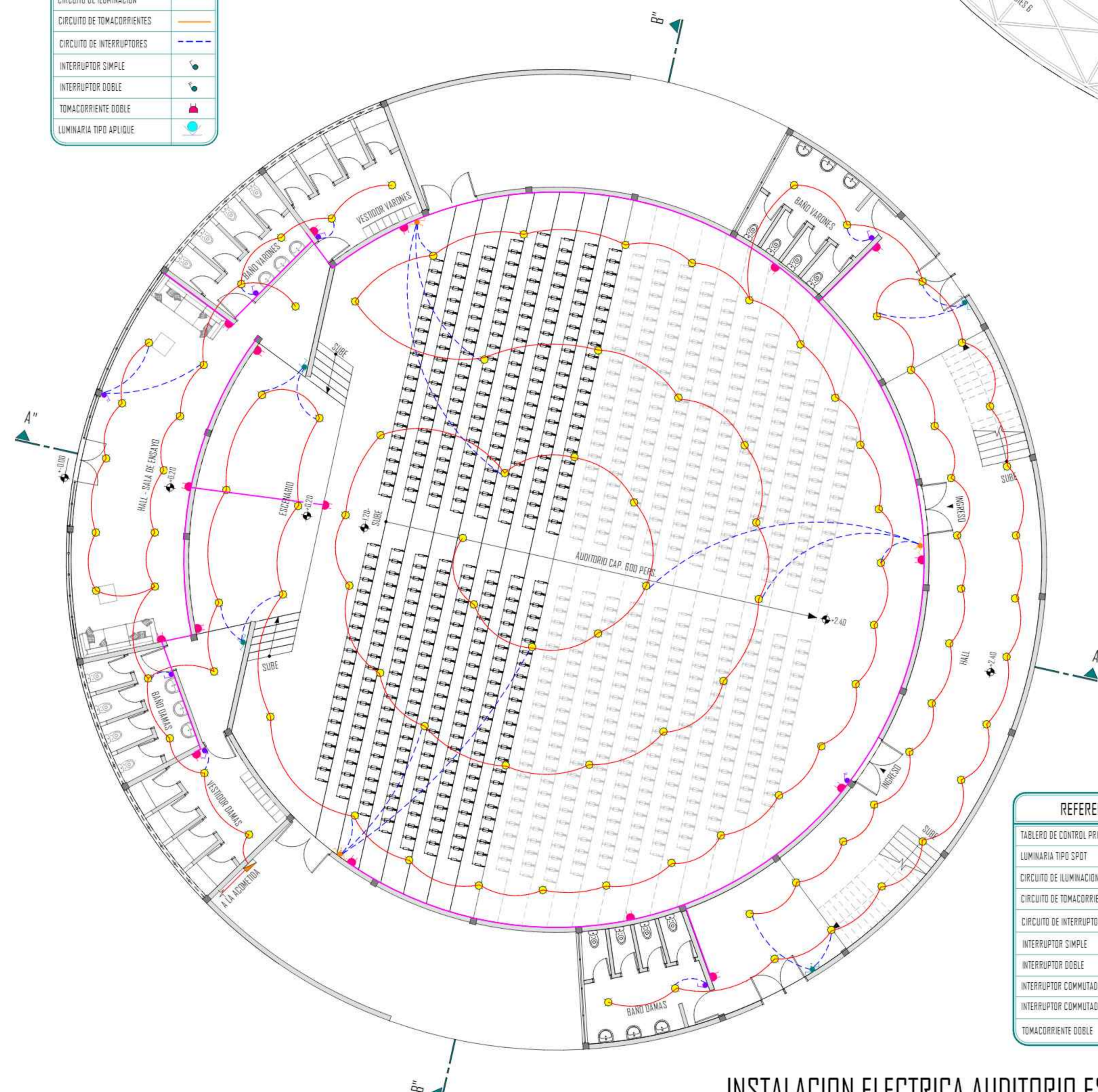
INSTALACION ELECTRICA AUDITORIO ESC. 1:100
