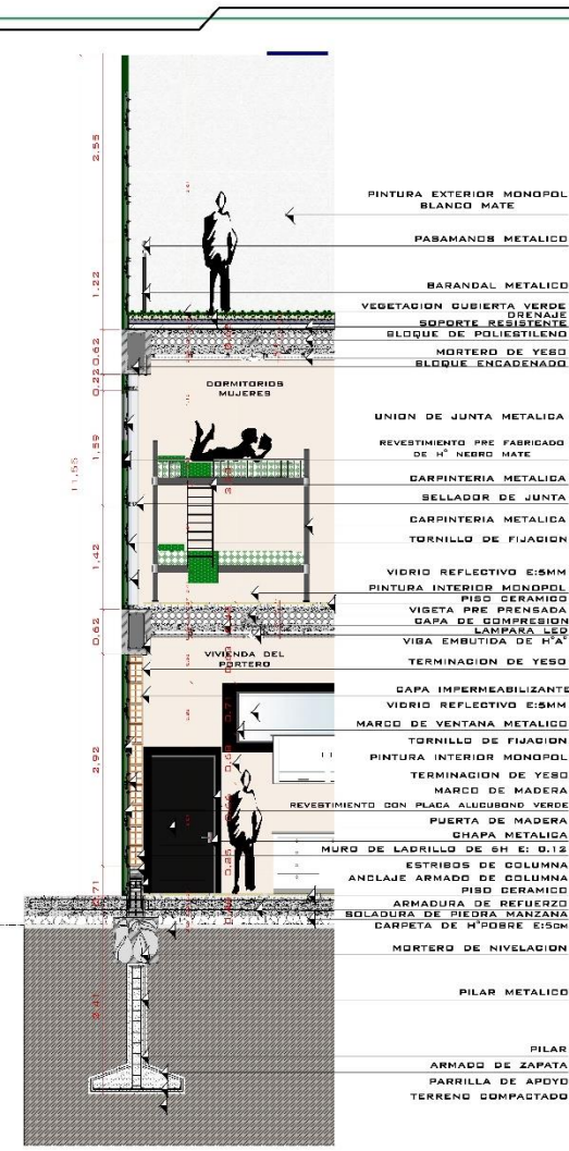
CORTE DE BORDE ESC. 1:15
