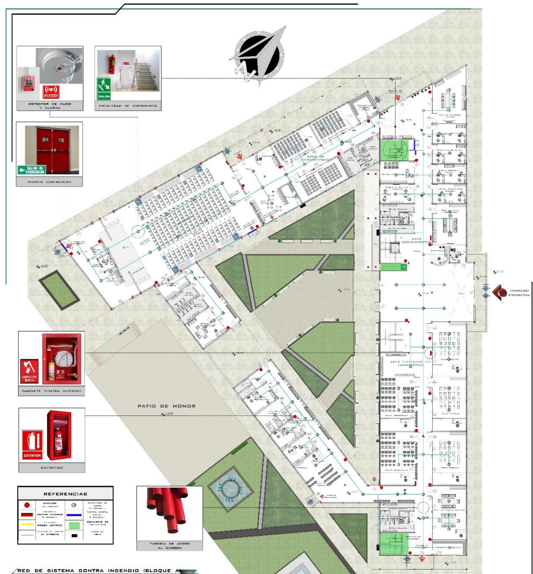
RED DE SISTEMA CONTRA INCENDIO (BLOQUE A) ESCALA 1:100
