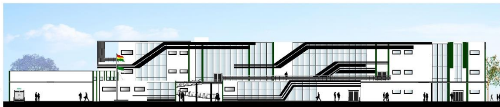
FACHADA POSTERIOR BLOQUE A
