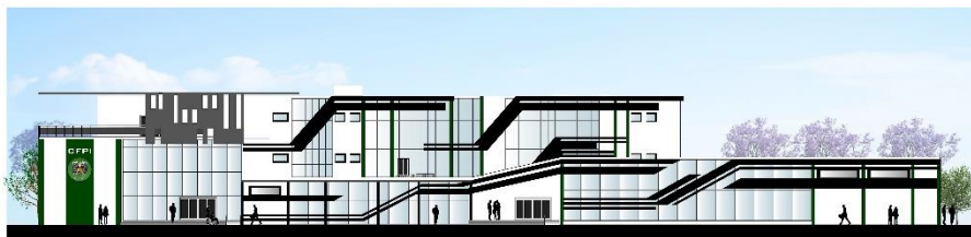
FACHADA LATERAL DERECHO BLOQUE A
