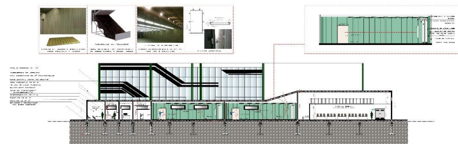
CORTE LONGITUDINAL F-F
