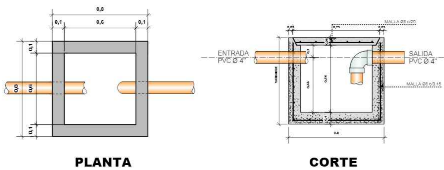
CAMARA DESGRASADORA ESCALA 1:15
