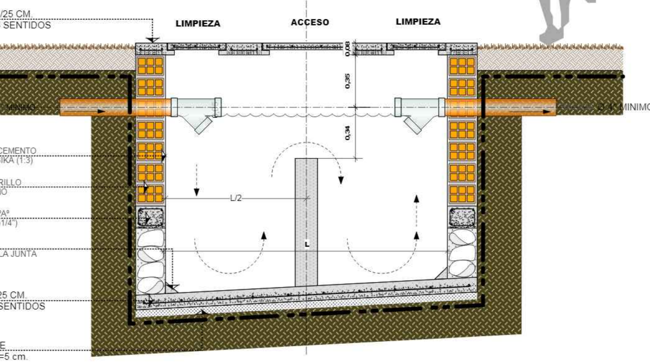
CORTE DE CAMARAS SEPTICAS ESCALA: 1:15
