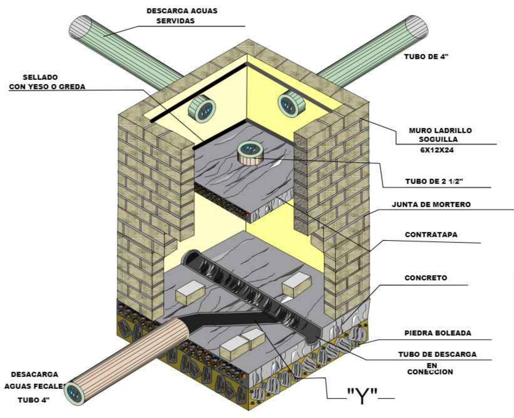
DETALLE CONSTRUCTIVO : CAMARAS DE INSPECCION ESCALA 1:35
