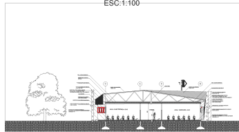
CORTE "G" - "G" ESC:1:100
