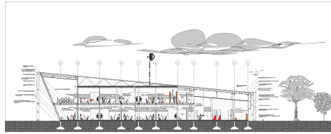
CORTE "C" - "C" ESC:1:100
