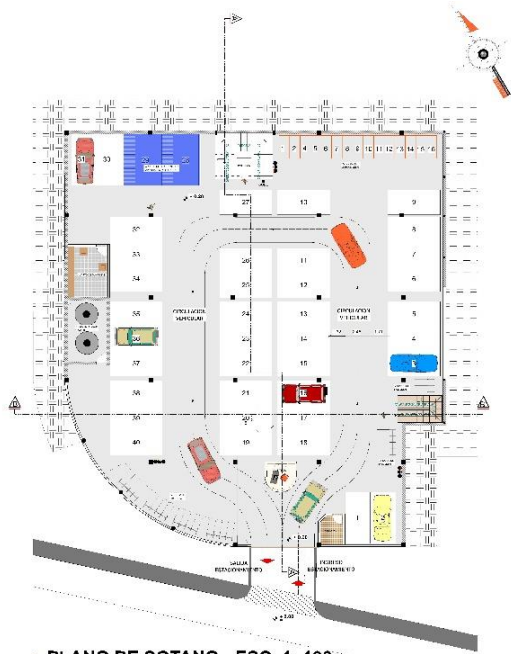
PLANO DE SOTANO ESC. 1: 100
