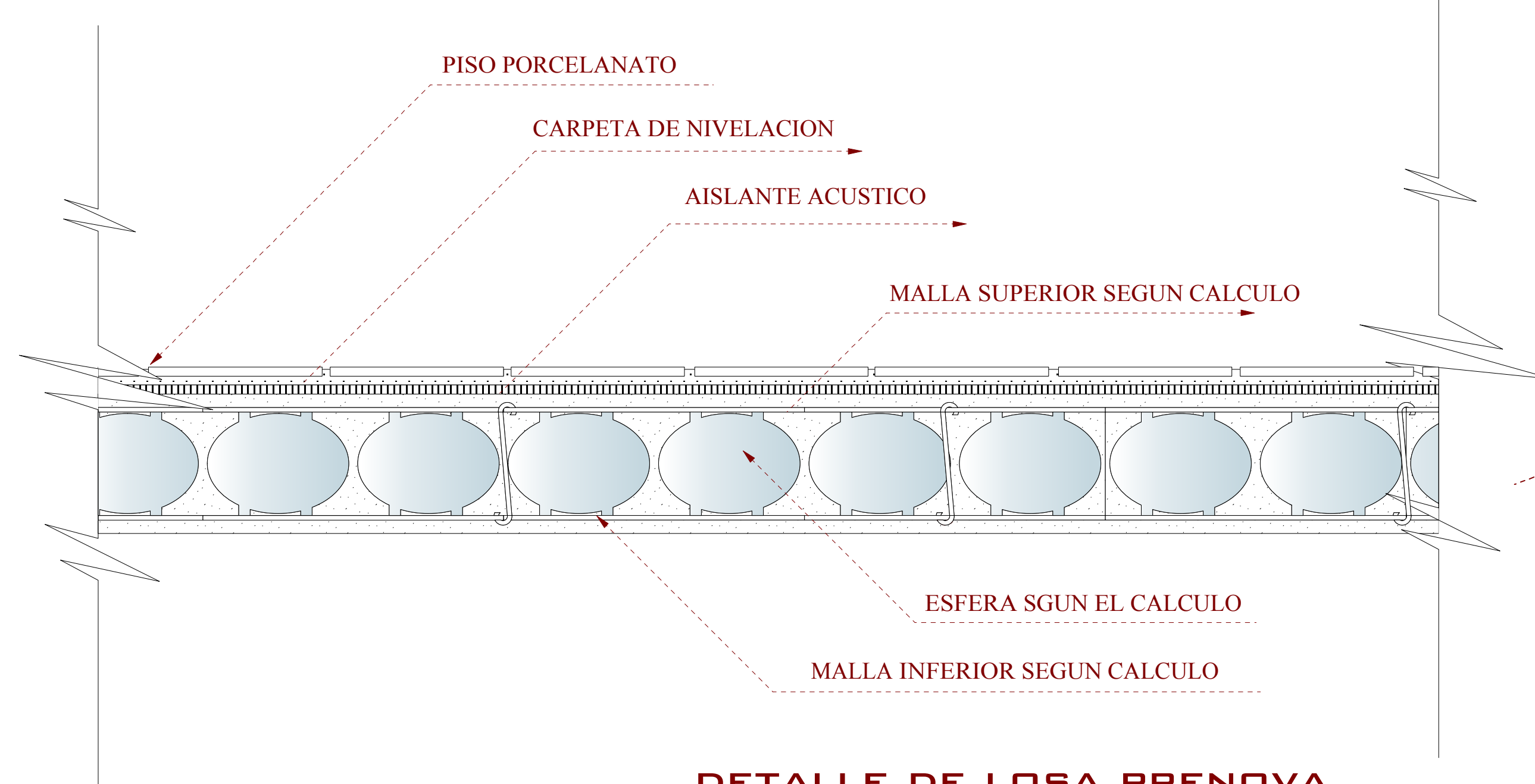
DETALLE DE LOSA PRENOVA ESCALA: 1:10
