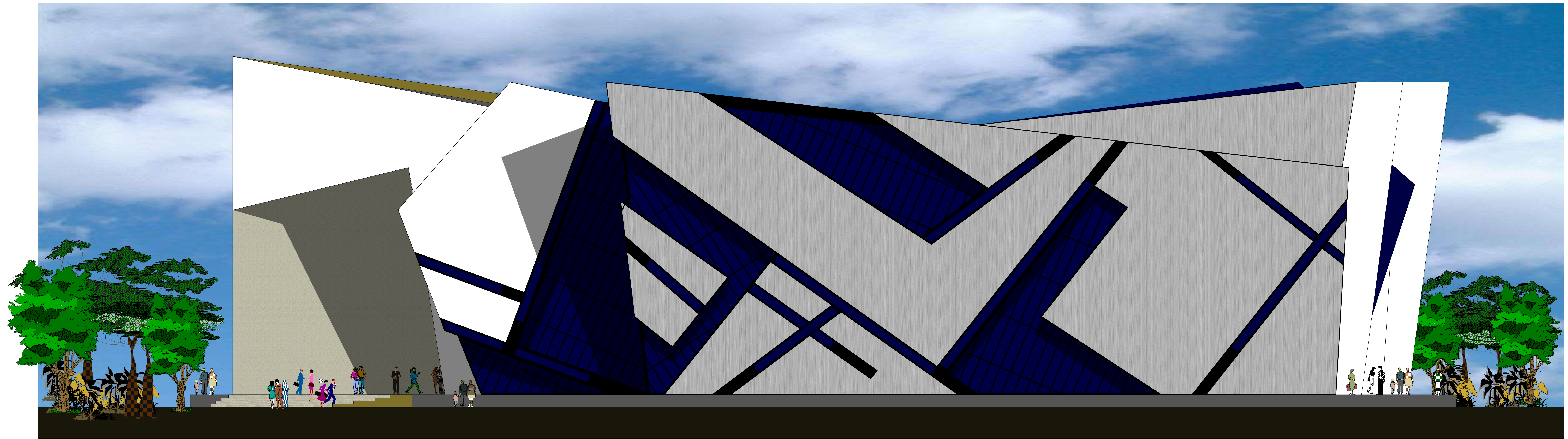
FACHADA LATERAL DERECHA Esc. 1:100
