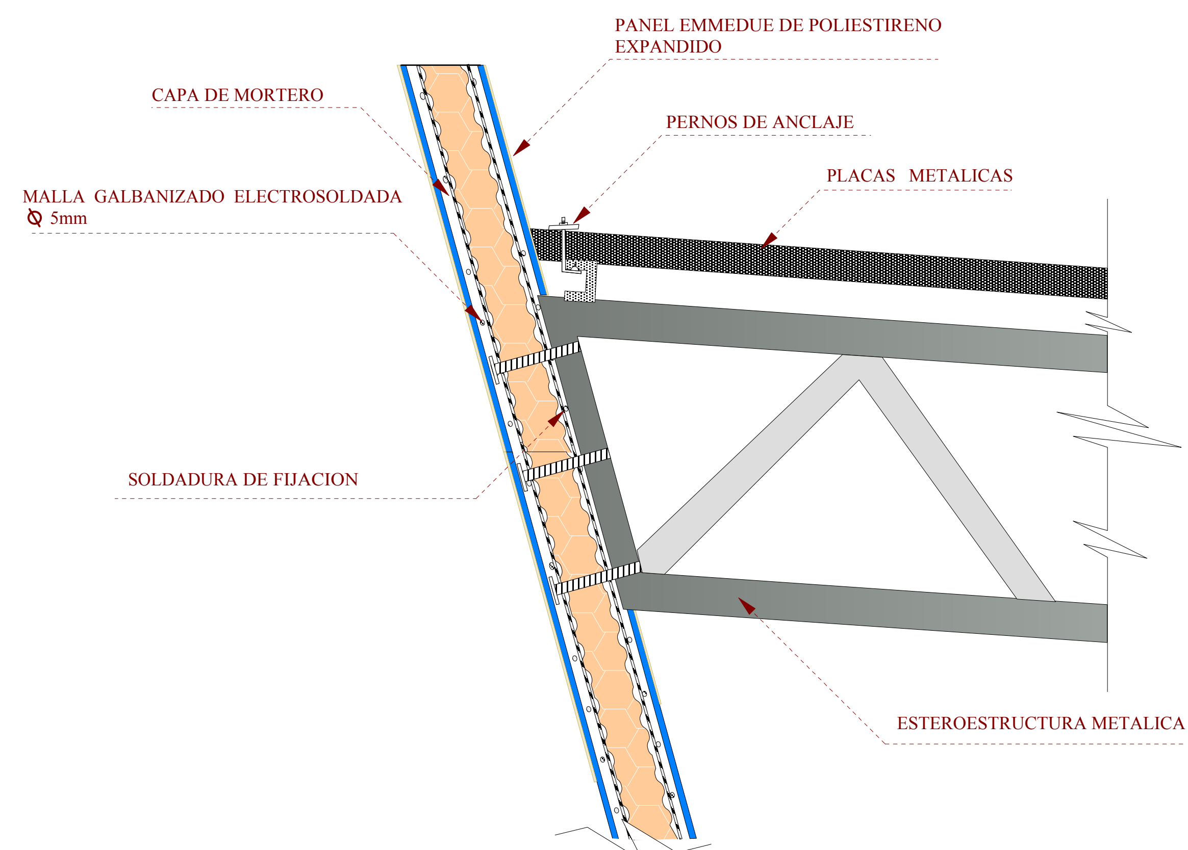
DETALLE DE UNION MURO M2 CON ESTEROESTRUCTURA. ESCALA: 1:10
