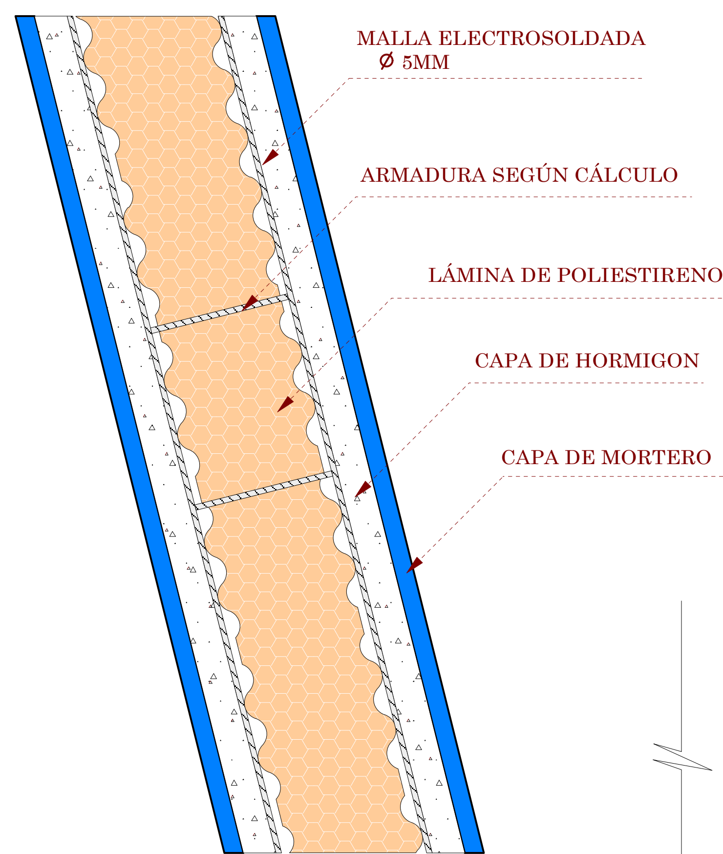
DETALLE DE MURO M2 ESCALA: 1:20
