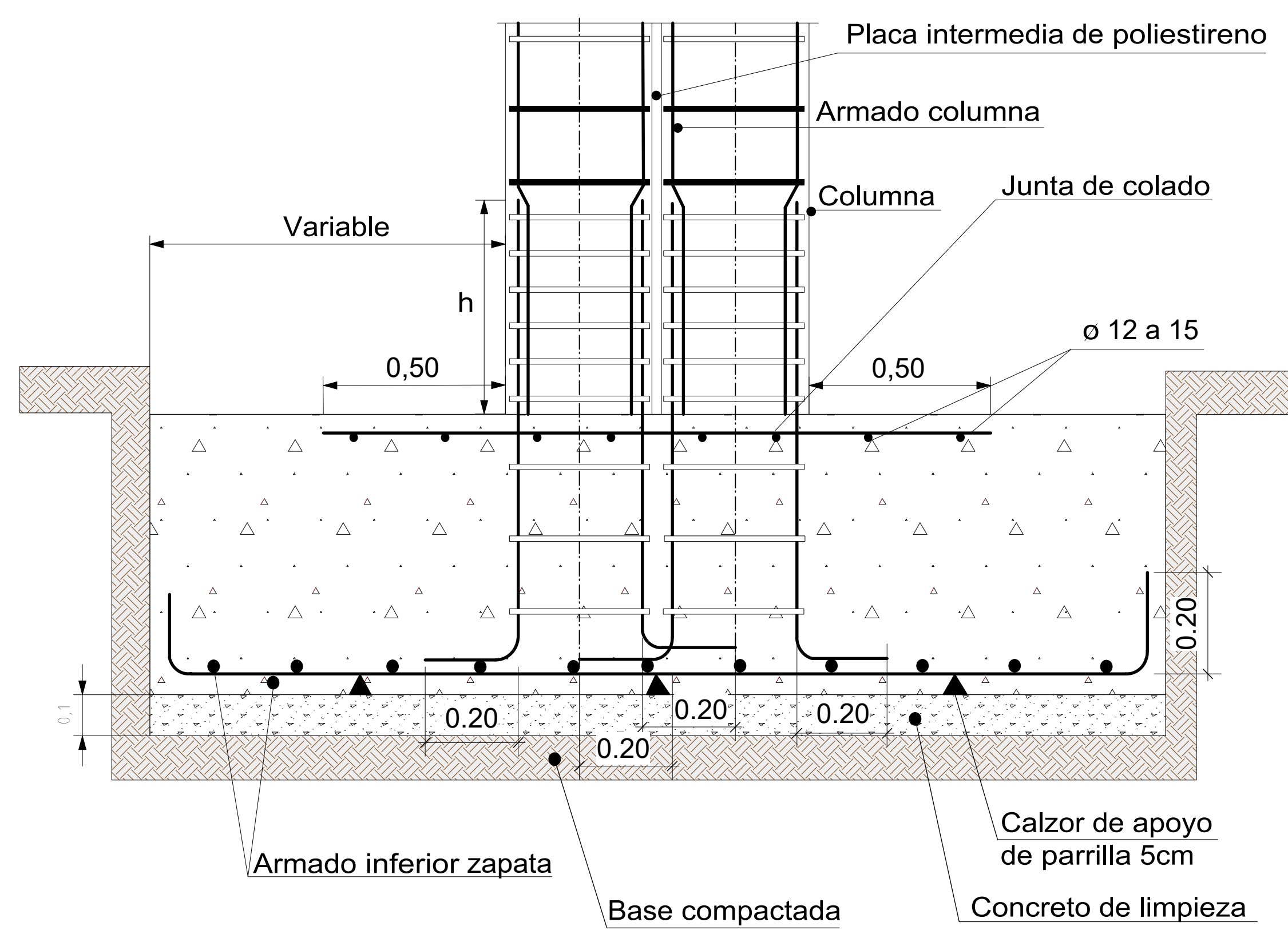
ZAPATA JUNTA DE DILATAION ESC. 1:10
