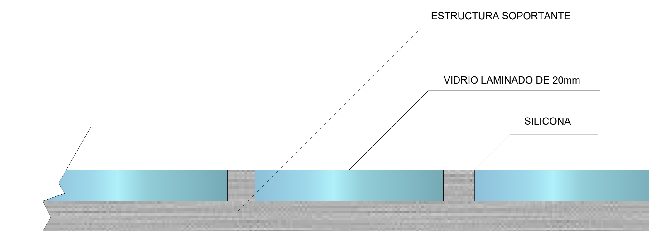
DETALLE VIDRIO PARA PISO LAMINADO ESC. 1:15
