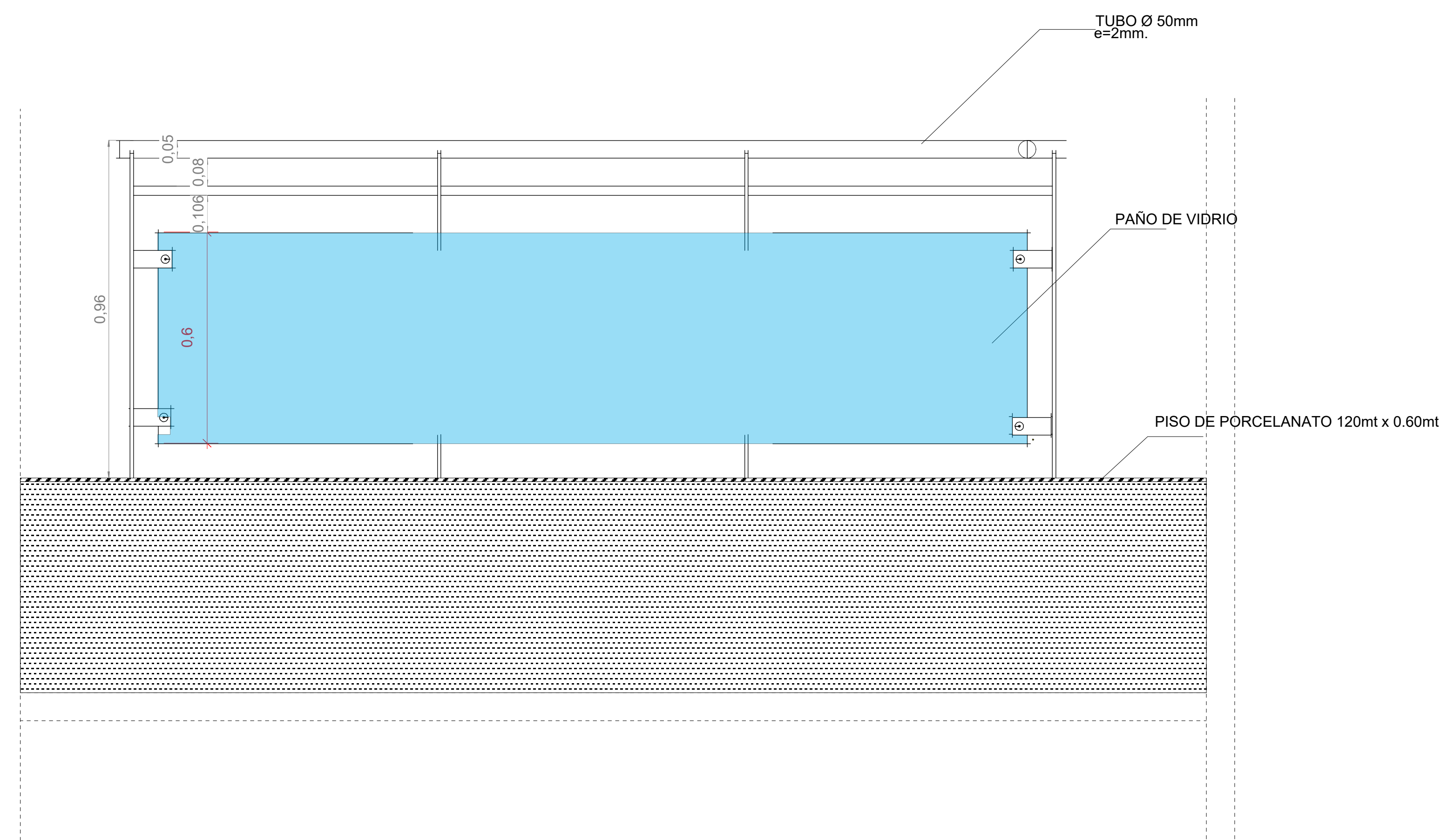
DETALLE DE BARANDA ESC: 1:10
