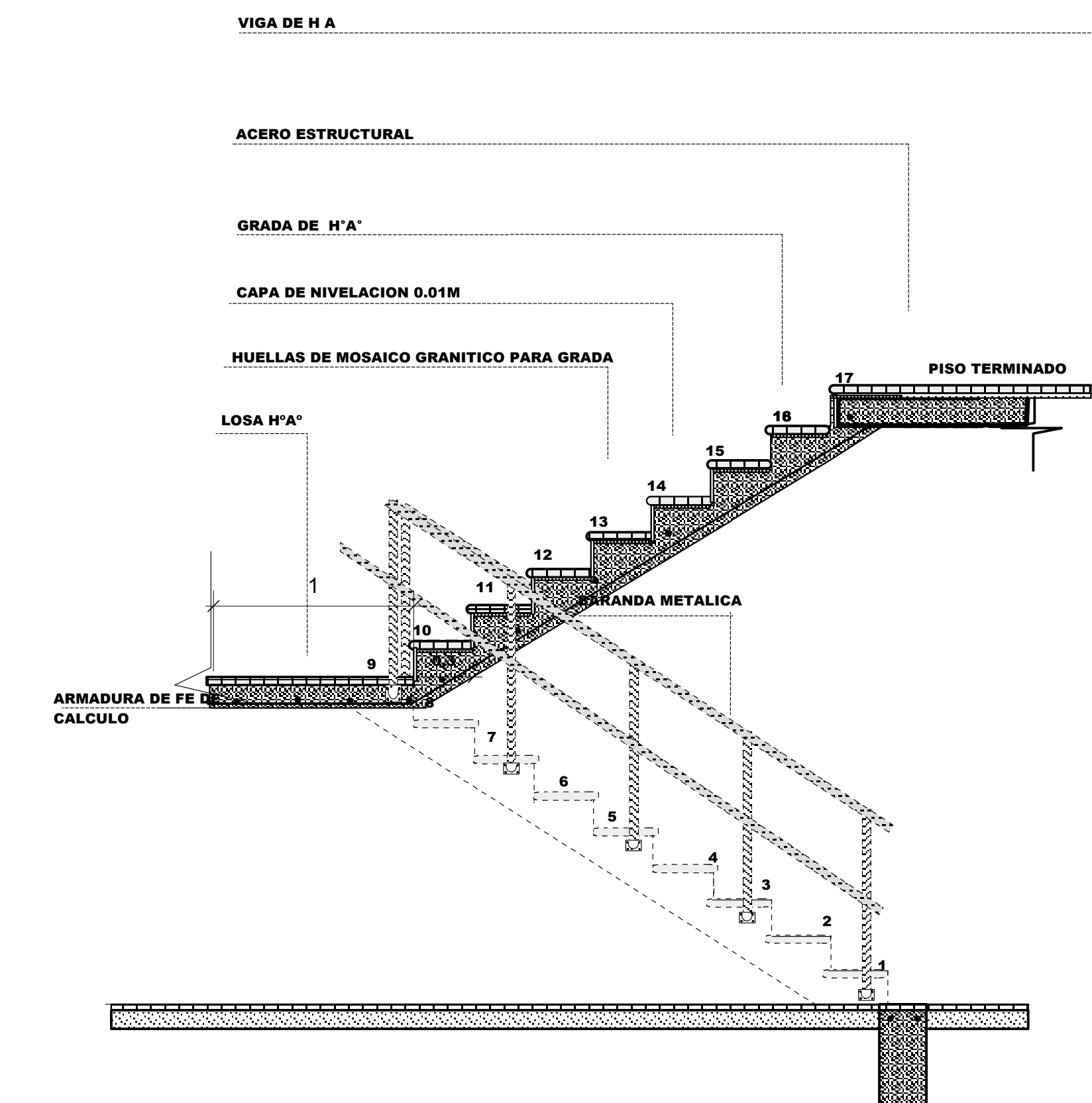
DETALLE DE GRADA DE H°A° ESC. 1:20
