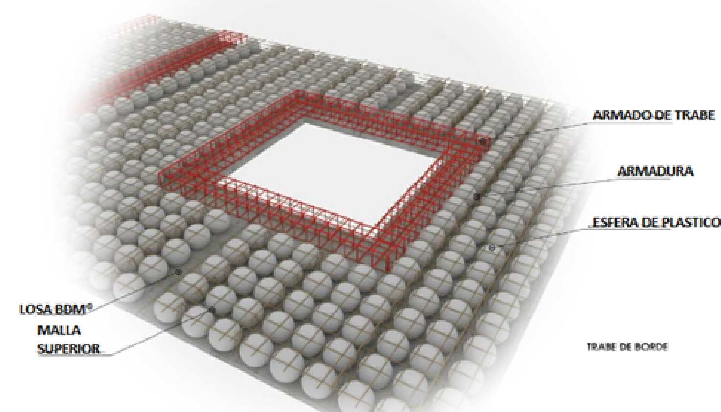
3.8.8.- Traves de Borde
