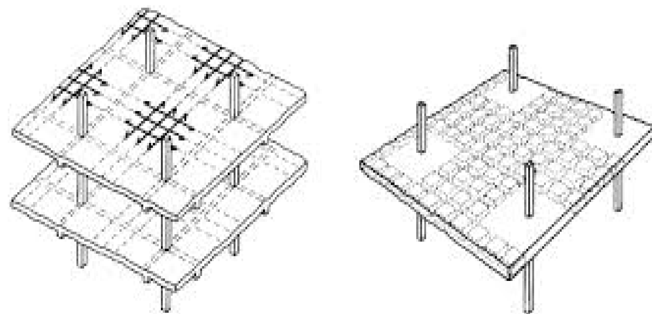
DETALLE DE LA LOSA PRENOVA ESC. 1:10
