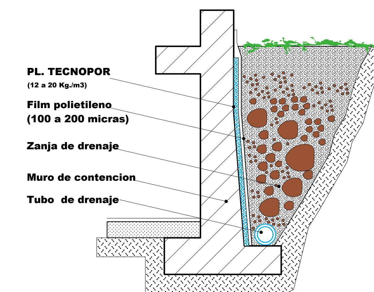
AISLAMIENTO TERMICO DE MUROS DE CONTECION O DE SOTANOS ESC. 1:20
