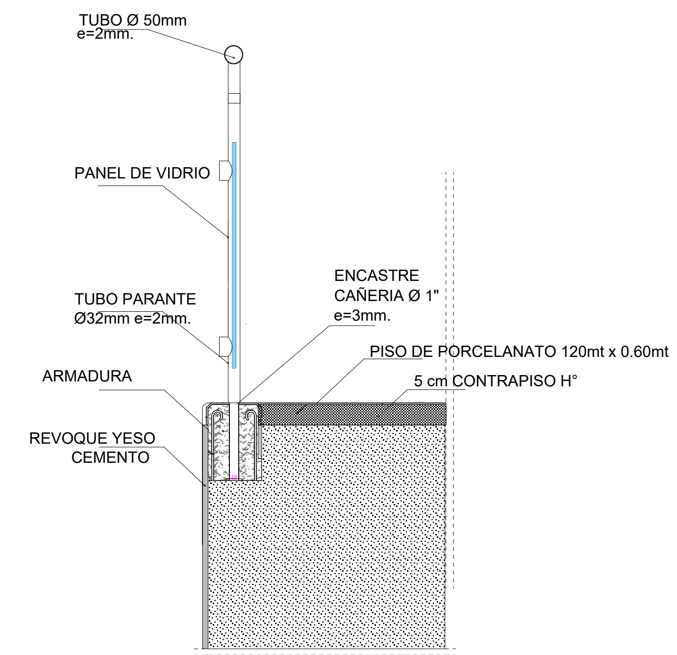
DETALLE DE BARANDA DE ALUMINIO ESC: 1:10
