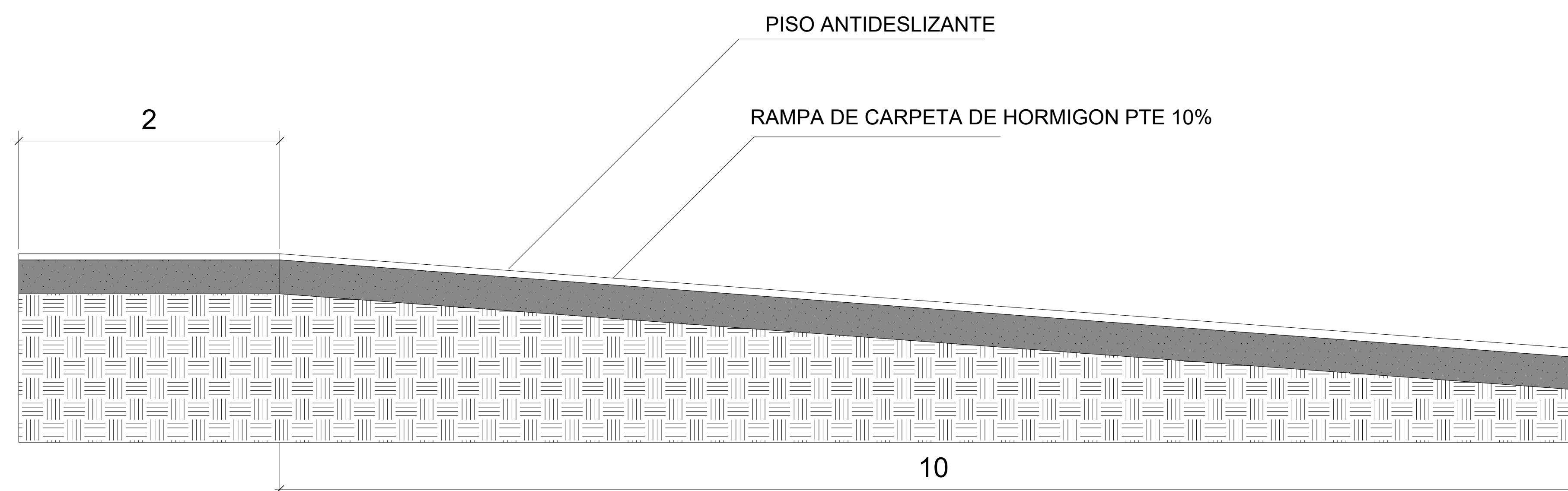
DETALLE DE RAMPA DE CARPETA DE HORMIGON ESC. 1:20
