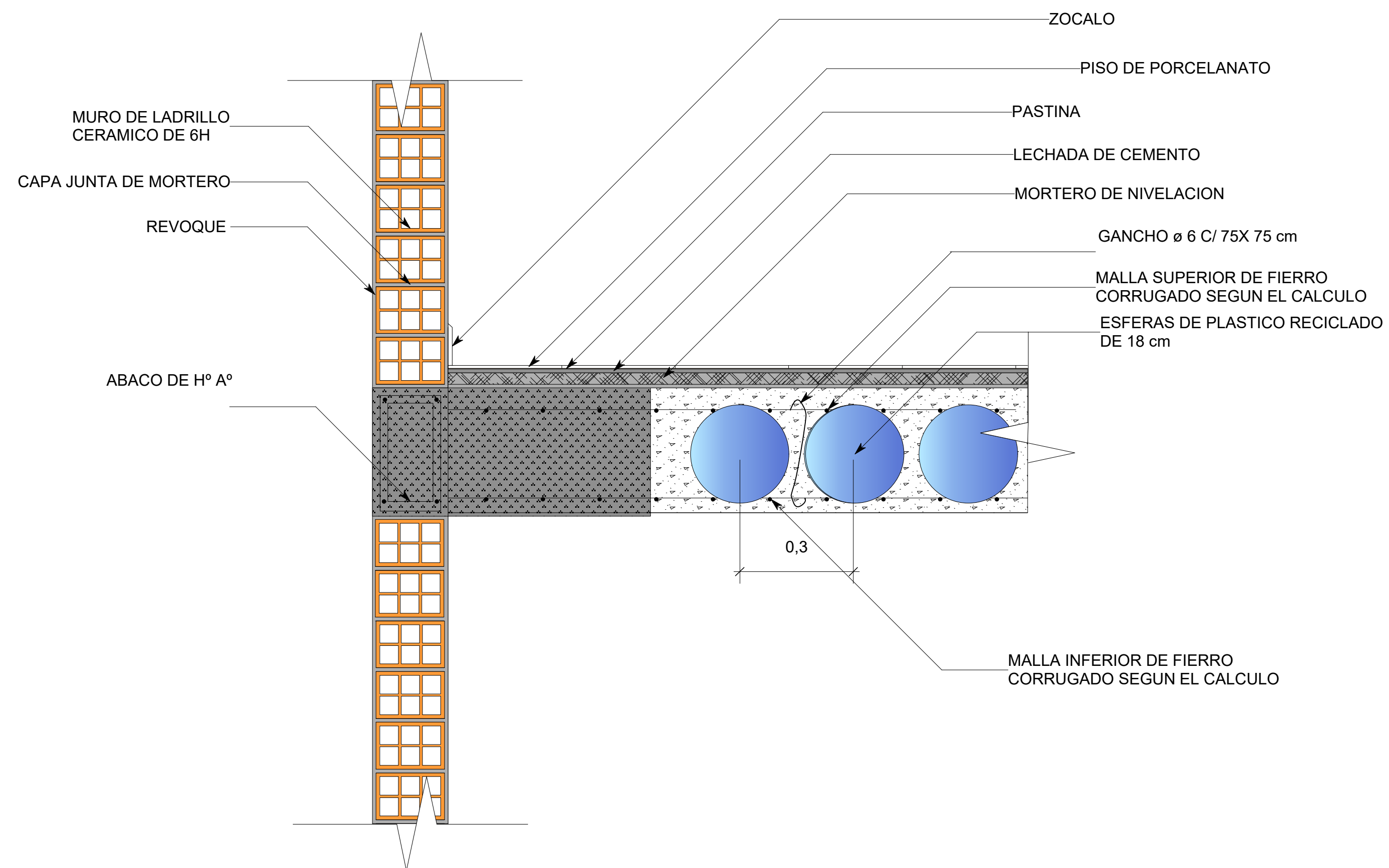
DETALLE UNIÓN DE LA LOSA PRENOVA Y EL ABACO ESC. 1:10
