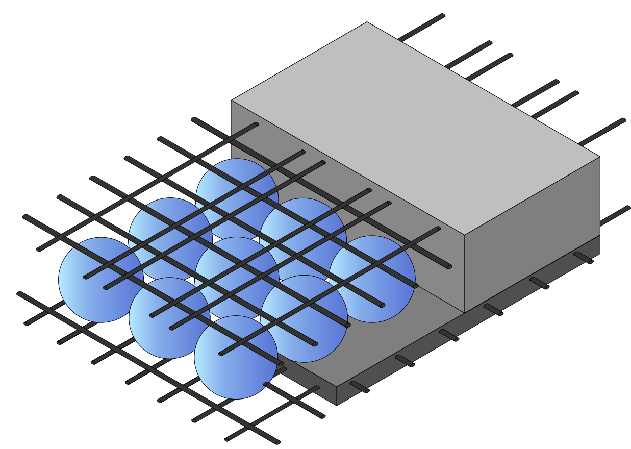
DETALLE DE LA LOSA PRENOVA ESC. 1:10
