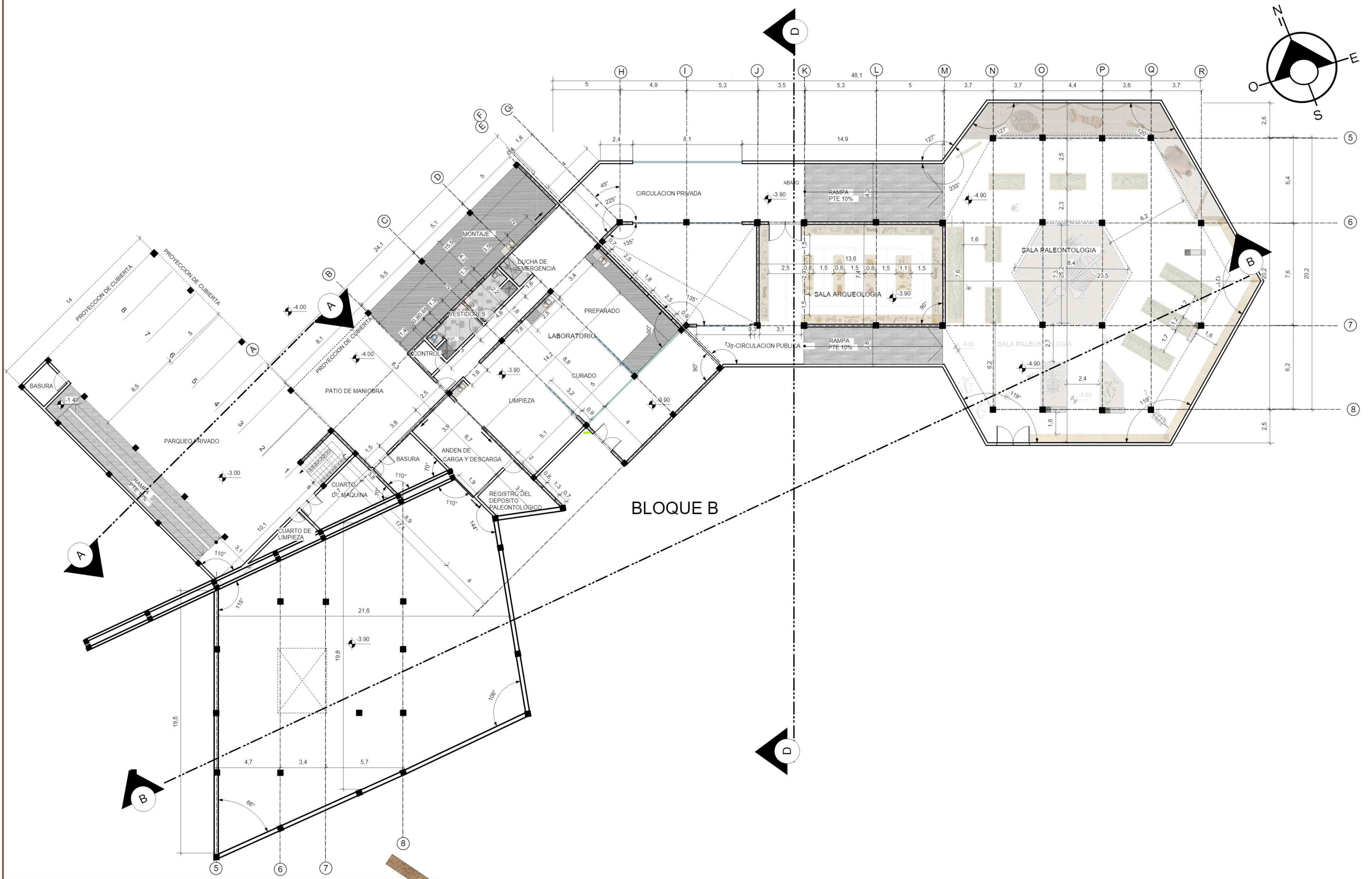
PLANO ACOTADO DEL BLOQUE B NIVEL -4.00 ESC. 1:100
