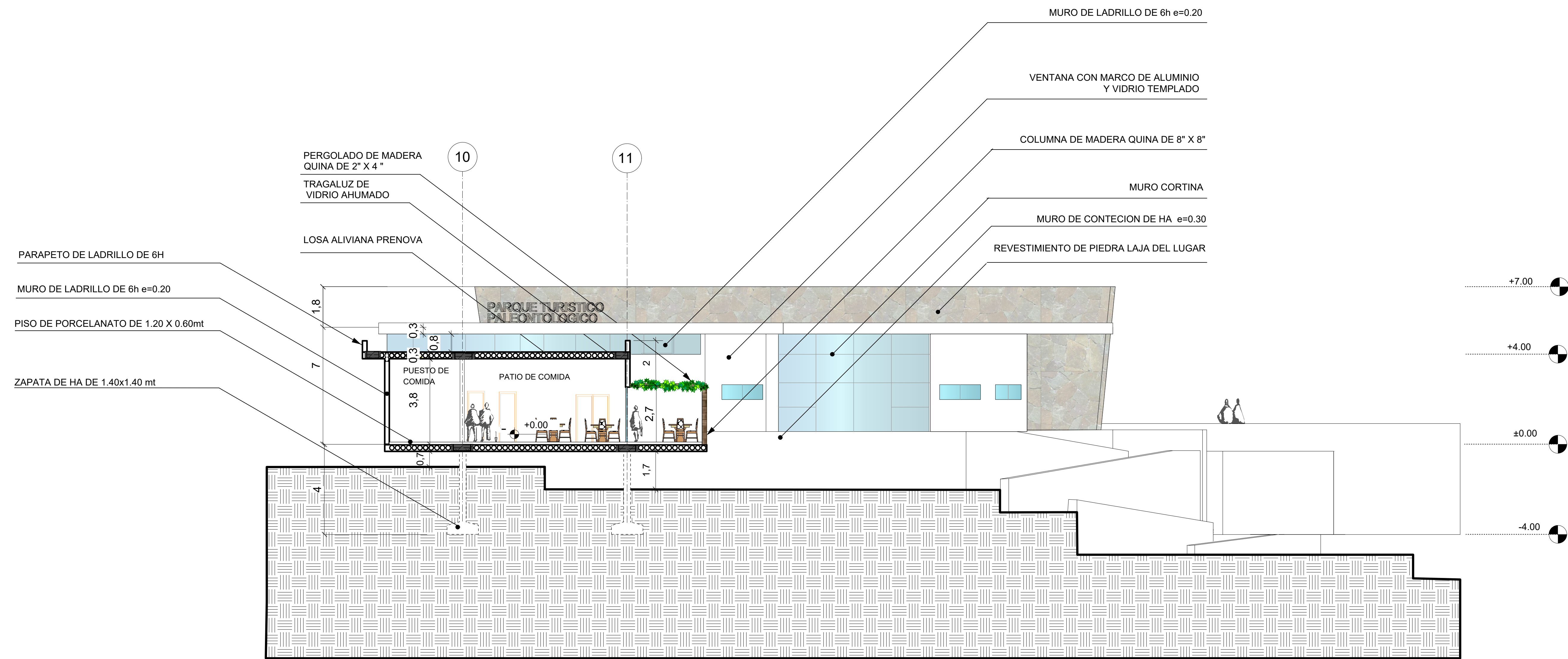
CORTE C-C"
