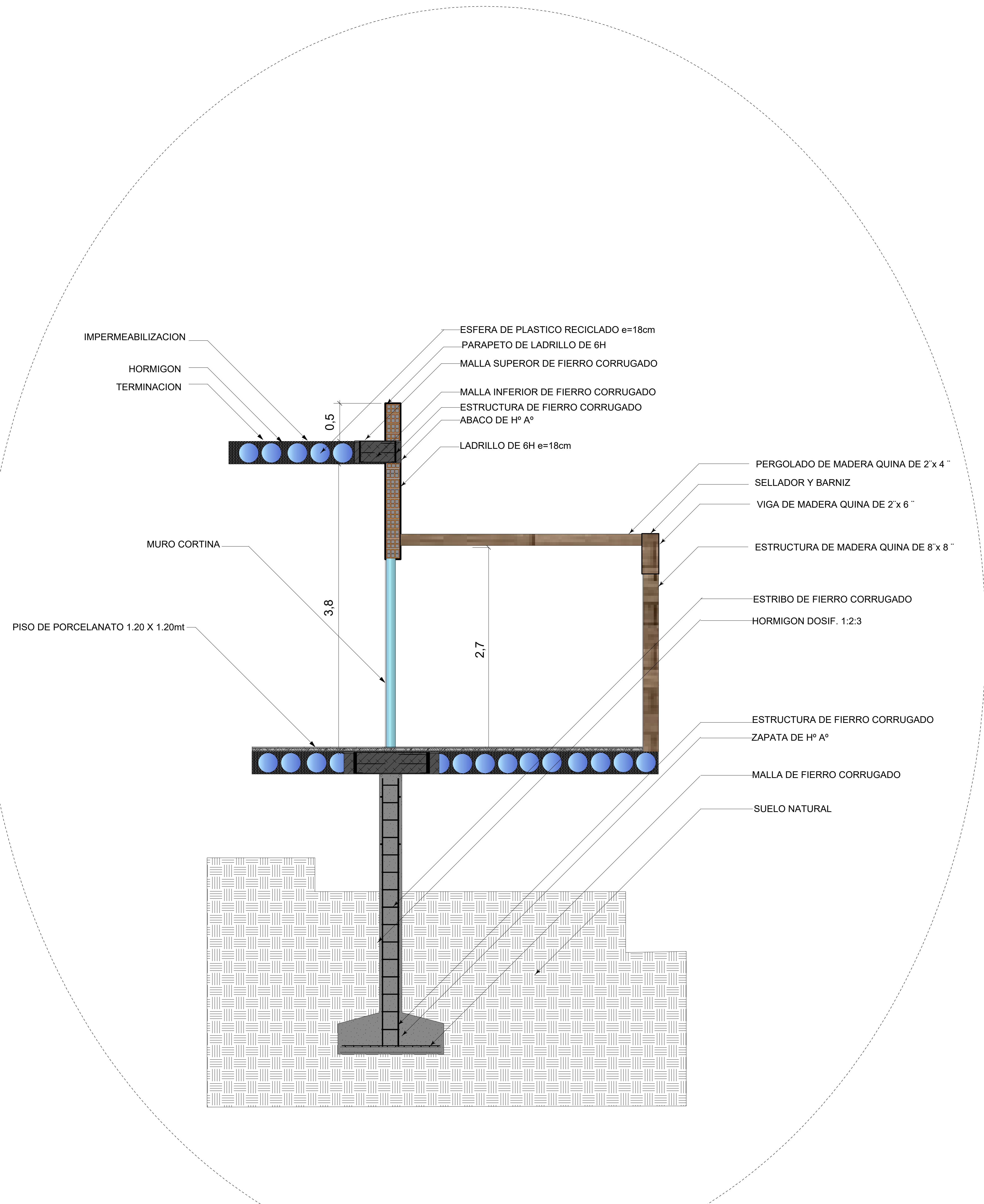
CORTE DE BORDE
