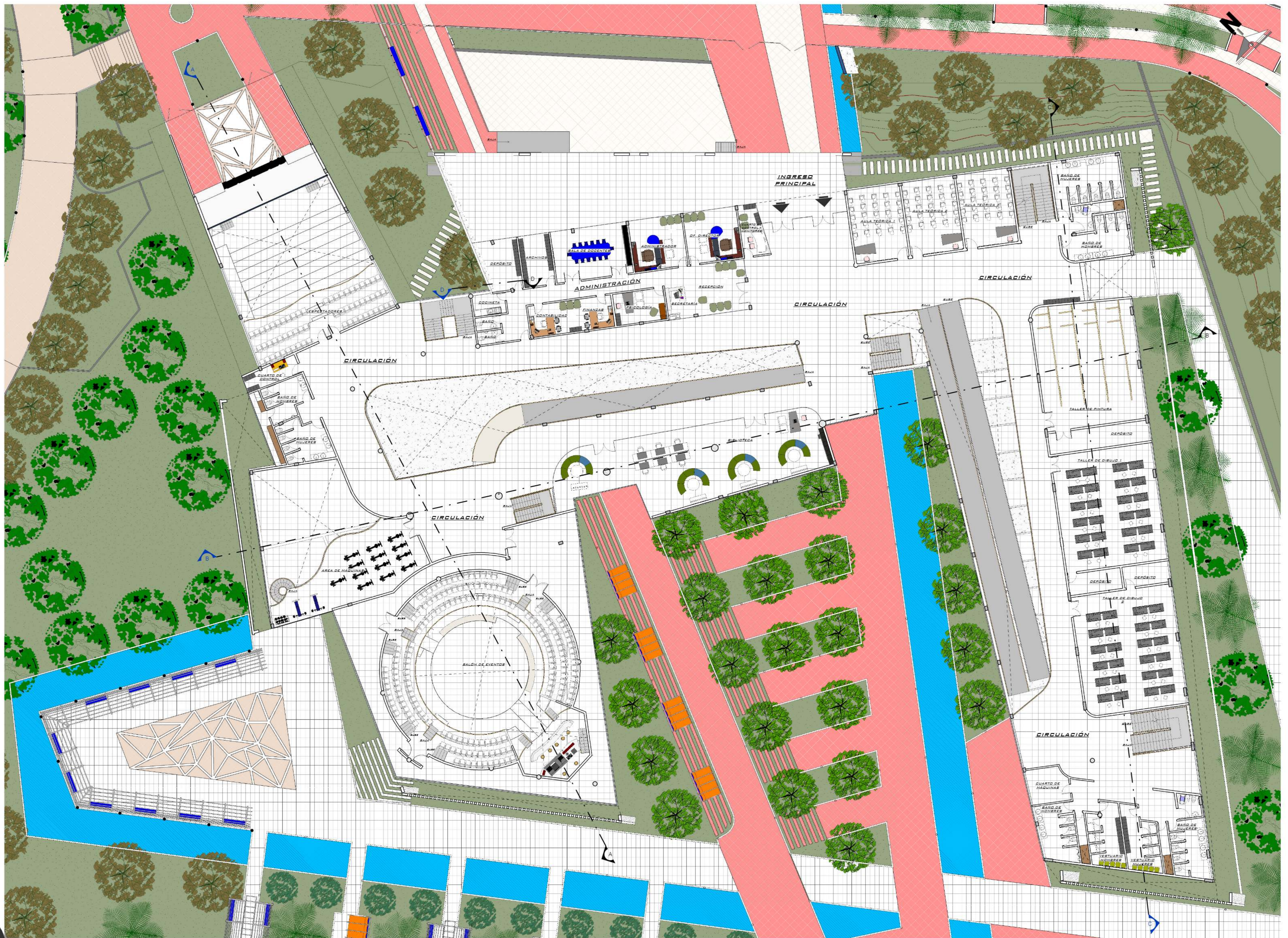
1º PLANTA AMOBLADA Esc. 1:150 CENTRO CULTURAL DE ARTE URBANO
