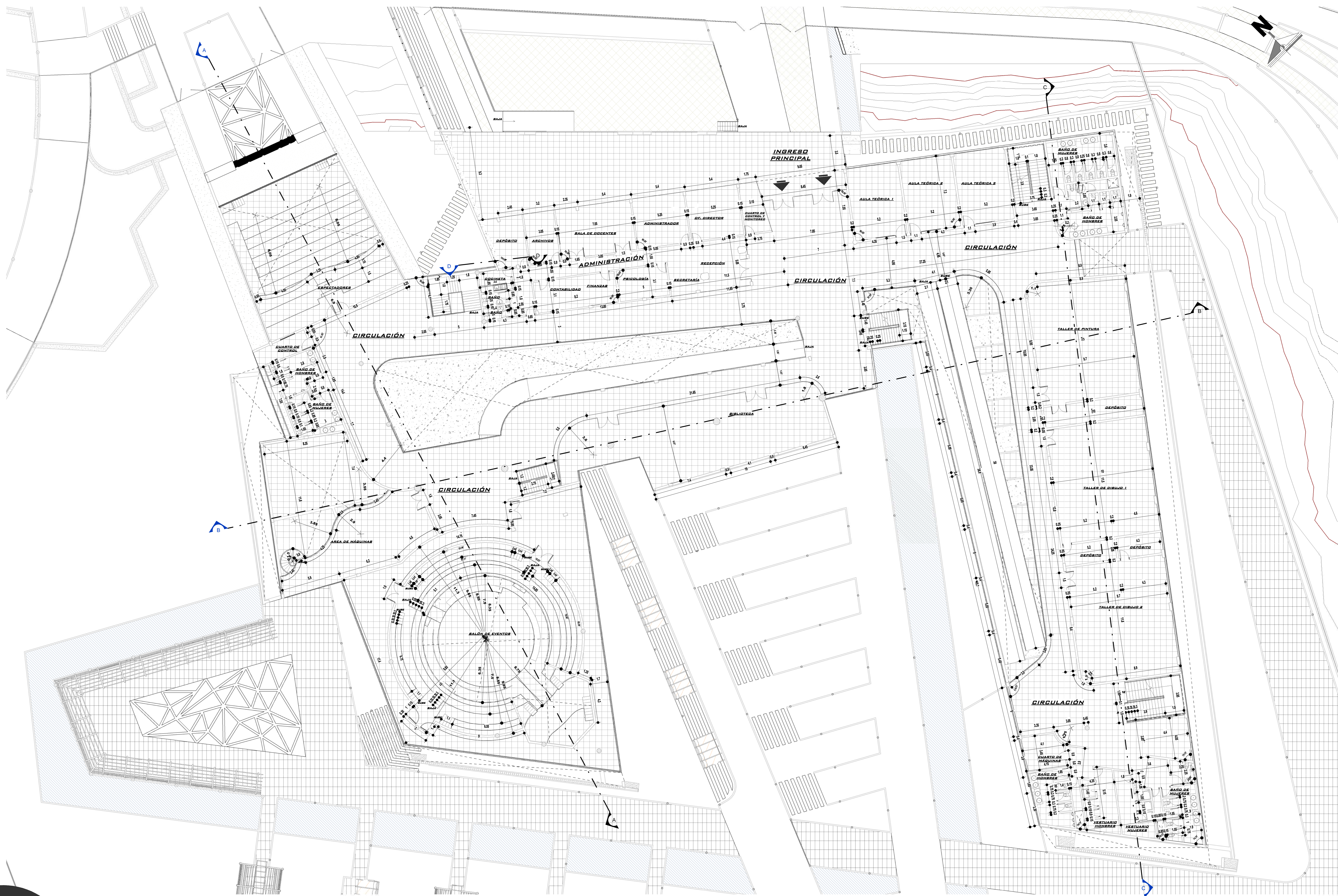
1º PLANTA ACOTADA Esc. 1:150
