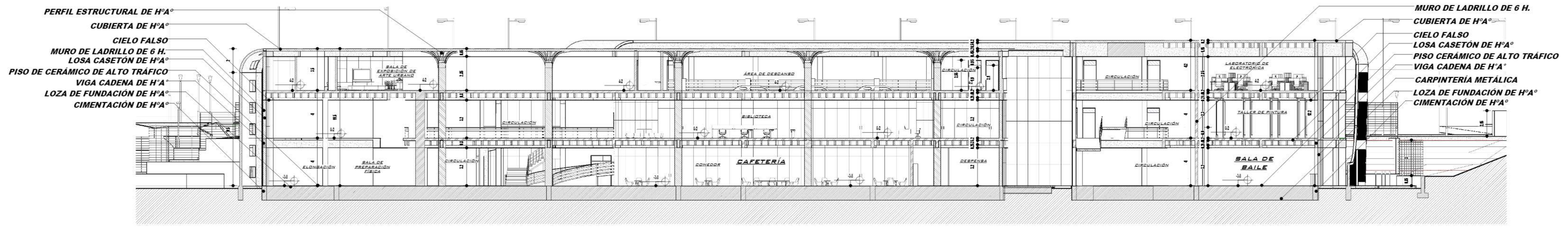
CORTE B - B' Esc. 1:150
