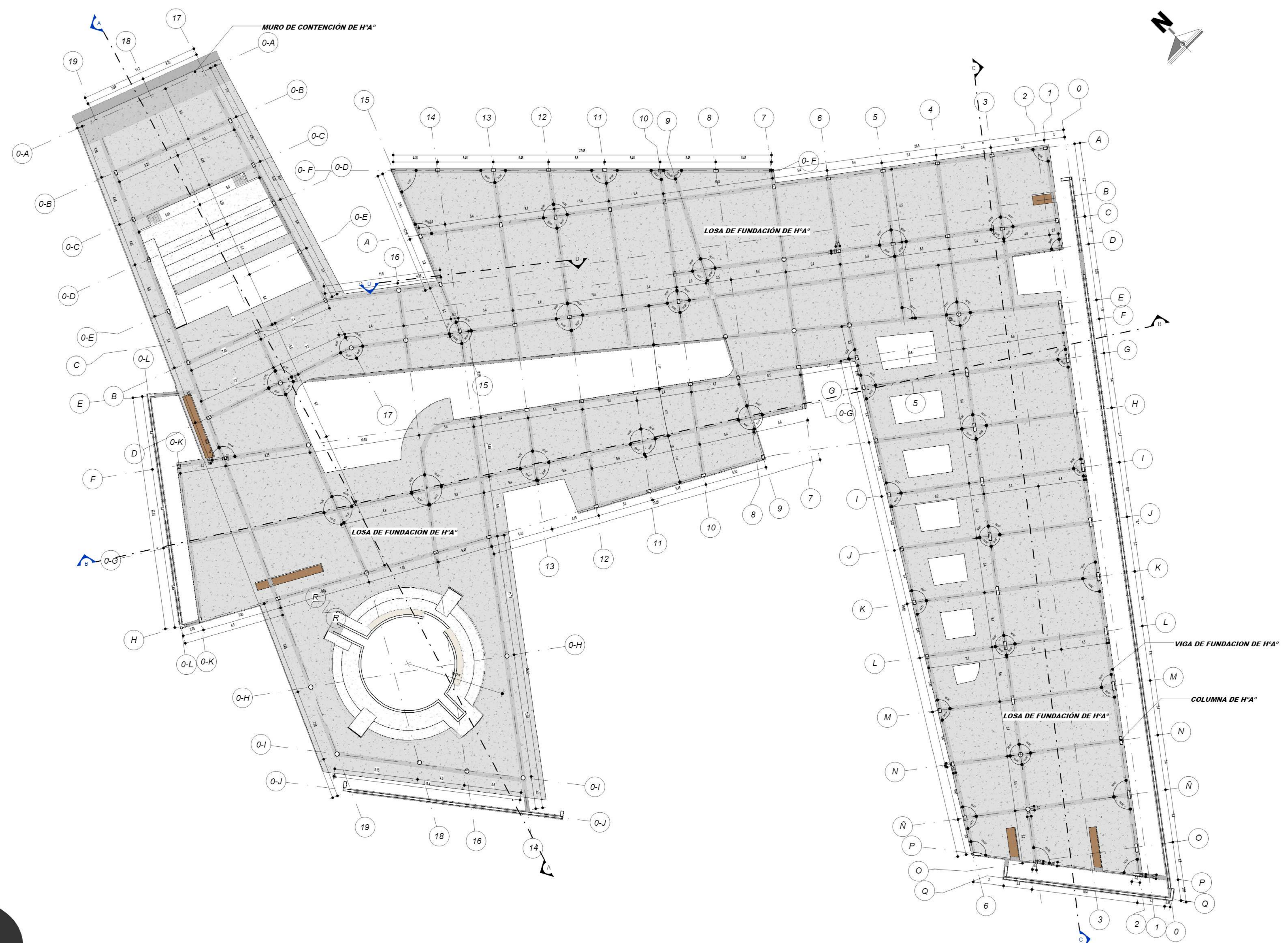
PLANO DE CIMIENTOS
