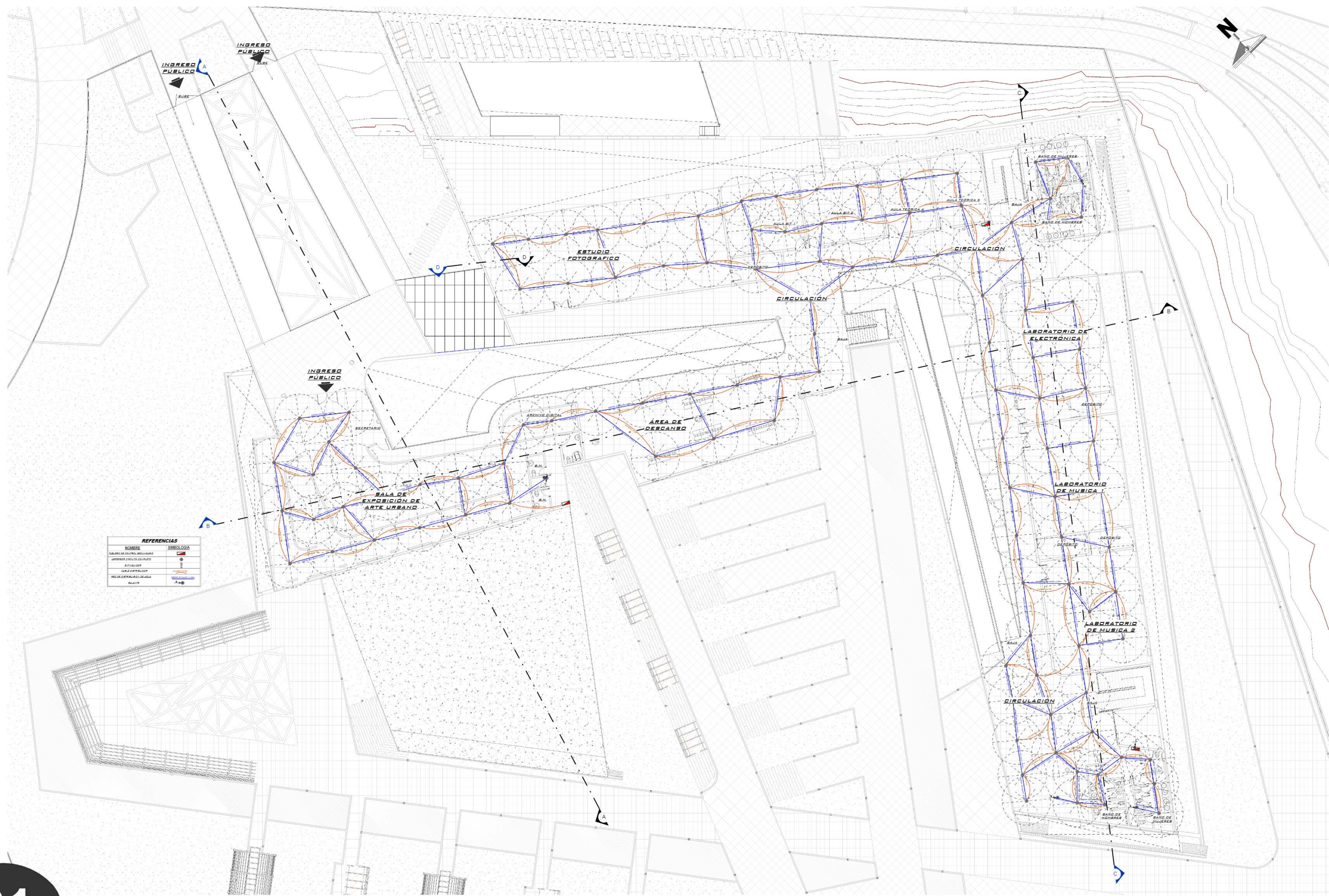
SISTEMA DE INSTALACIÓN CONTRA INCENDIOS - 2º PLANTA
