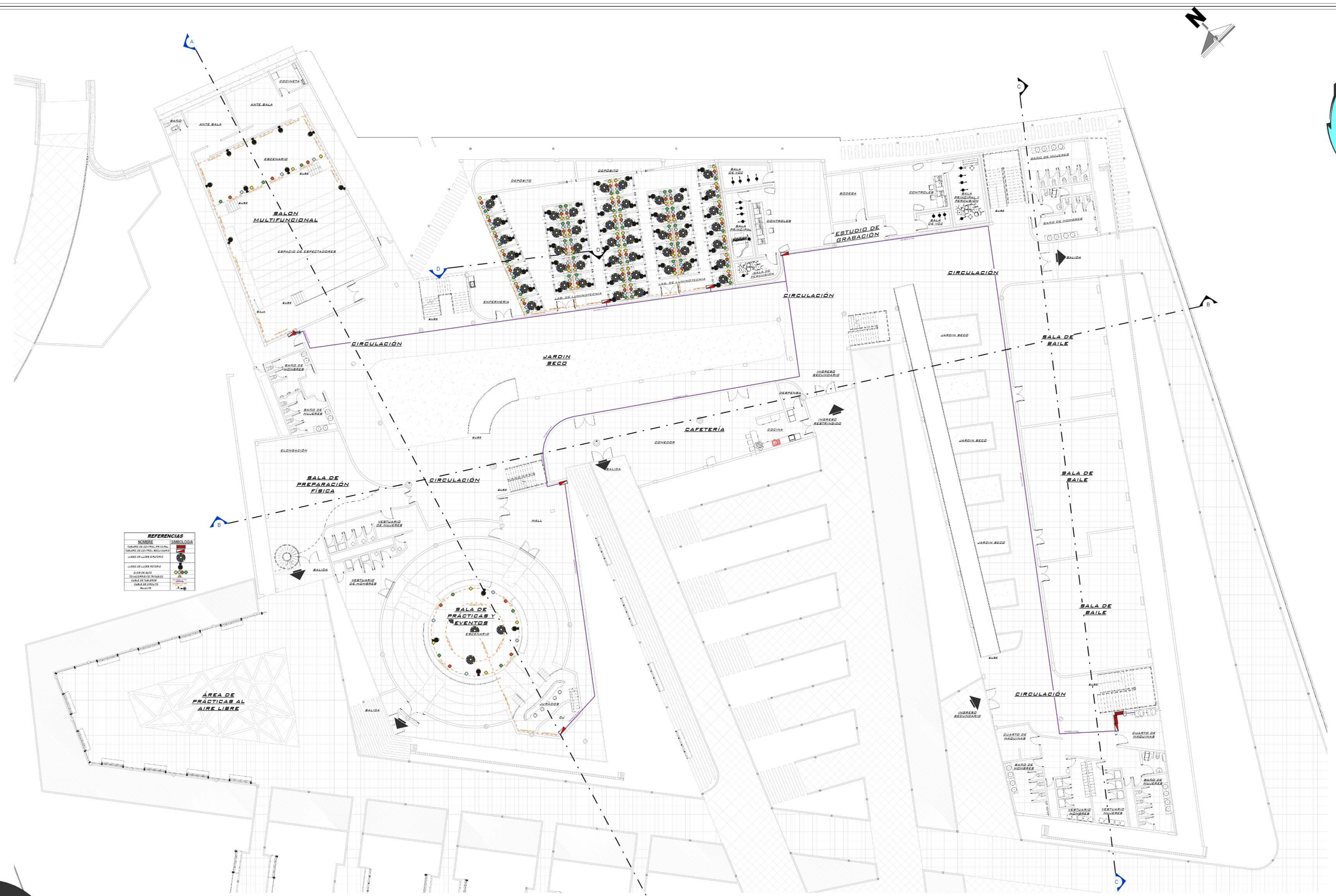
SISTEMA DE INSTALACIÓN DE LUMINOTECNIA - PLANTA BAJA
