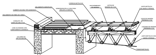
DETALLE DE LA CUBIERTA Y ESTRUCTURA DEL GIMNASIO
