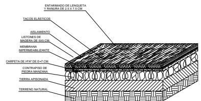
DETALLE DEL PISO DEL GIMNASIO
