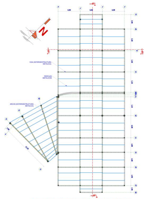
CUBIERTA SISTEMA ESTRUCTURAL- BLOQUE PERNOCTACION
