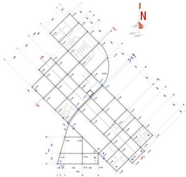
PLANO DE FUNDACIONES – (BLOQUE DE PERNOCTACION)
