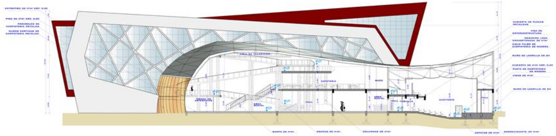
CORTE B-B''
