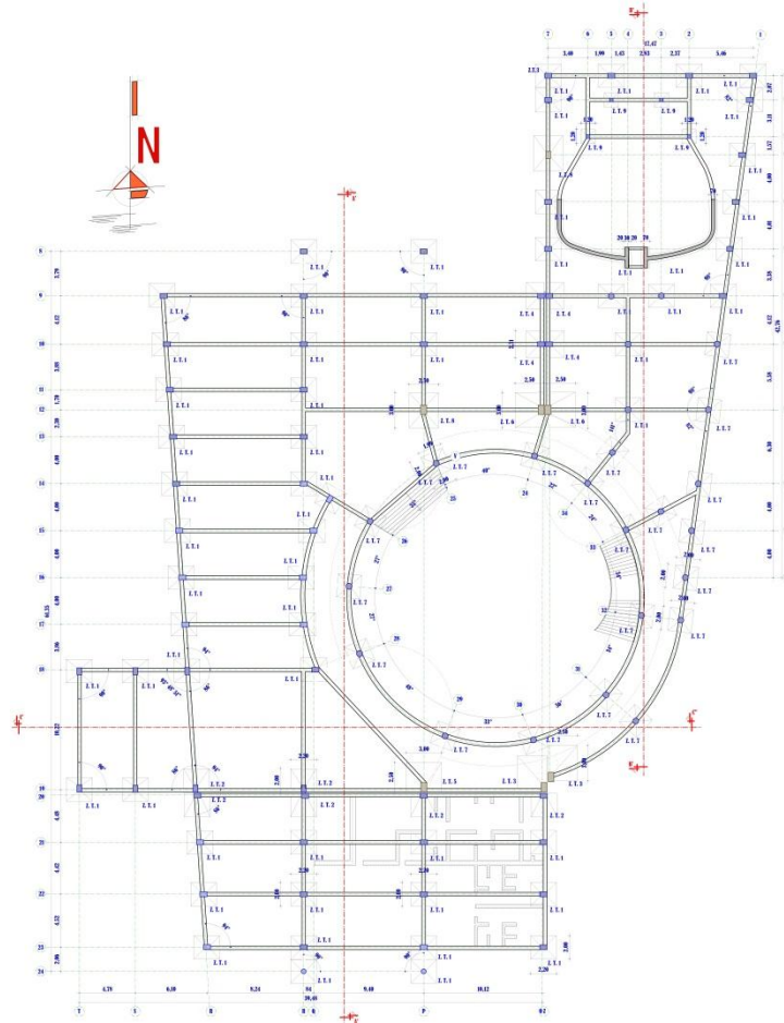
PLANO DE FUNDACIONES – (BLOQUE DE INTERPRETACION)
