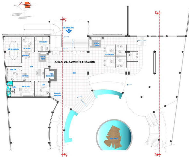
NIVEL 1.20m. (AREA DE SOCIAL) – BLOQUE DE INTERPRETACION
