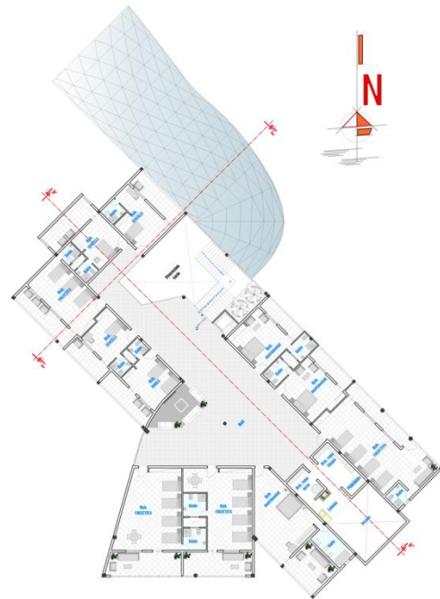
PLANTA ALTA – BLOQUE PERNOCTACION
