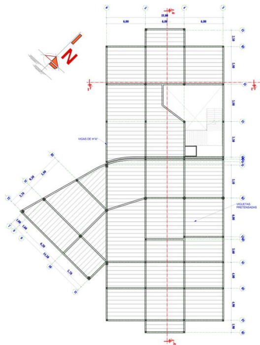
PLANTA ALTA SISTEMA ESTRUCTURAL - BLOQUE PERNOCTACION
