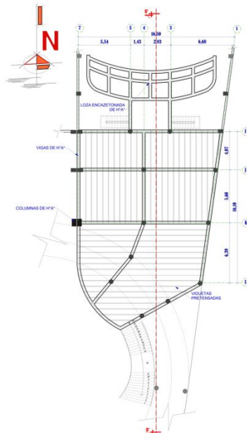
PLANO SISTEMA ESTRUCTURAL - NIVEL 4.00 m. - BLOQUE INTERPRETACION ESC. 1:100 CAFETERIA
