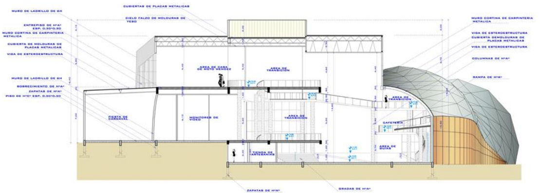
CORTE C-C''
