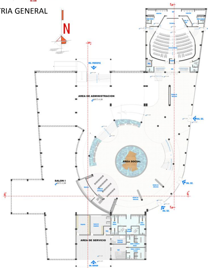
PLANTA BAJA (AREA DE SOCIAL) – BLOQUE DE INTERPRETACION
