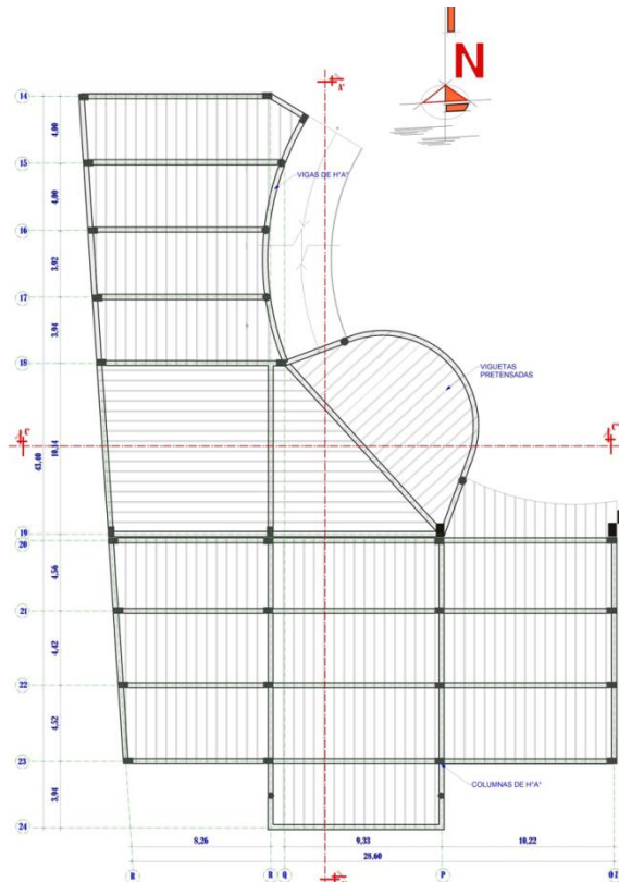
PLANO SISTEMA ESTRUCTURAL - NIVEL 10.00m. - BLOQUE INTERPRETACION
