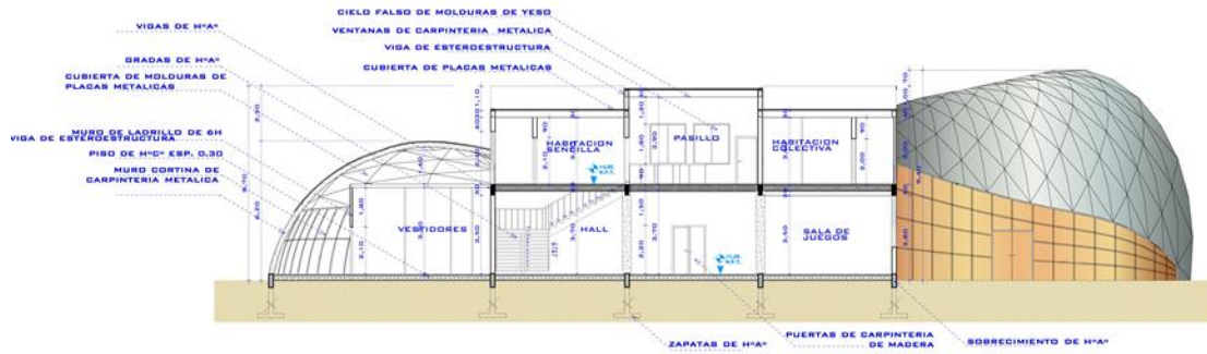
CORTE D-D''
