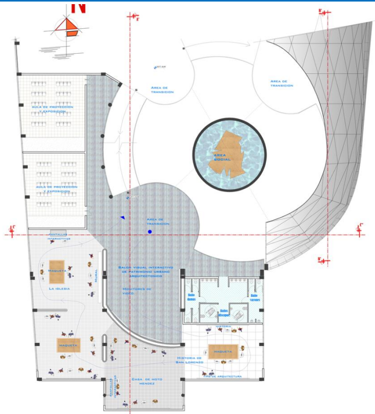
NIVEL 10.00m. (SALON 3) – BLOQUE DE INTERPRETACION
