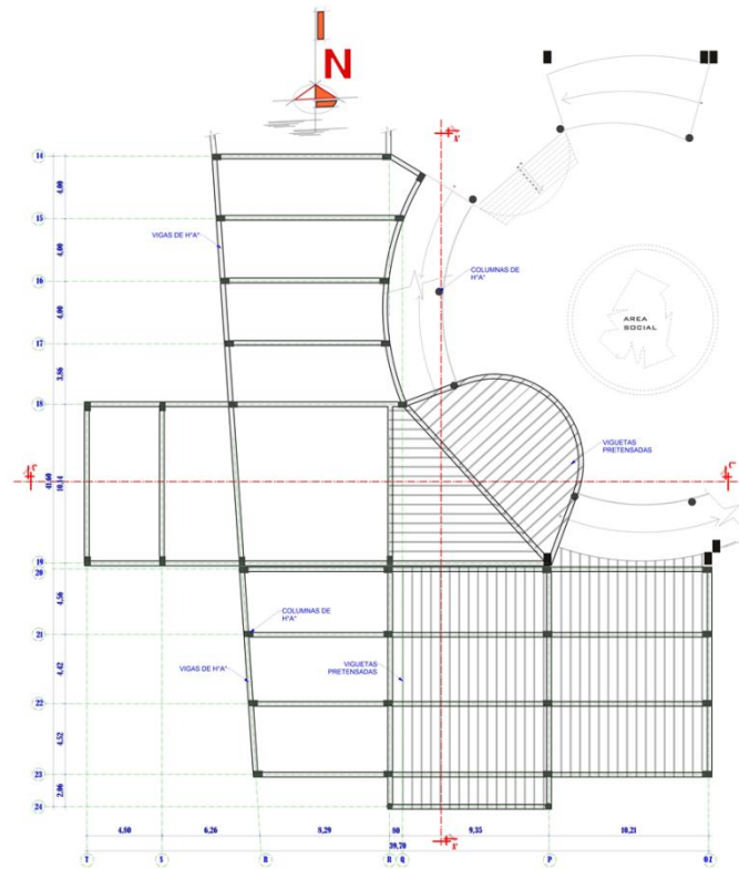
PLANO SISTEMA ESTRUCTURAL - NIVEL 2.90m. - BLOQUE INTERPRETACION ESC. 1:100 SALON I
