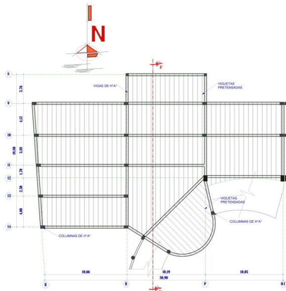
PLANO SISTEMA ESTRUCTURAL - NIVEL 8.40m. - BLOQUE INTERPRETACION ESC. 1:100 SALON II
