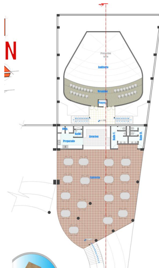
NIVEL 4.00m. (CAFETERIA) – BLOQUE DE INTERPRETACION
