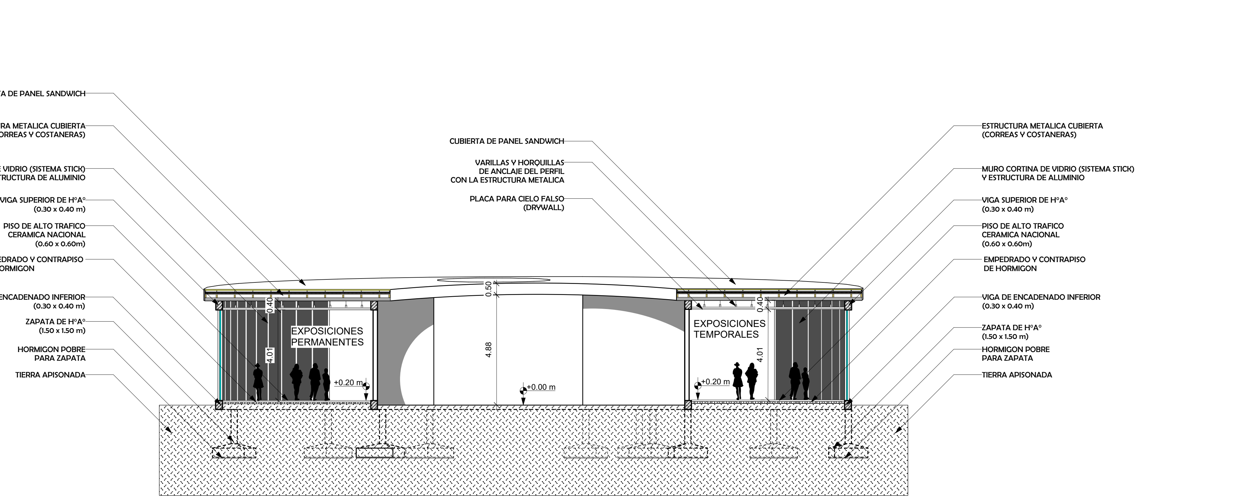
CORTE E'-E' Esc. 1:100
