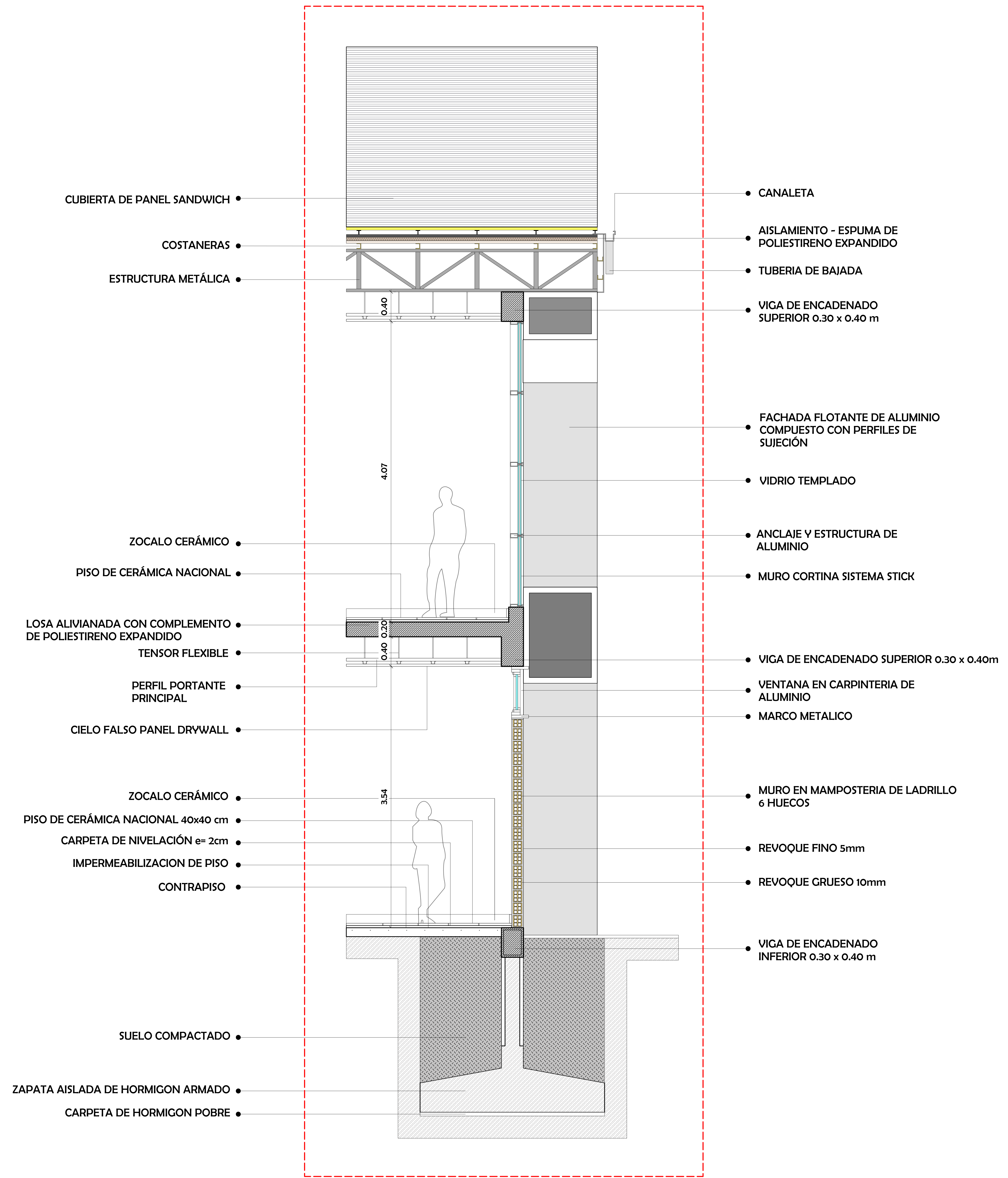
CORTE DE BORDE - ESC. 1:20
