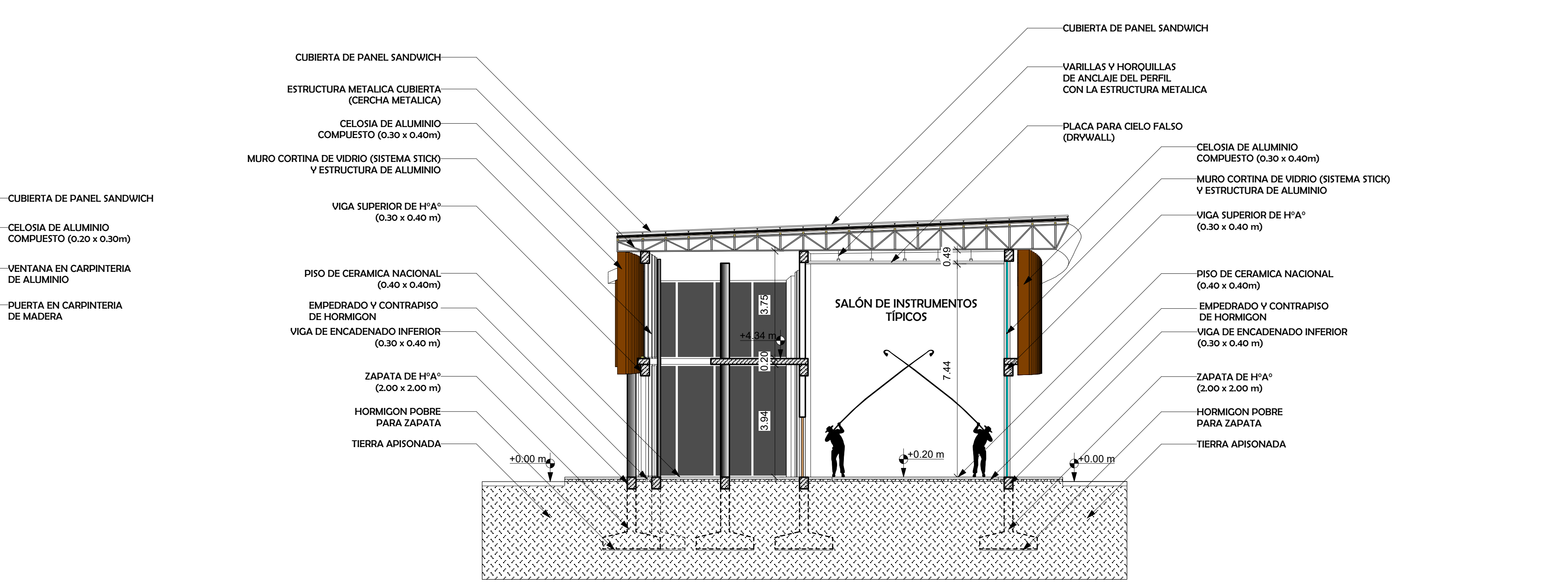
CORTE C'-C' Esc. 1:100
