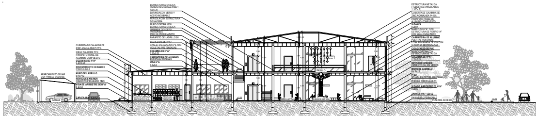
4 CORTE D-D 1:100
