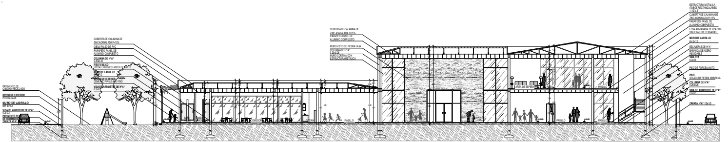
1 CORTE A-A 1:100
