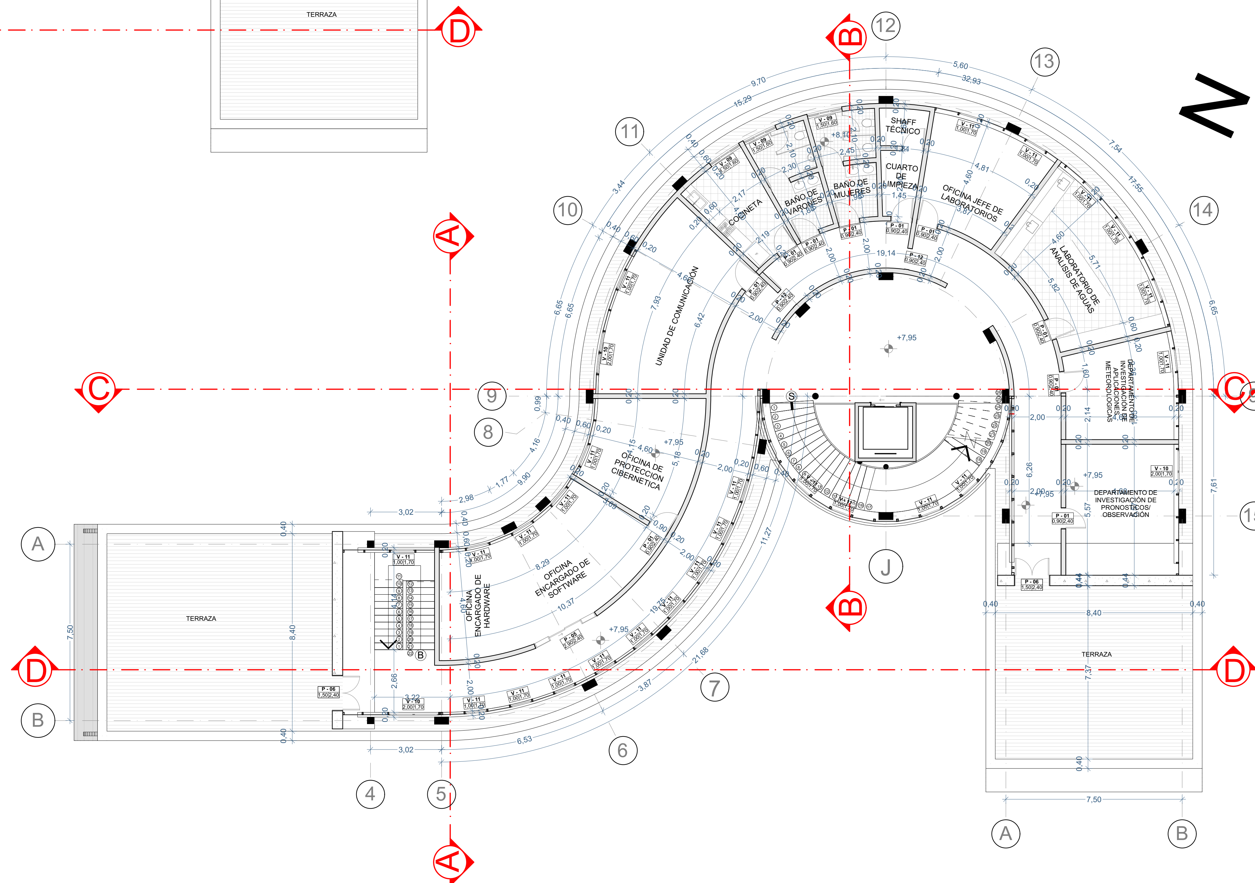
SEGUNDO PISO PLANTA ACOTADA ESC: 1:100
