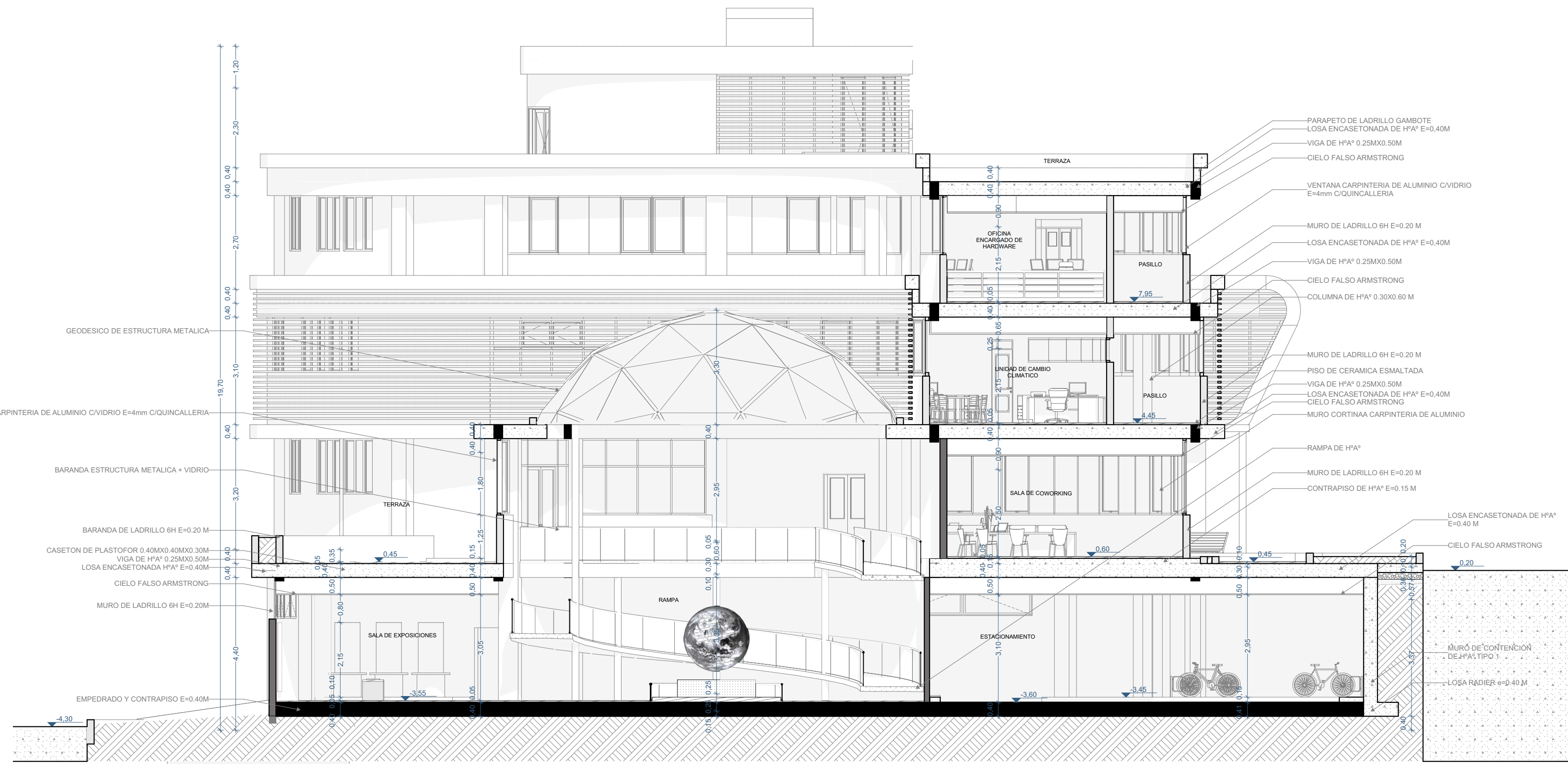
CORTE A - A' ESC: 1:100
