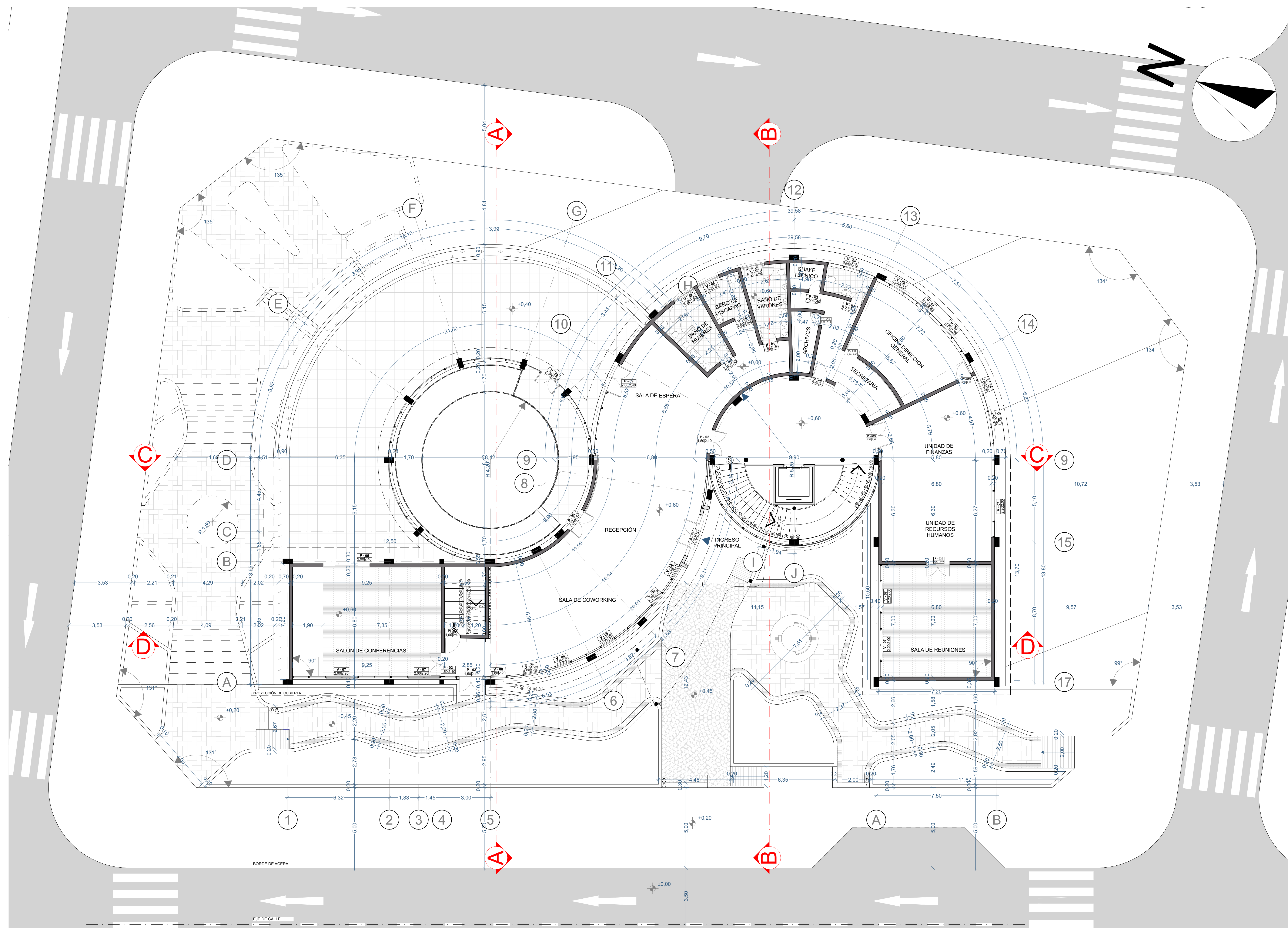
PLANTA BAJA ACOTADA ESC: 1:100
