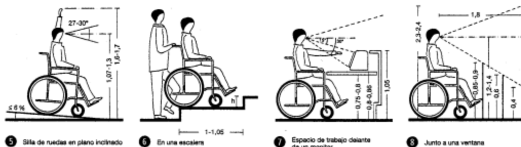
5 Silla de ruedas en plano inclinado
