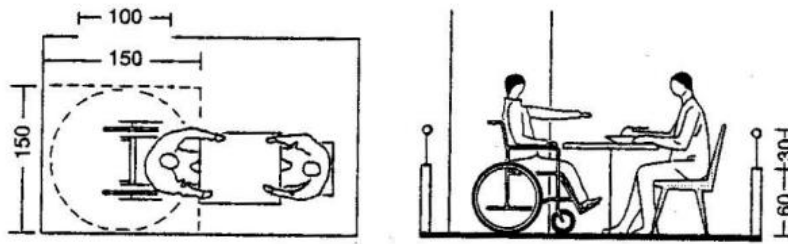
5 Espacio libre: planta
