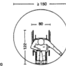
12 Espacio mínimo de giro
