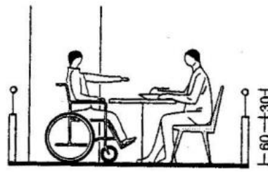
6 Espacio libre: alzado
