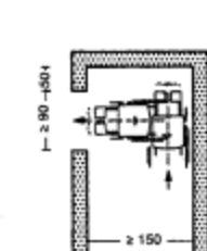
13 Anchura de paso con 1 puerta
