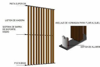
DETALLE ESTRUCTURA DE MADERA ESC: 1:10
