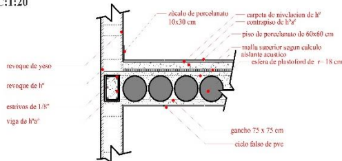
DETALLE CONSTRUCTIVO DE LOSA PRENOVA ESC: 1:20
