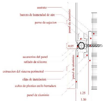
DETALLE DE LA FACHADA FALSA DE ALUCUBOND ESC: 1:20
