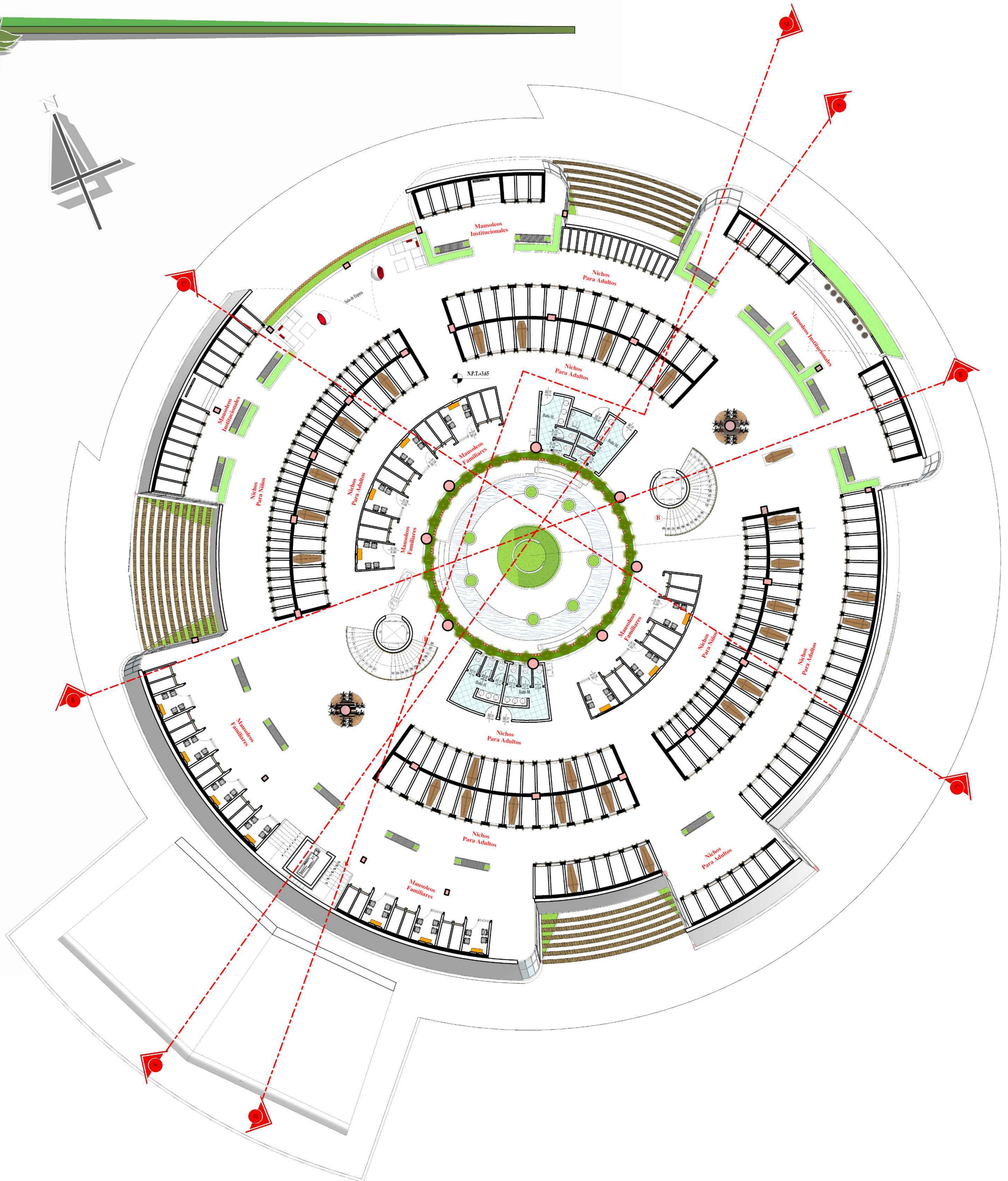
--PLANO DE PRIMER PISO AMOBLADO-- ESC:1:100
