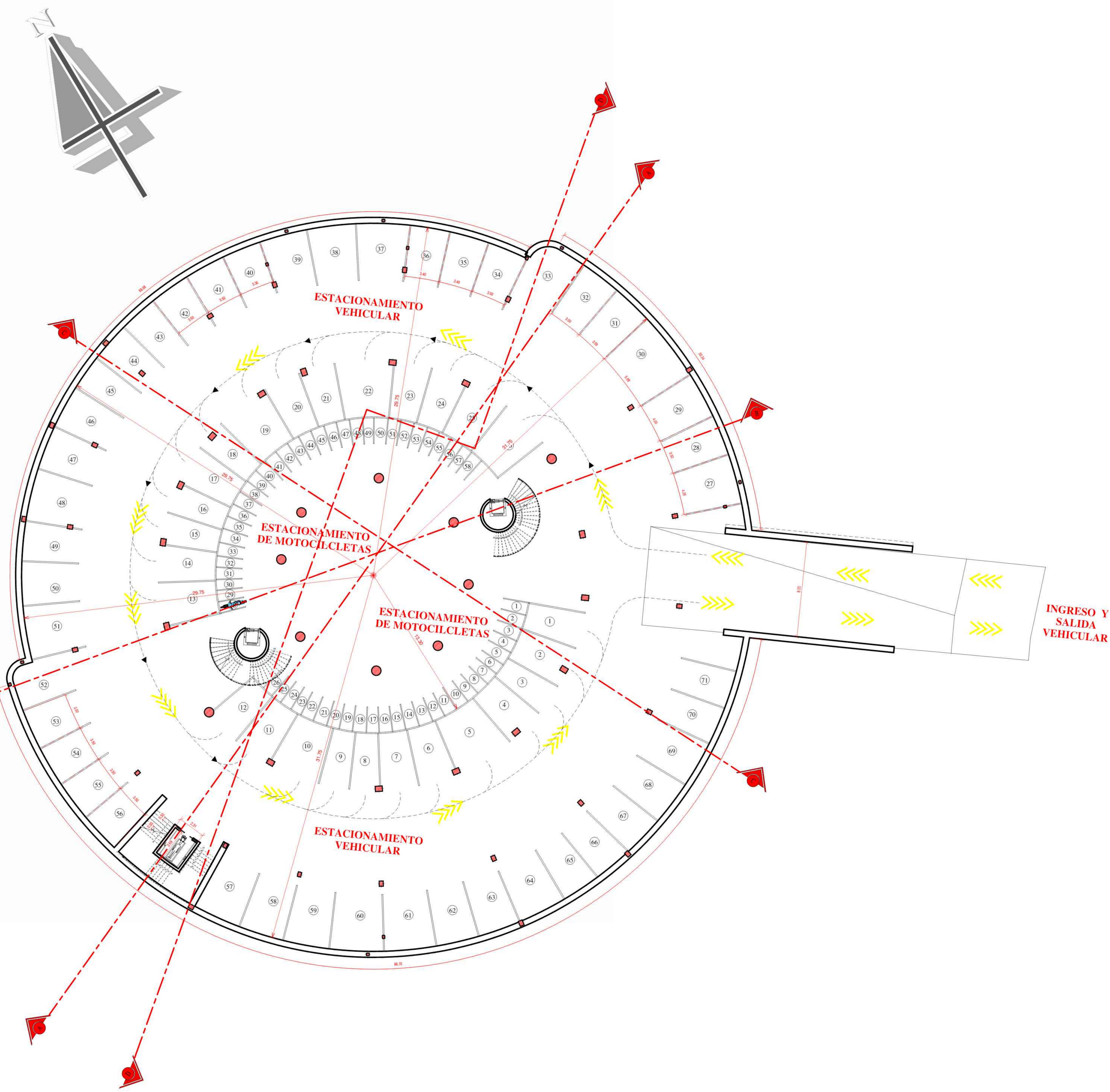
--PLANO DE SUBSUELO ACOTADO-- ESC:1:100
