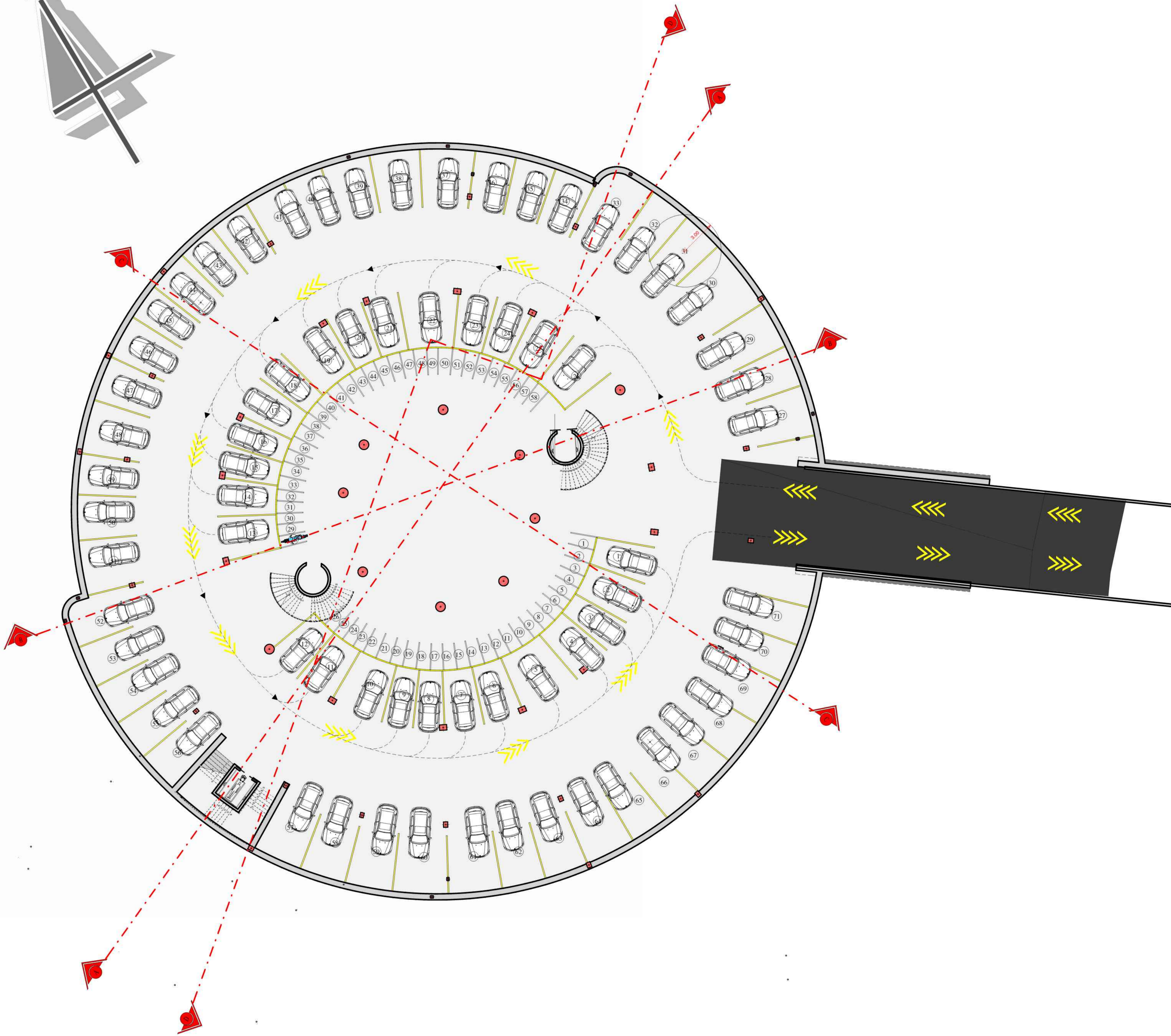
--PLANO DE SUBSUELO AMOBLADO-- ESC:1:100
