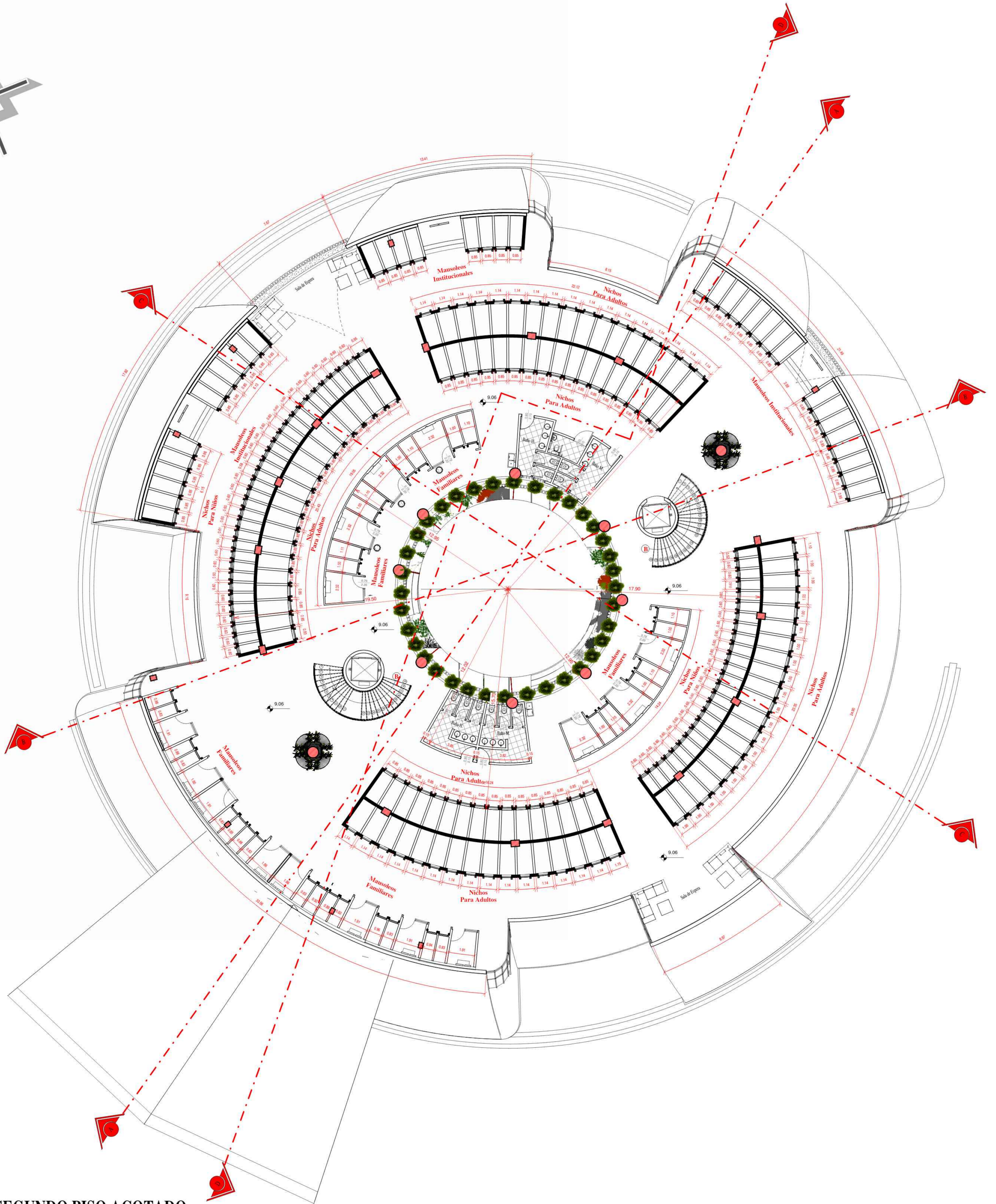
--PLANO DE SEGUNDO PISO ACOTADO-- ESC:1:100
