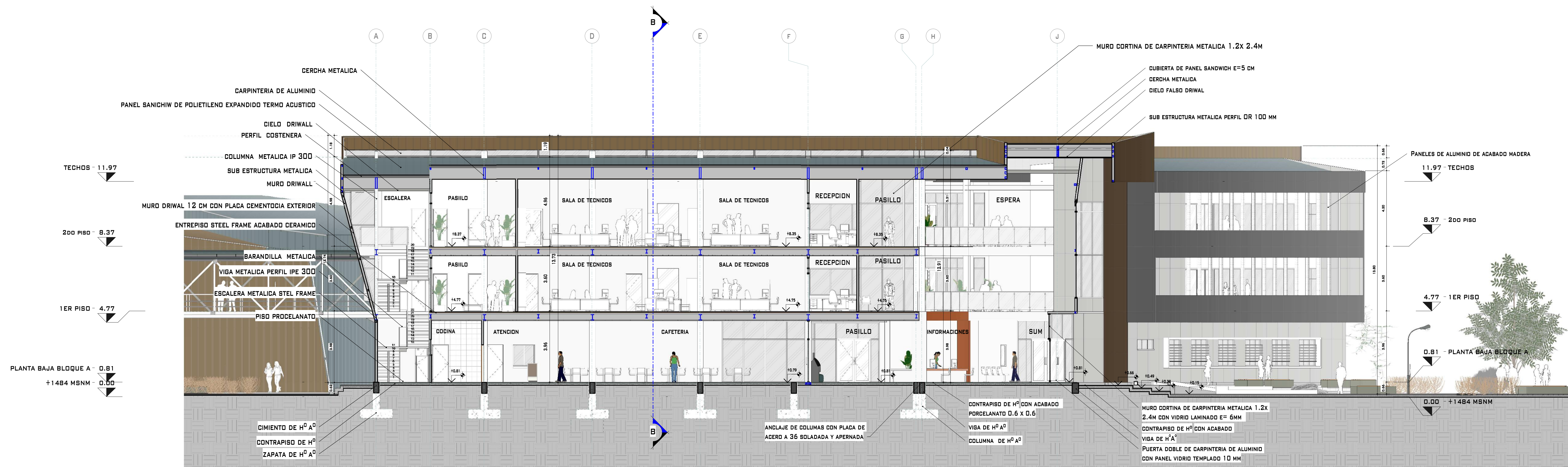
A BLOQUE A - CORTE LONGITUDINAL A-A 1 : 100
