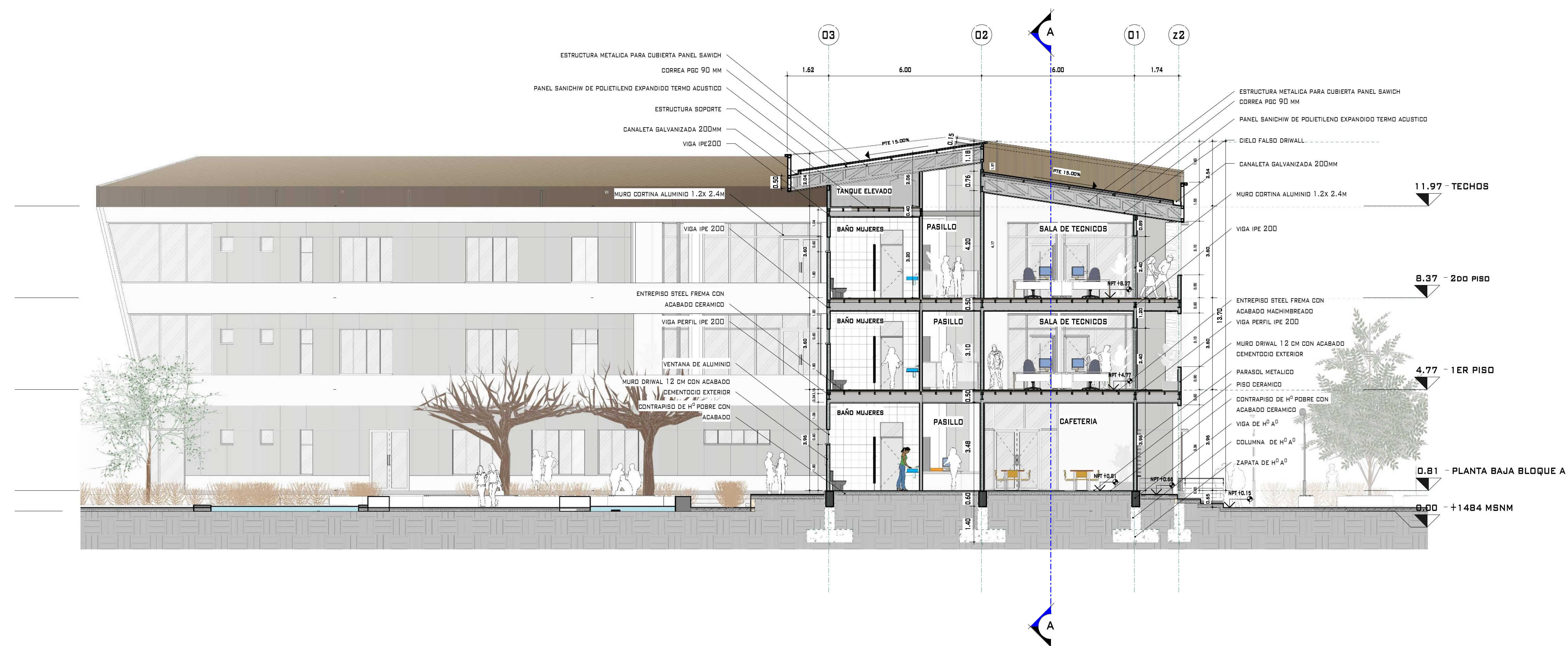
B BLOQUE A -CORTE TRANSVERSAL B- B 1 : 100
