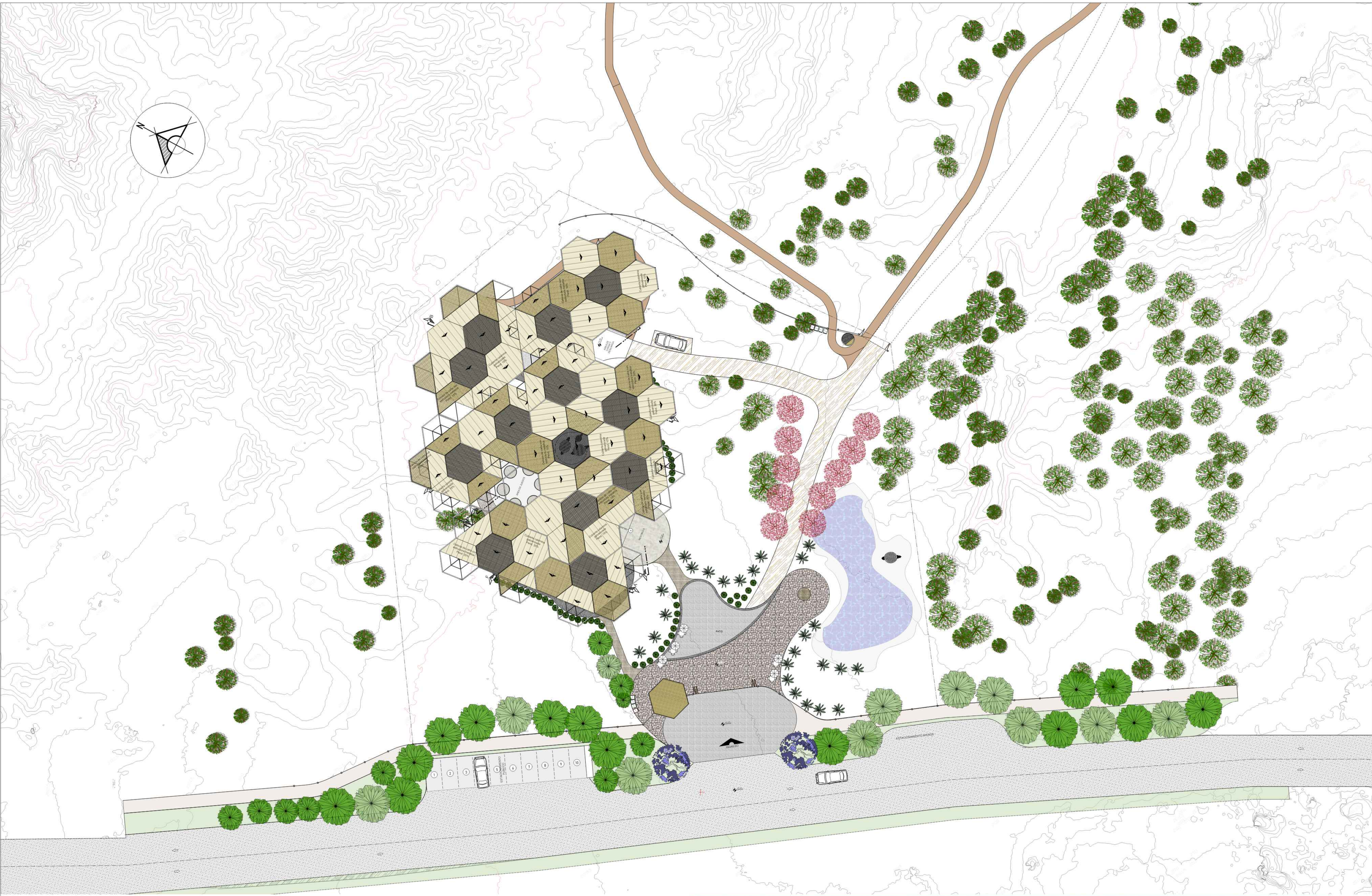
LAMINA DE SITIO Y TECHO ESC. 1:200
