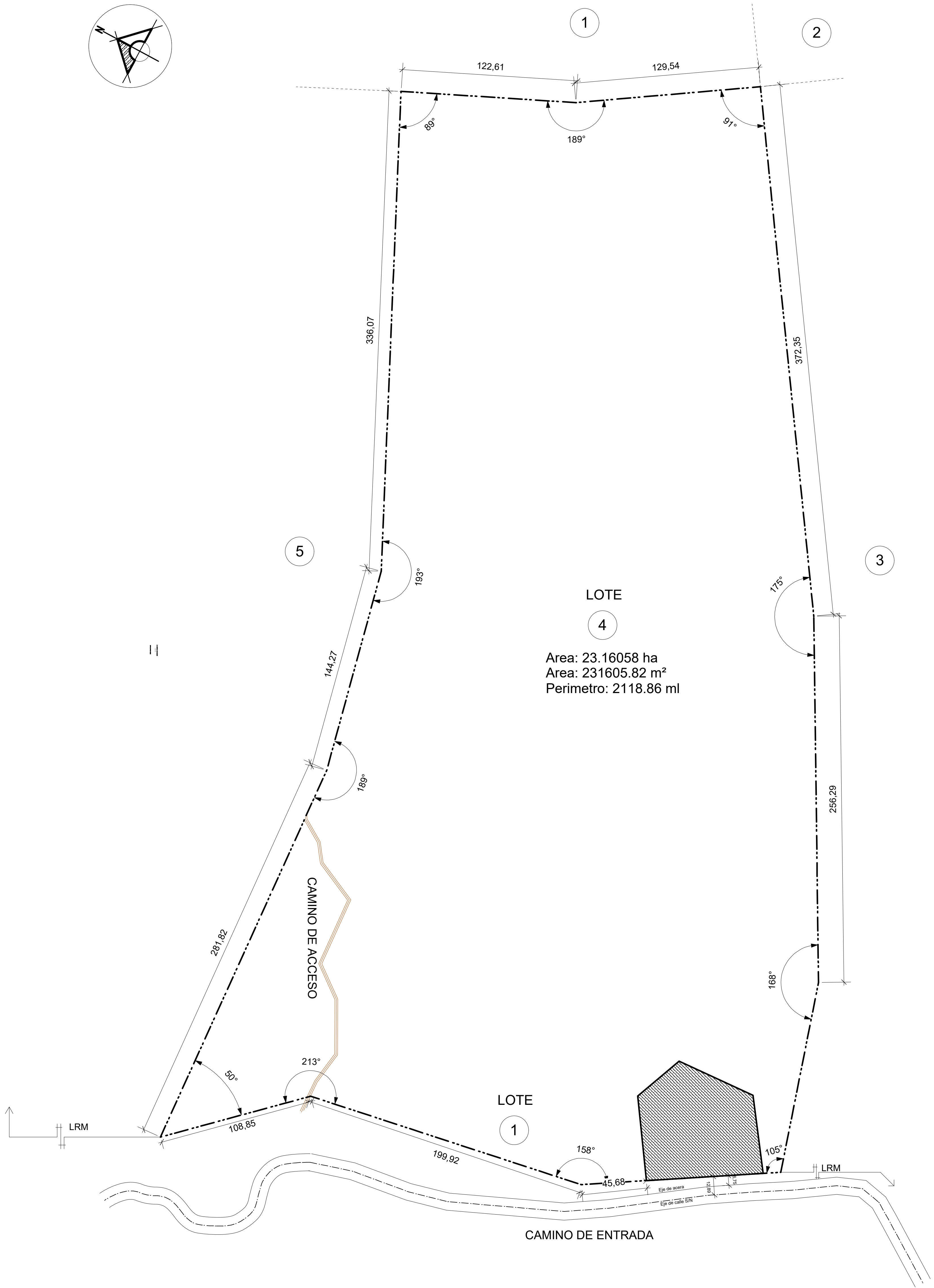
PLANO DE LOTE ESC. 1 : 1500
