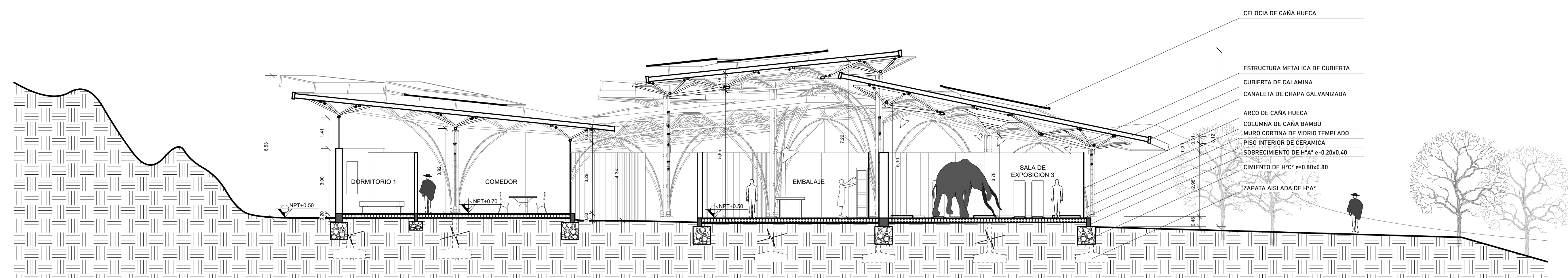
CORTE TRANSVERSAL " B-B "
