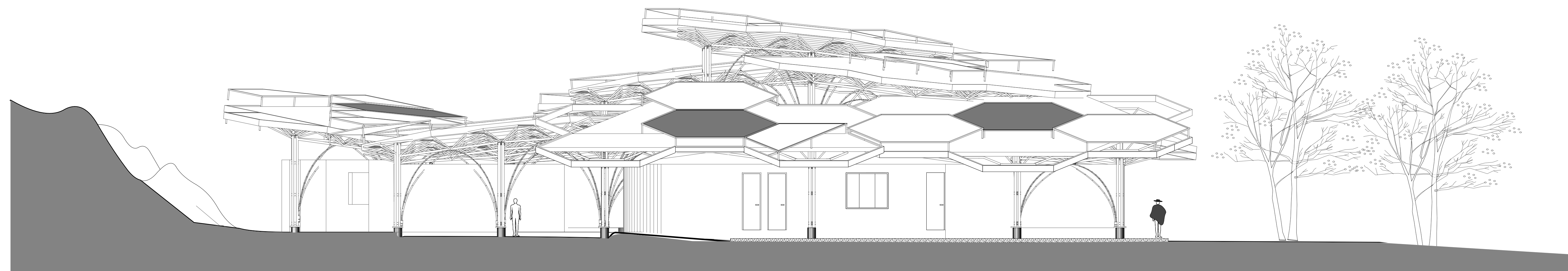
FACHADA LATERAL OESTE
