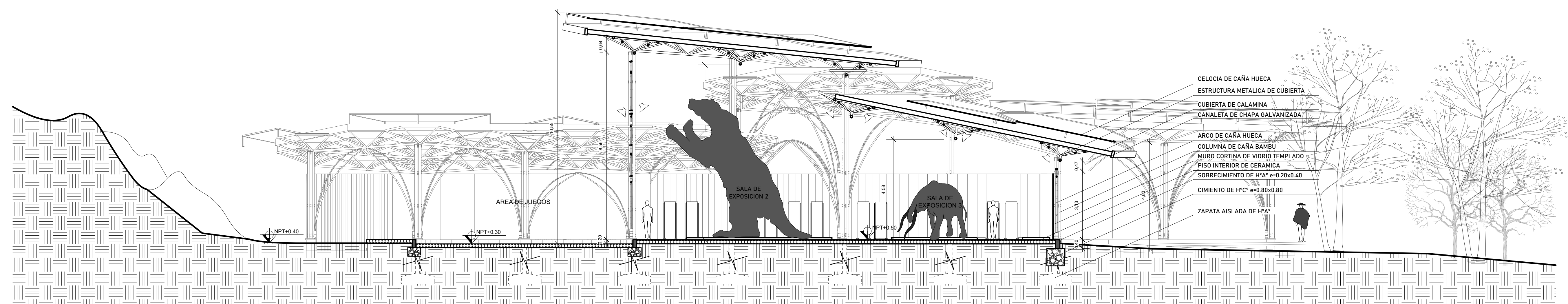
CORTE TRANSVERSAL " C-C "
