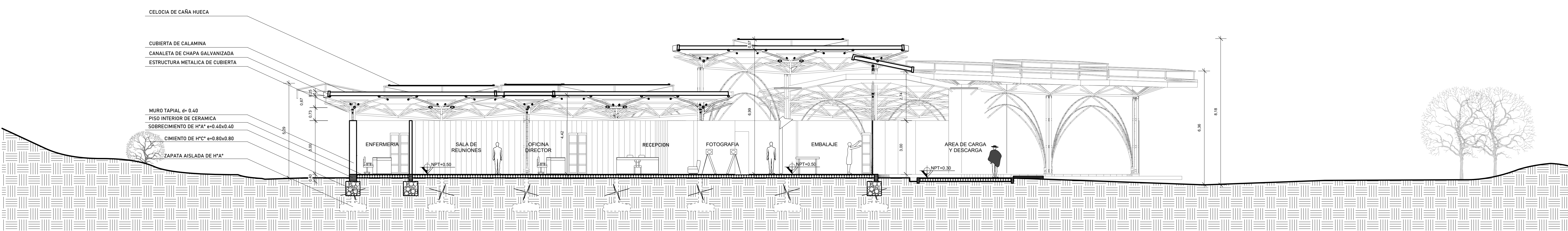
CORTE LONGITUDINAL "E-E"
