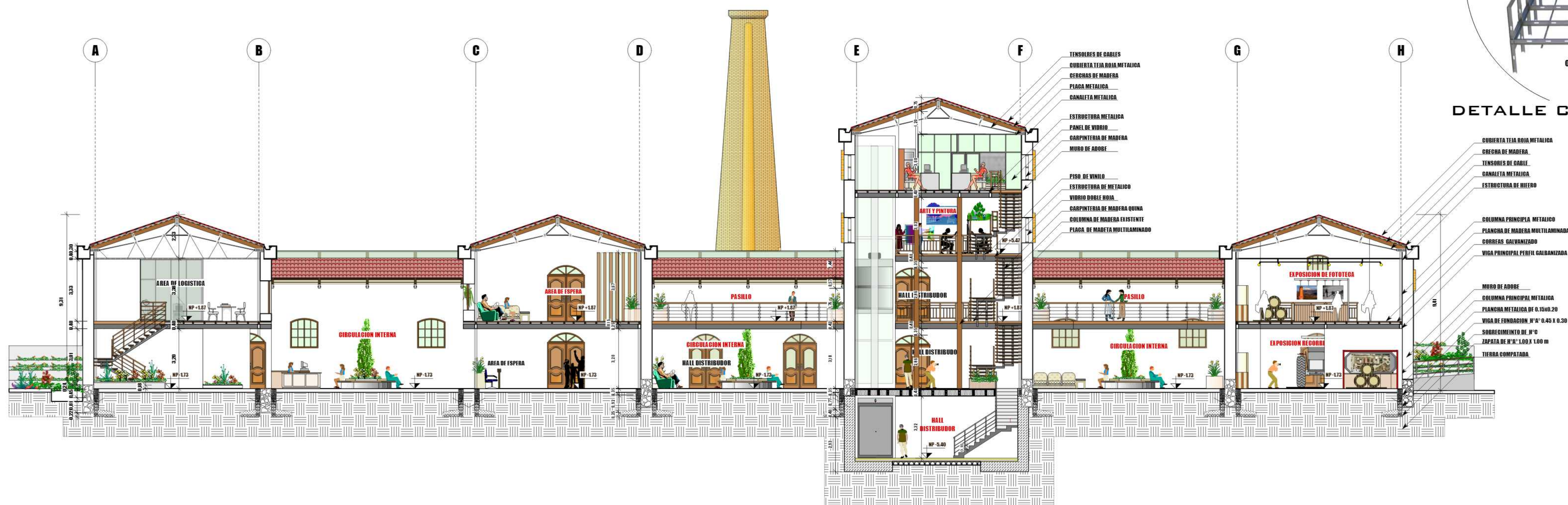
CORTE D - D
