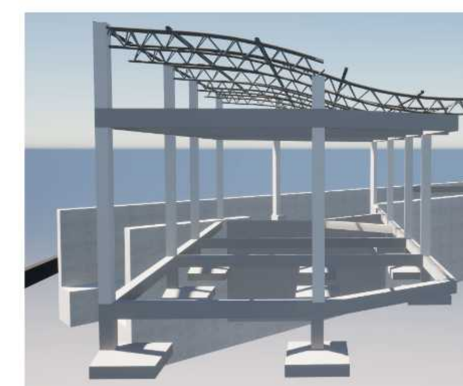
ESTRUCTURA DE H°A°
