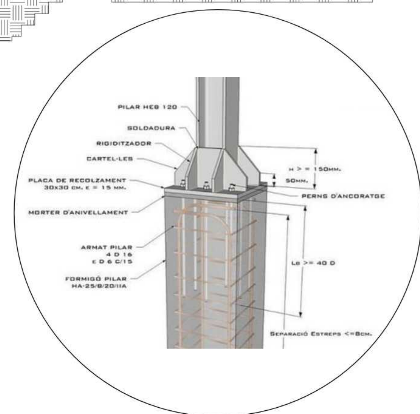
DETALLE CONSTRUCTIVO
