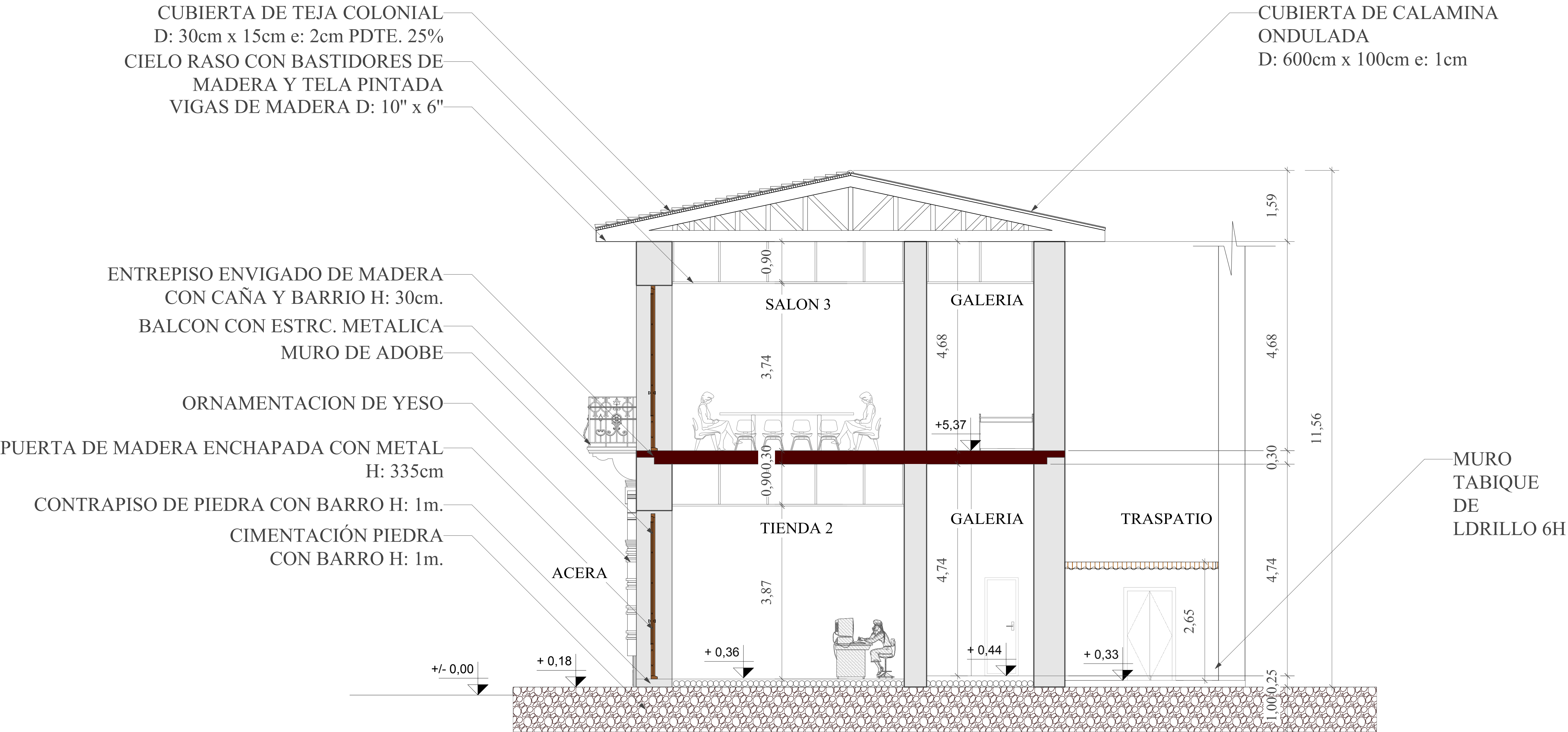
CORTE TRANSVERSAL B'- B" CASA NAVAJAS ACTUAL
