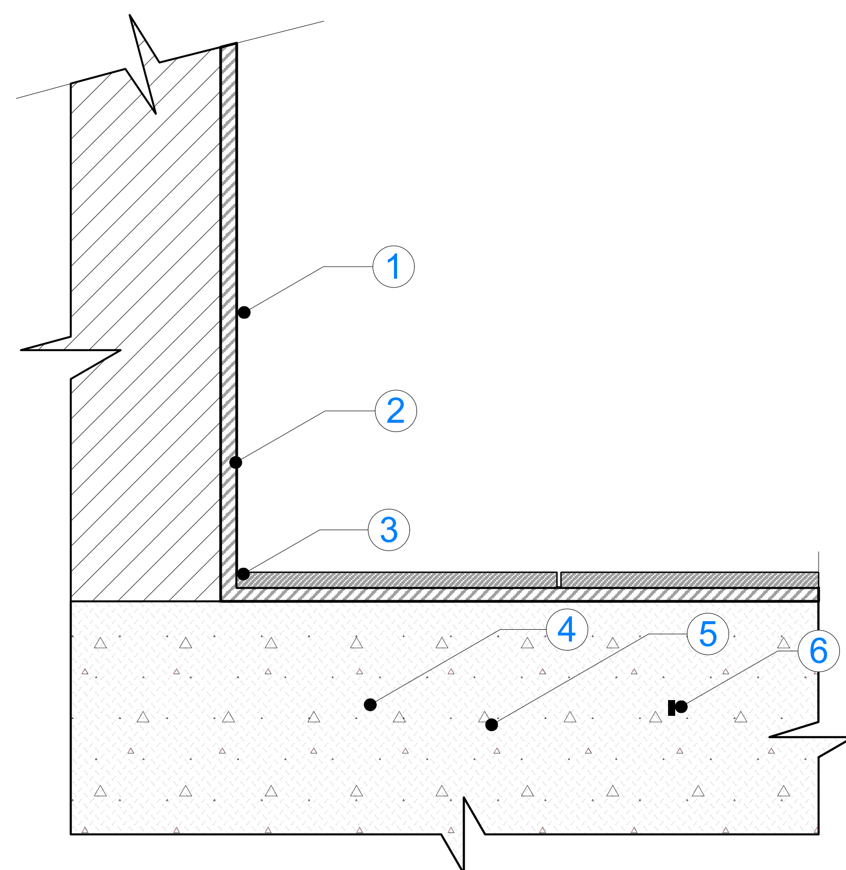
DETALLE: PISO DE PORCELANATO (ESC. 1:2)
