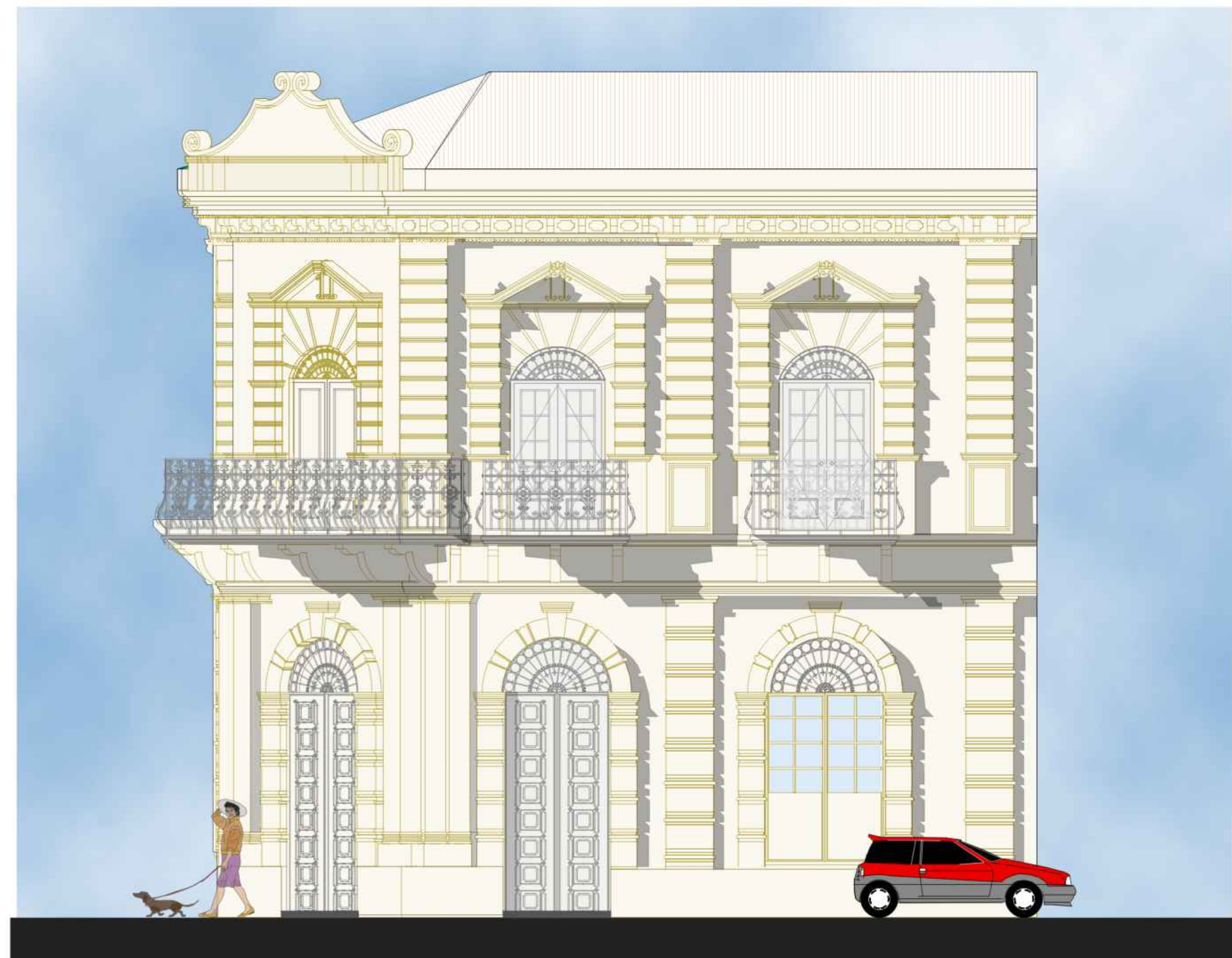
FACHADA TRANSVERSAL B'- B" CASA NAVAJAS ACTUAL
