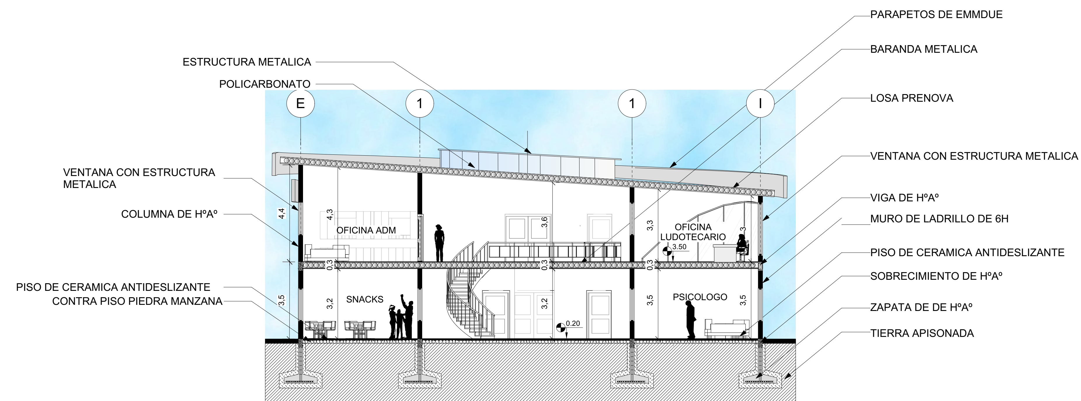
CORTE A-A ESC 1:100
