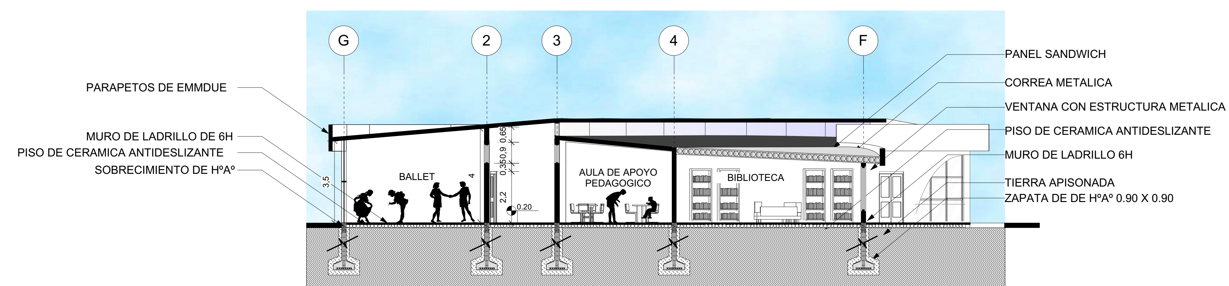
CORTE C-C ESC 1:100
