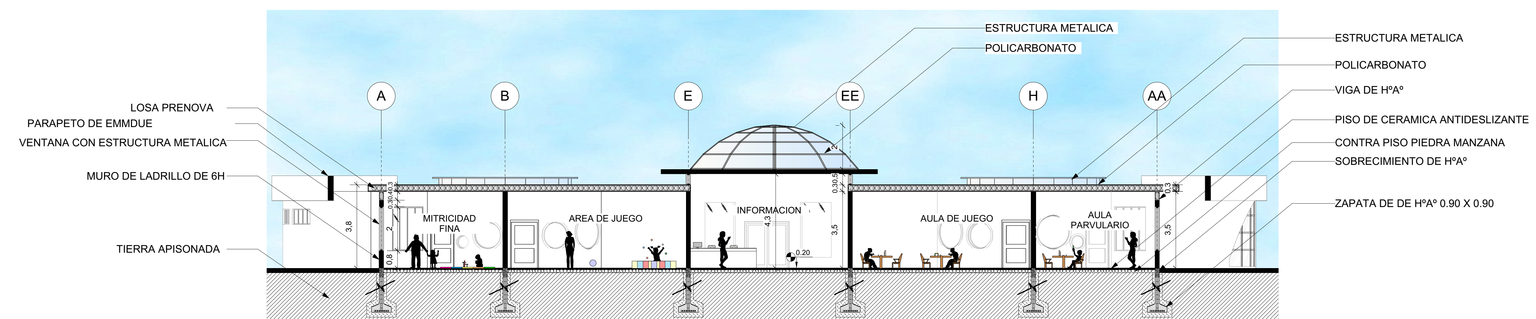
CORTE D-D ESC 1:100
