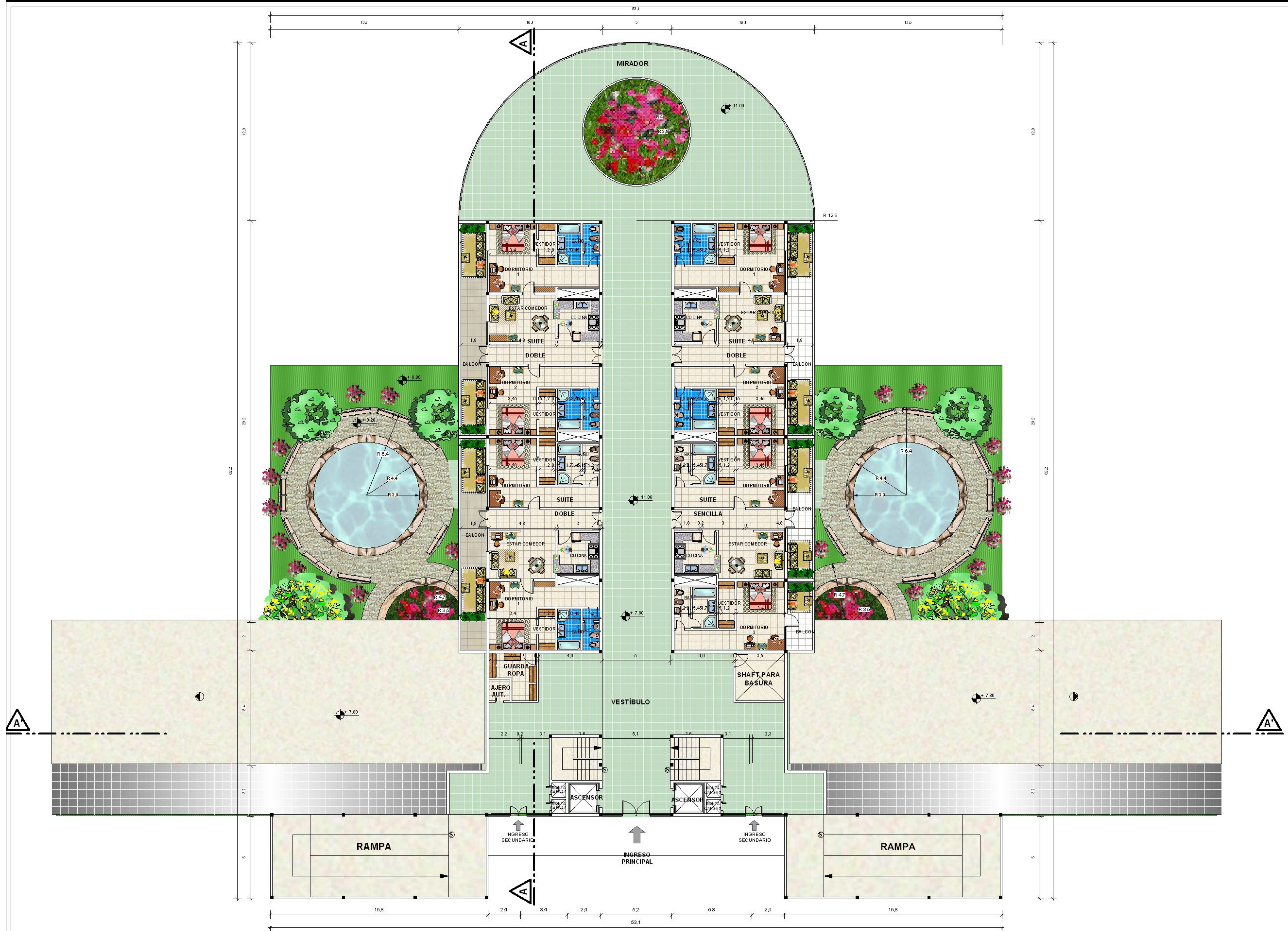
PLANTA TIPO PISO 4 AREA DE HOSPEDAJE HOTEL TURISTICO**** ESC. 1:100
