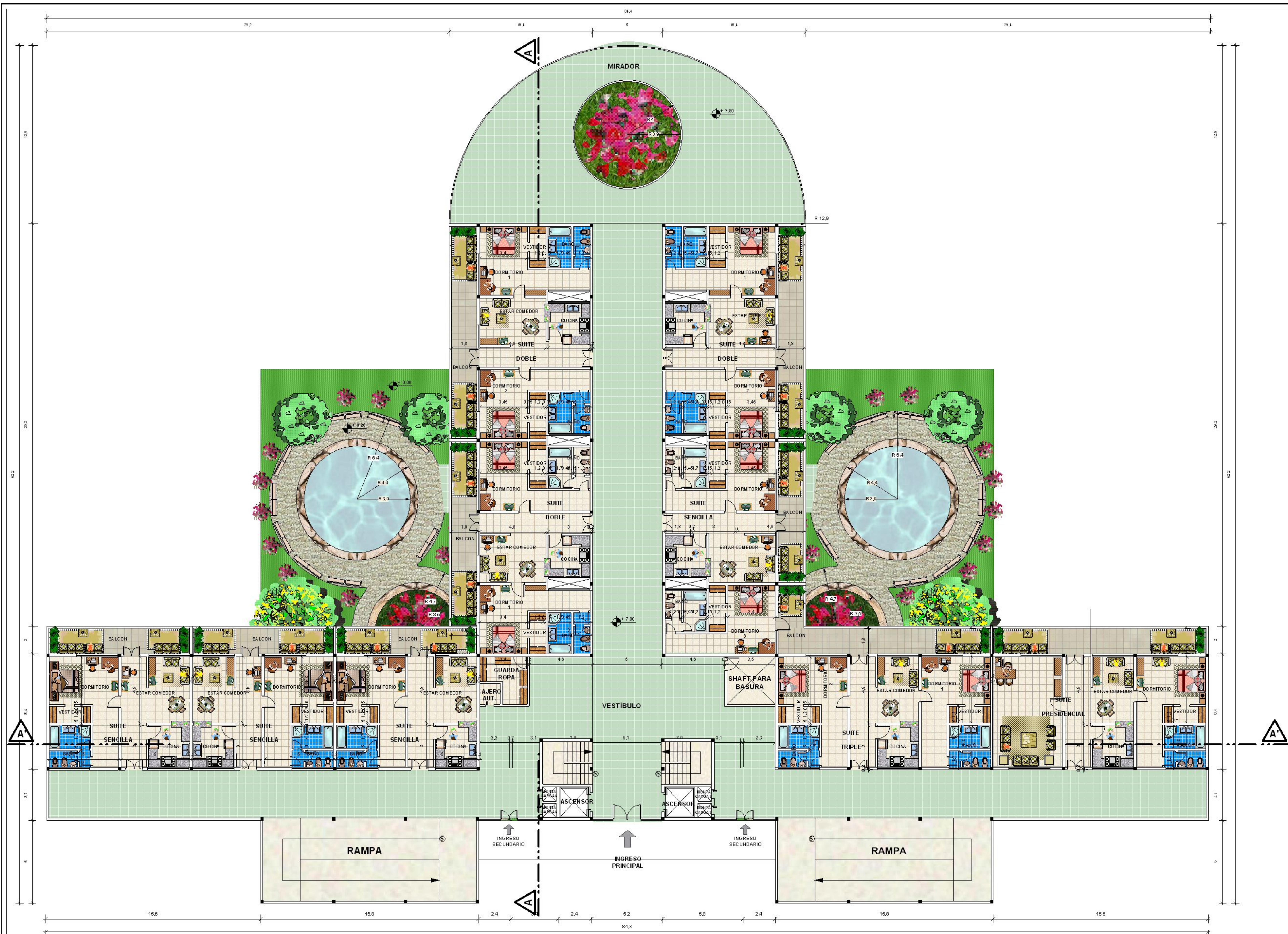
PLANTA TIPO PISO 2, 3, AREA DE HOSPEDAJE HOTEL TURISTICO**** ESC. 1:100
