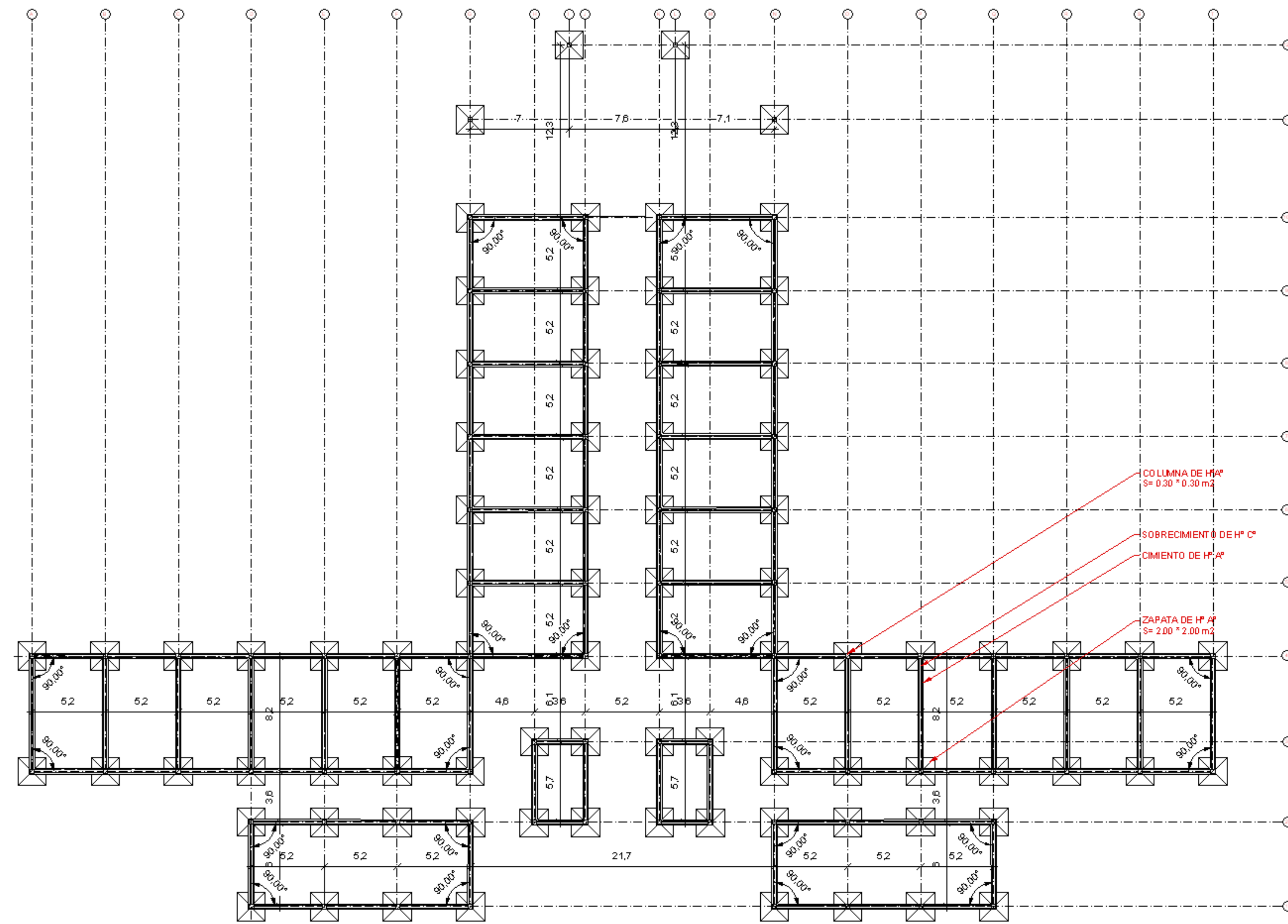
CIMENTOS, SOBRECIMENTOS Y FUNDACIONES DE AREA DE HOSPEDAJE HOTEL TURISTICO**** ESC. 1:200
