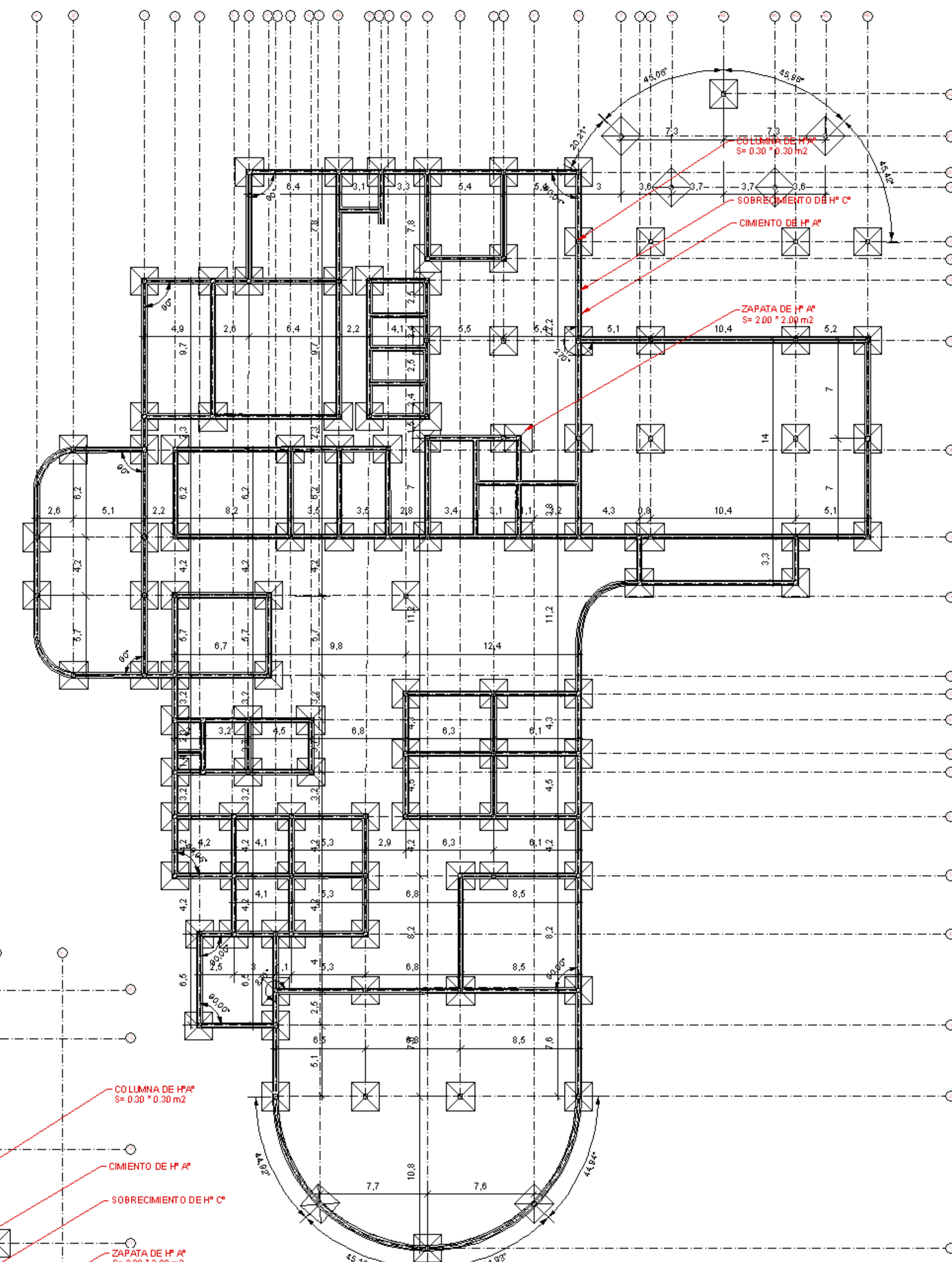
CIMENTOS, SOBRECIMENTOS Y FUNDACIONES DE AREA ADMINISTRACION Y SERVICIOS HOTEL TURISTICO**** ESC. 1:200
