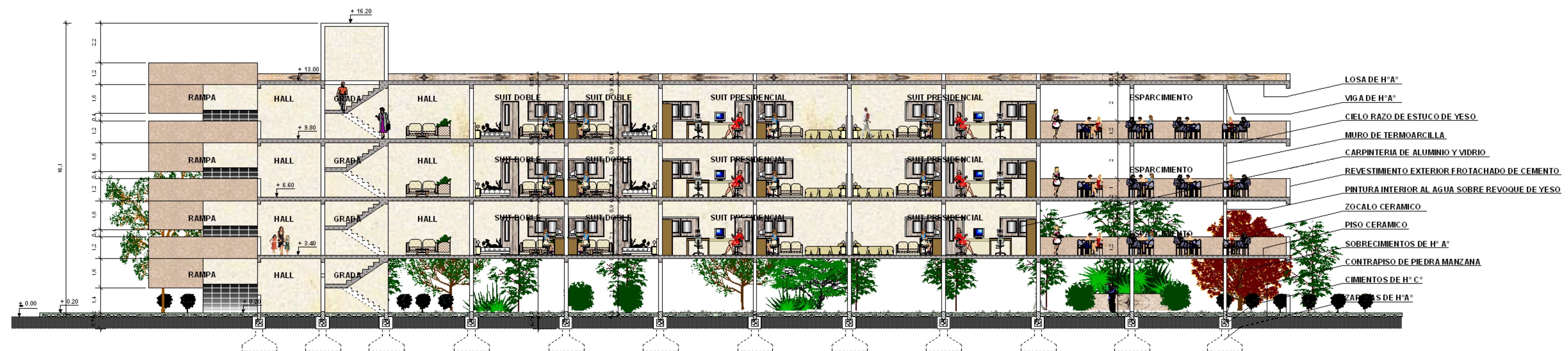
CORTE A'-A' HOTEL TURISTICO****
