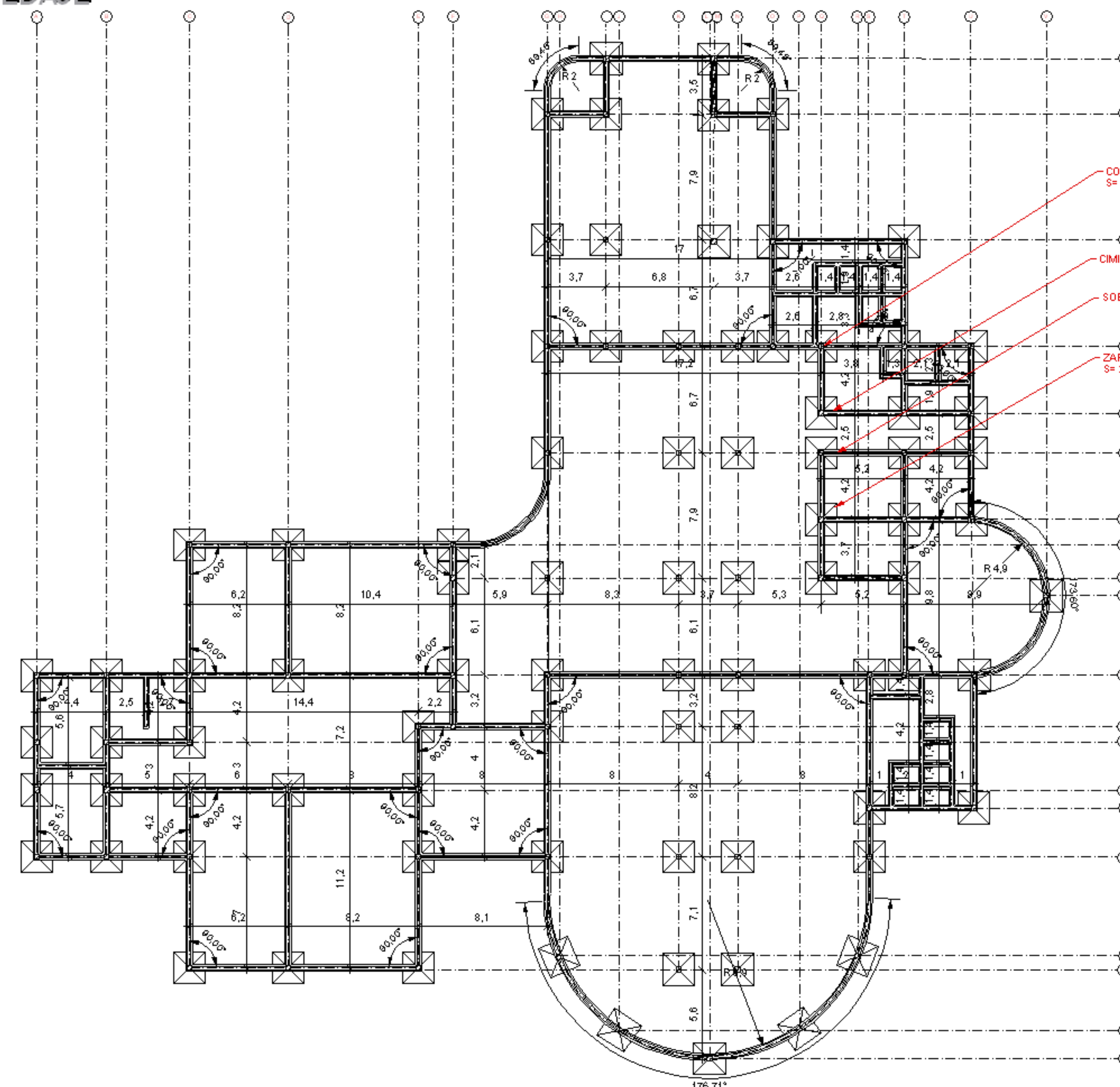
CIMENTOS, SOBRECIMENTOS Y FUNDACIONES DE AREAS: RECREACION, DEPORTES Y ESPECIALES HOTEL TURISTICO**** ESC. 1:100
