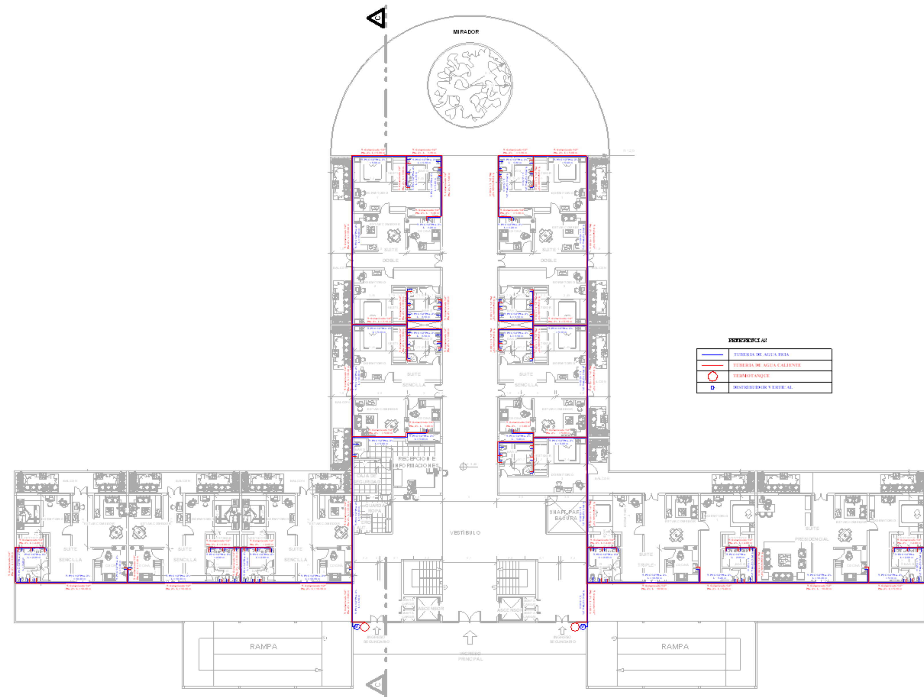
INSTALACIÓN DE AGUA PLANTA PISO 1 AREA DE HOSPEDAJE HOTEL TURISTICO**** ESC. 1:100
