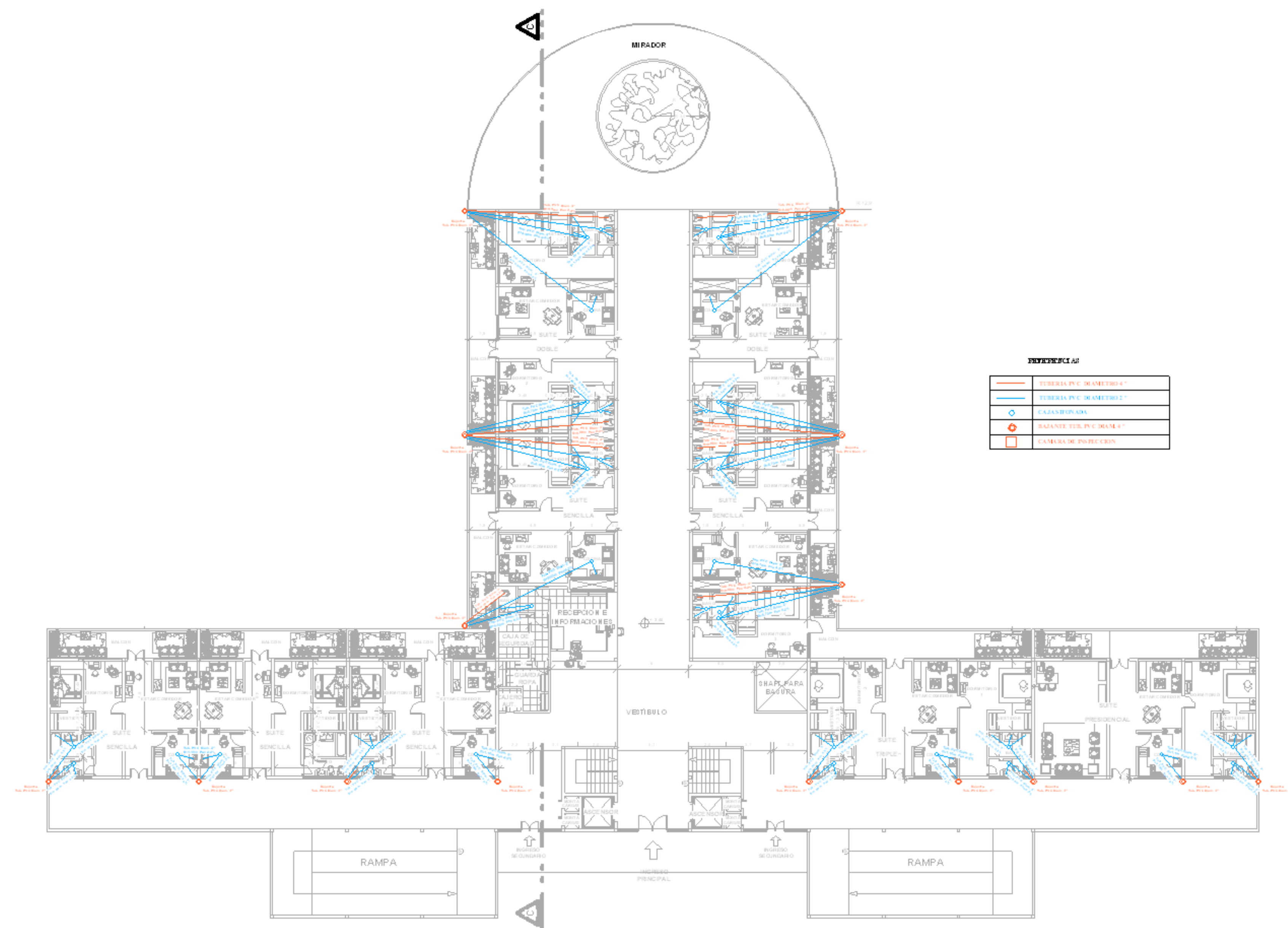
INSTALACIÓN SANITARIA PLANTA PISO 1-4 AREA DE HOSPEDAJE HOTEL TURISTICO**** ESC. 1:100
