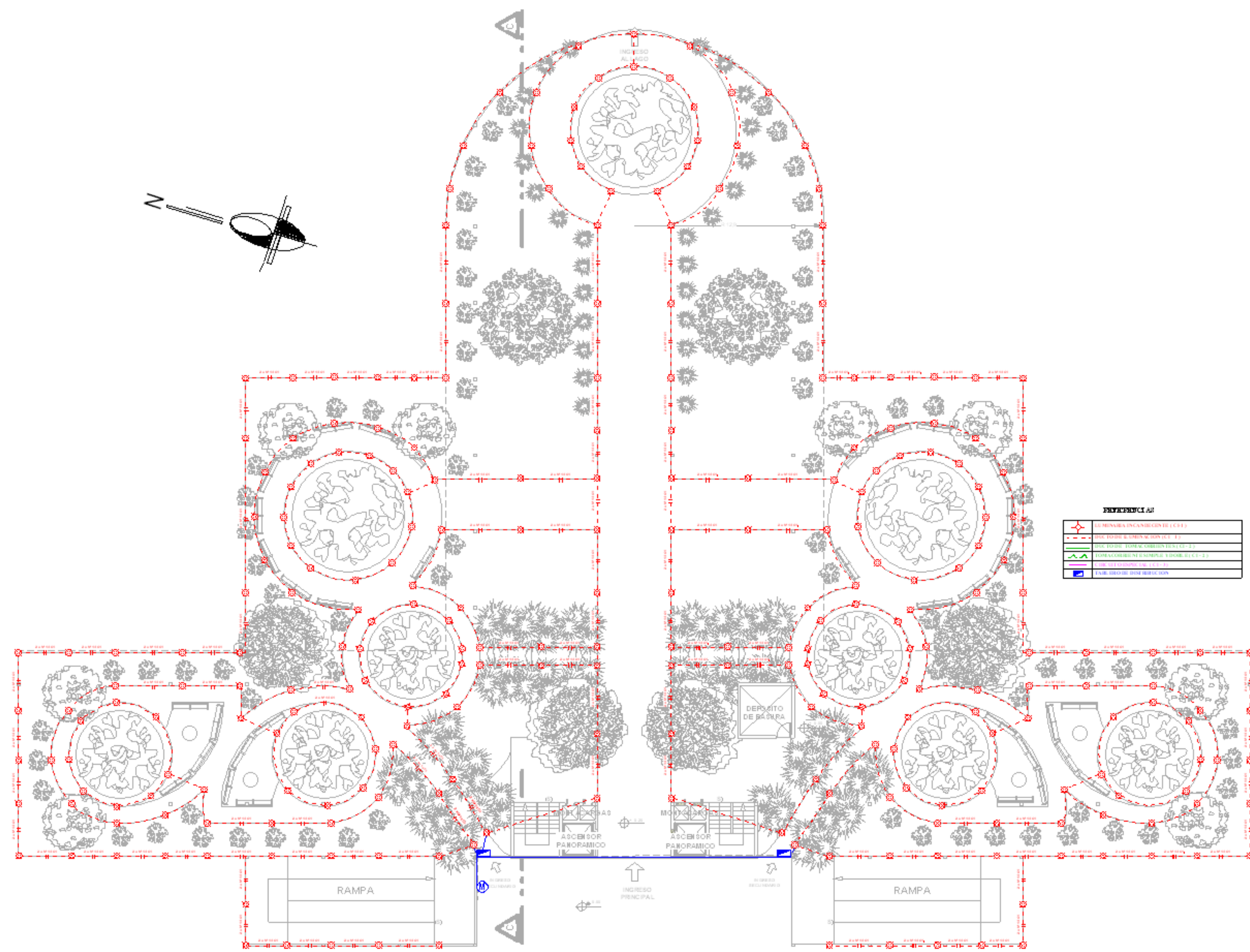
INSTALACION ELECTRICA PLANTA BAJA AREA DE HOSPEDAJE HOTEL TURISTICO**** ESC. 1:200
