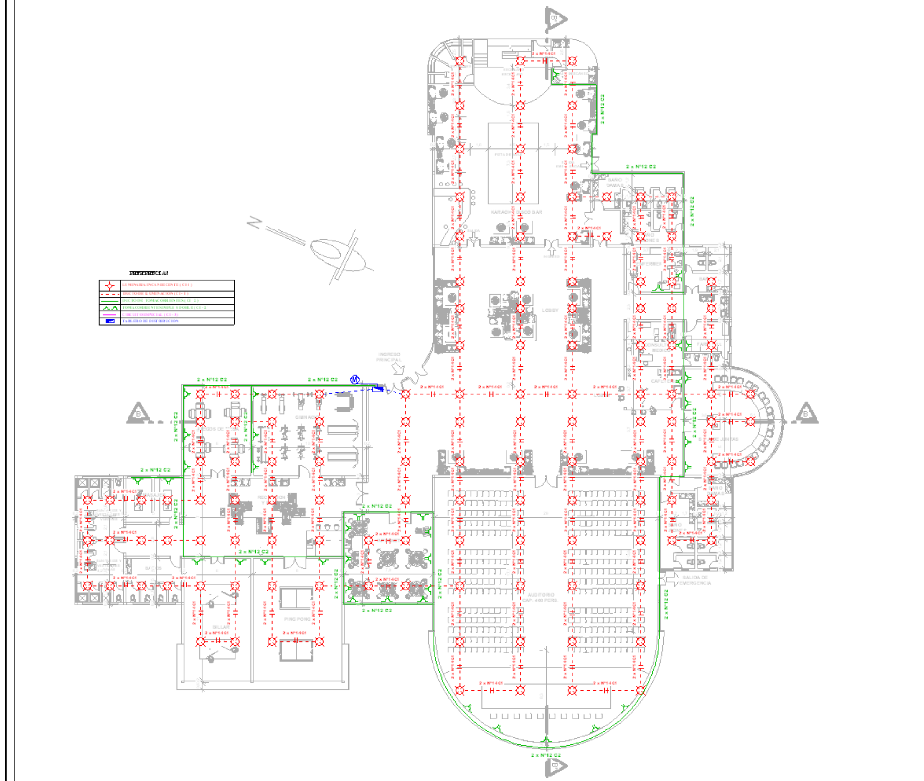
INSTALACION ELECTRICA DE AREA RECREACION. DEPORTES Y ESPECIALES HOTEL TURISTICO**** ESC. 1:200
