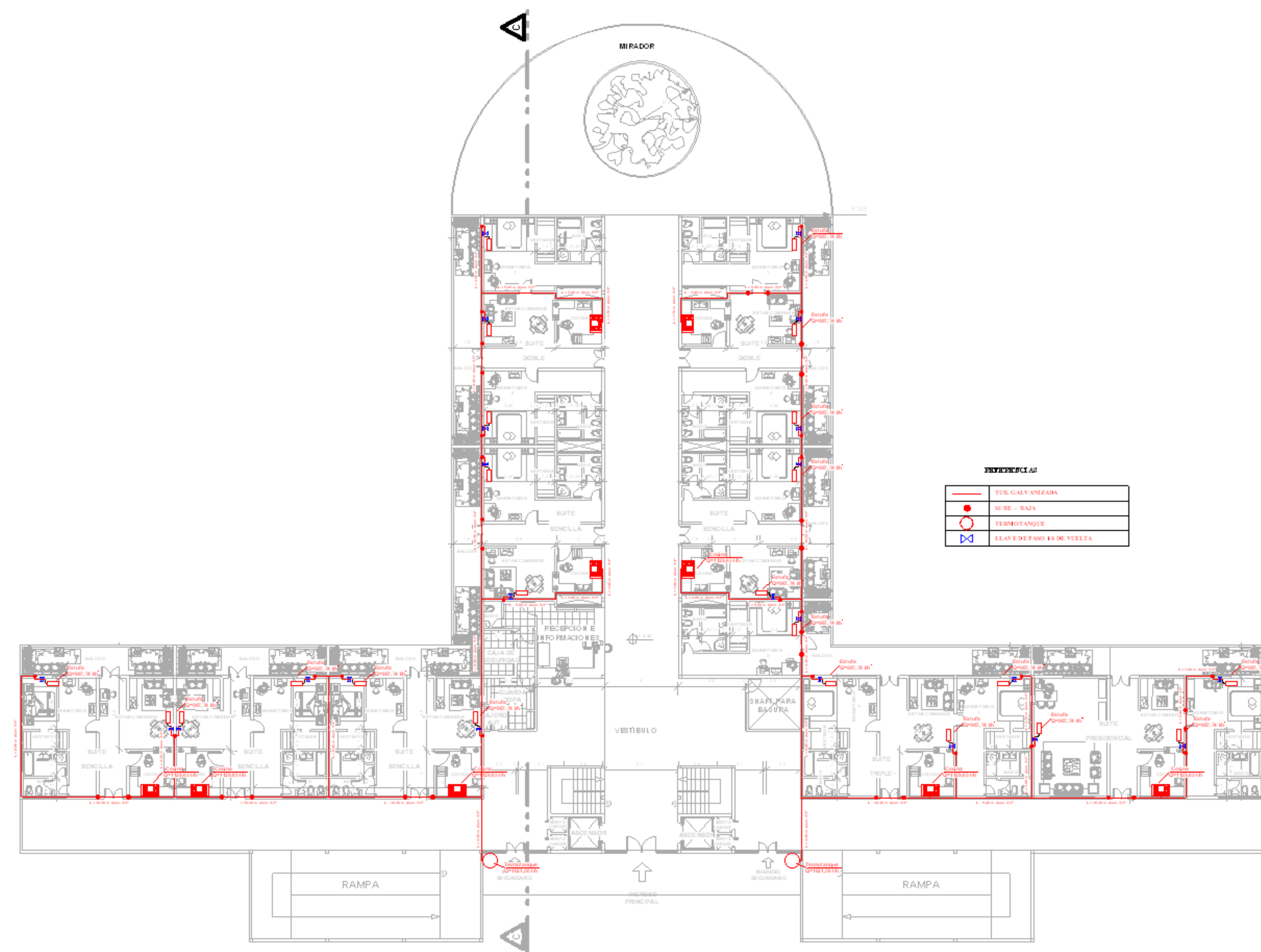
INSTALACIÓN DE GAS PLANTA PISO 1-4 AREA DE HOSPEDAJE HOTEL TURISTICO**** ESC. 1:100
