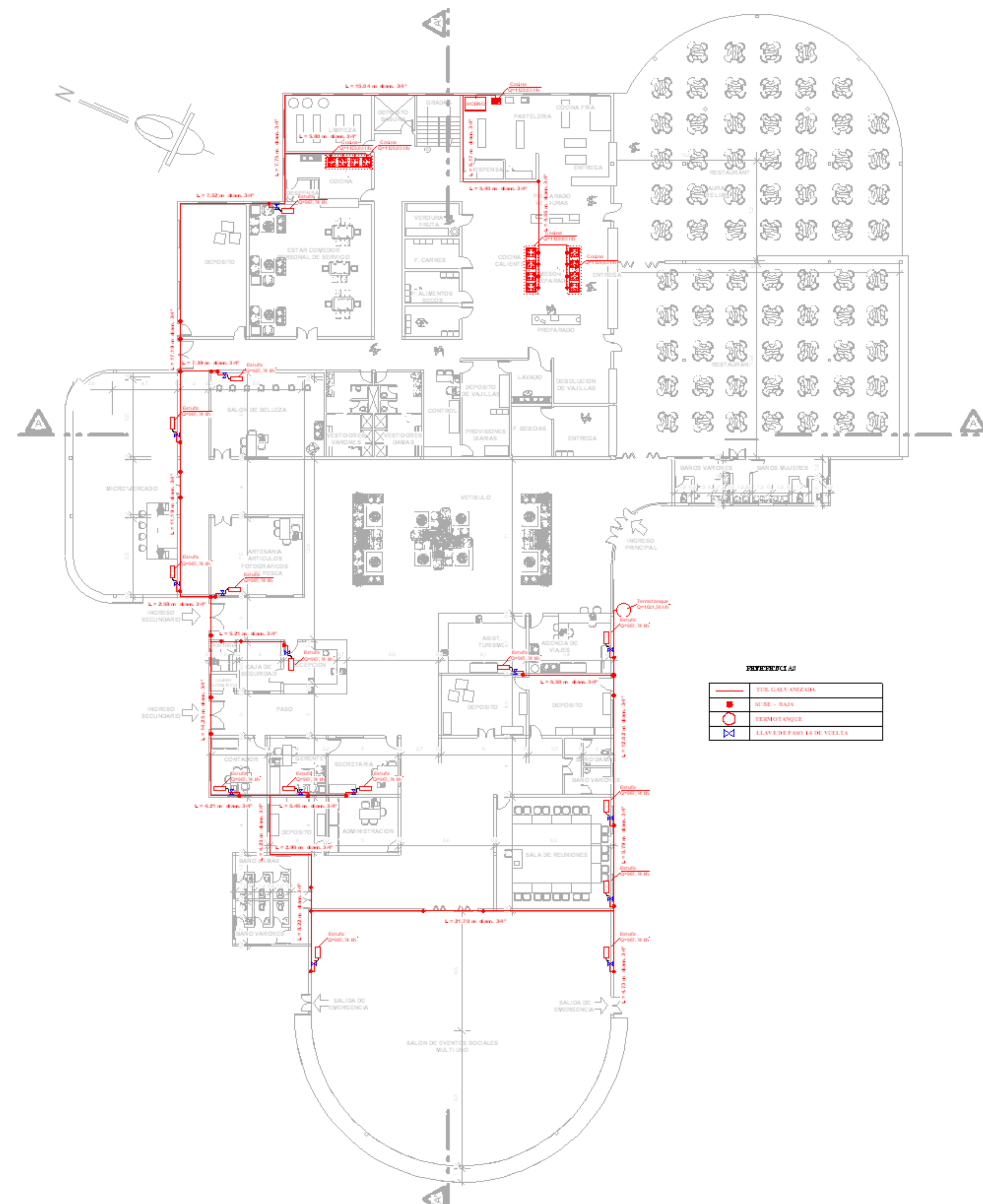
INSTALACION DE GAS AREA ADMIN ISTRATIVA Y SERVICIO HOTEL TURISTICO**** ESC. 1:200
