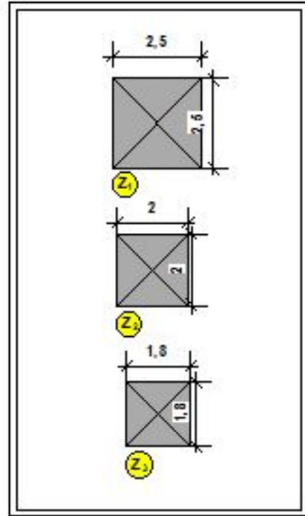
DETALLE ZAPATA 1 Esc. 1:50
