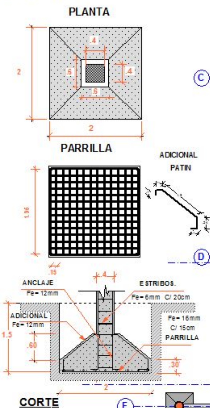
DETALLE ZAPATA 1 Esc. 1:50
