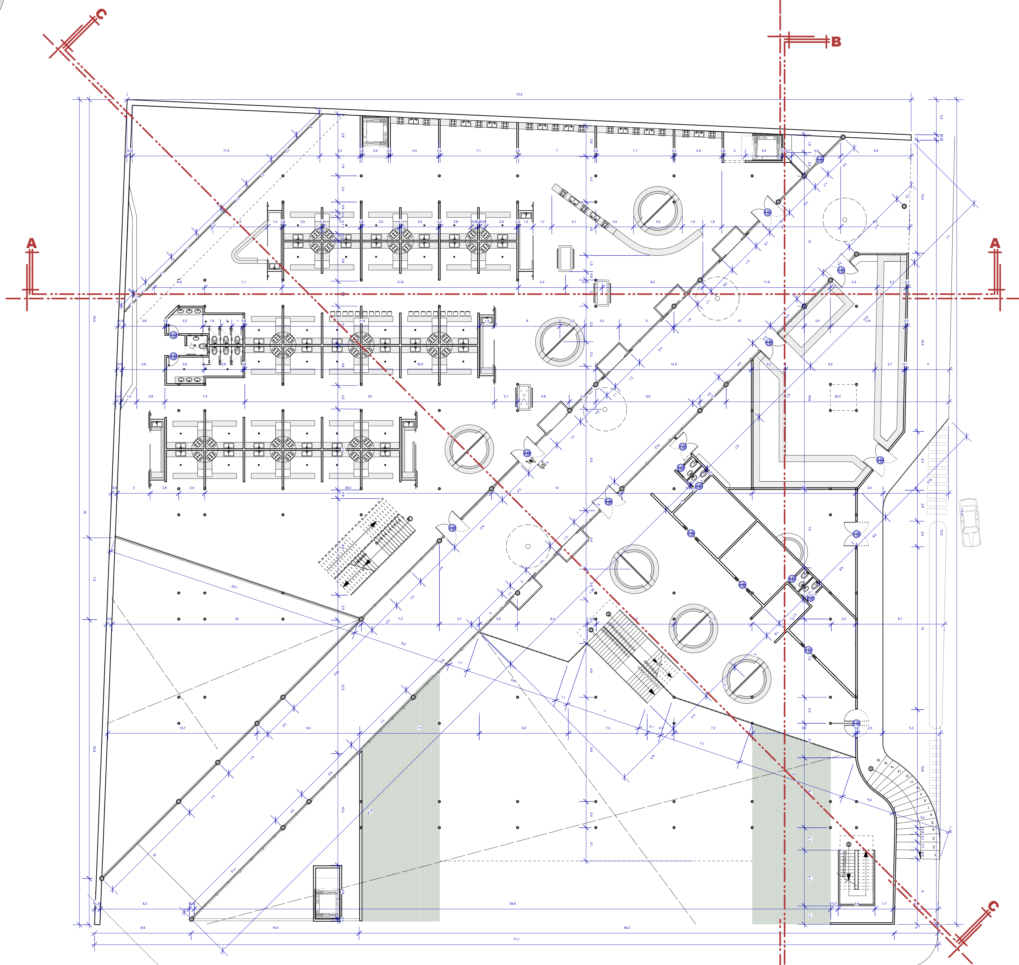
PLANTA PEATONAL (ACOTADA)
