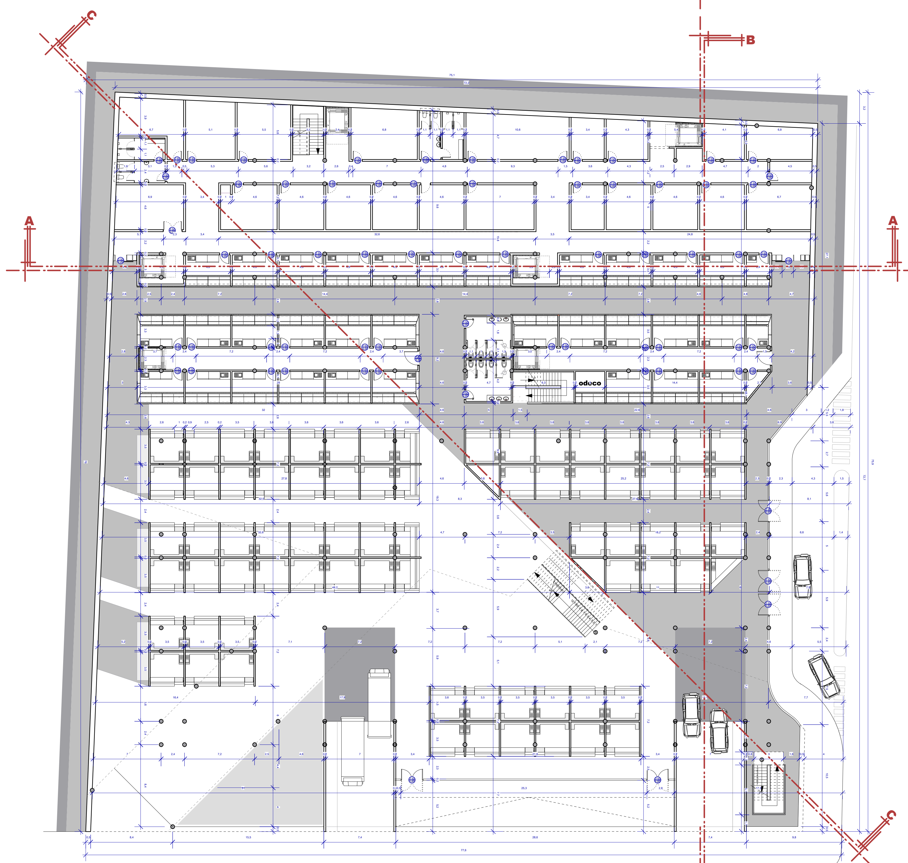
PLANTA SUB-SOTANO (ACOTADA)
