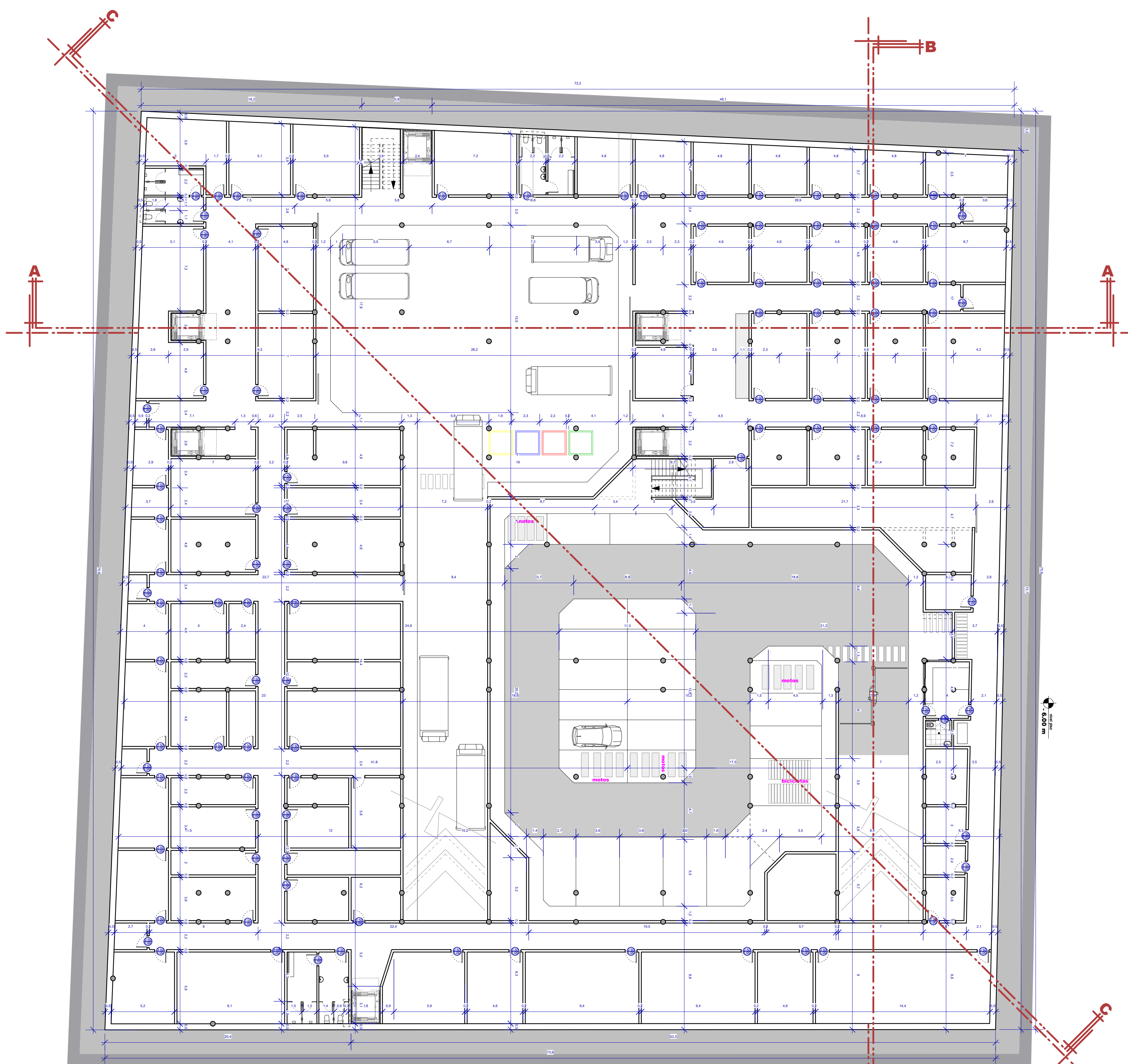
PLANTA SOTANO (ACOTADA)
