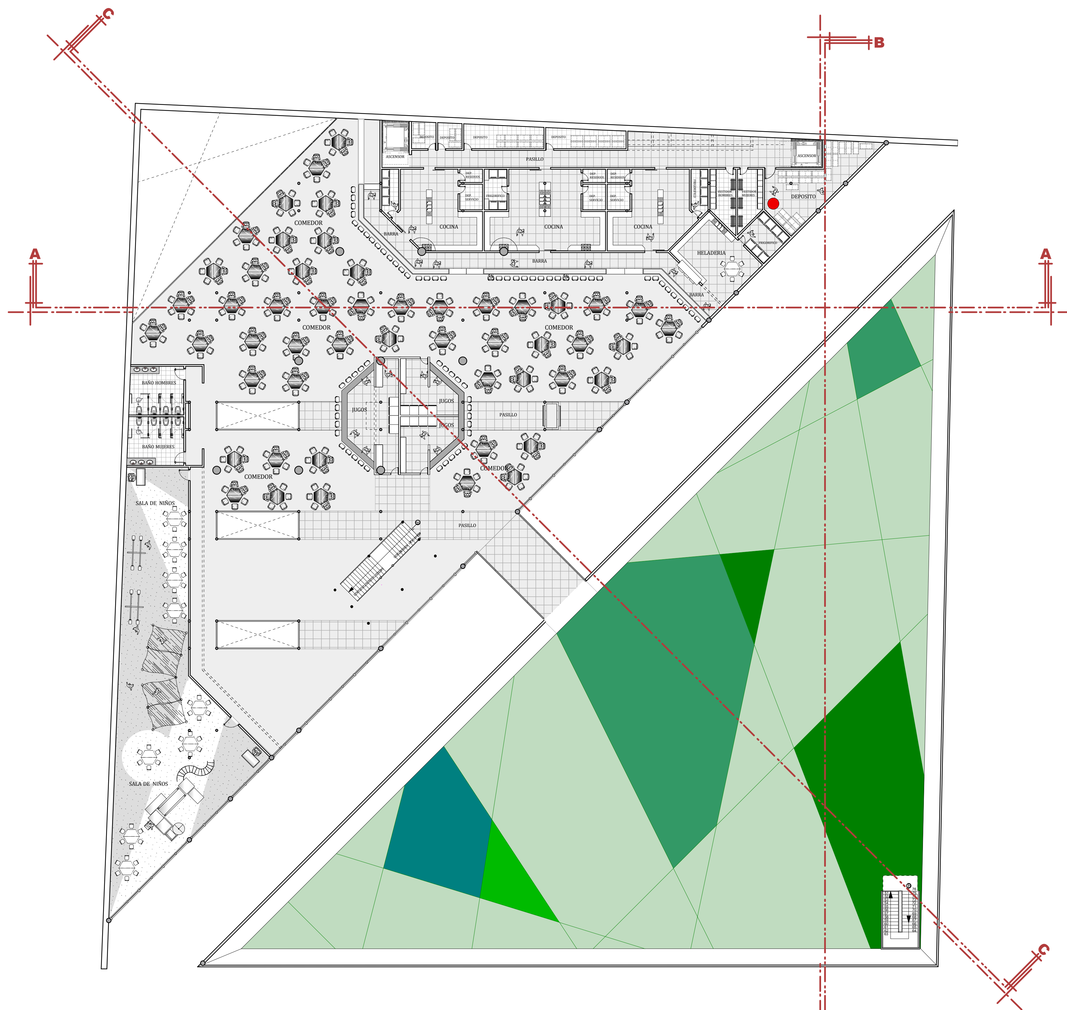
PLANTA 2do. PISO (EQUIPADA)
