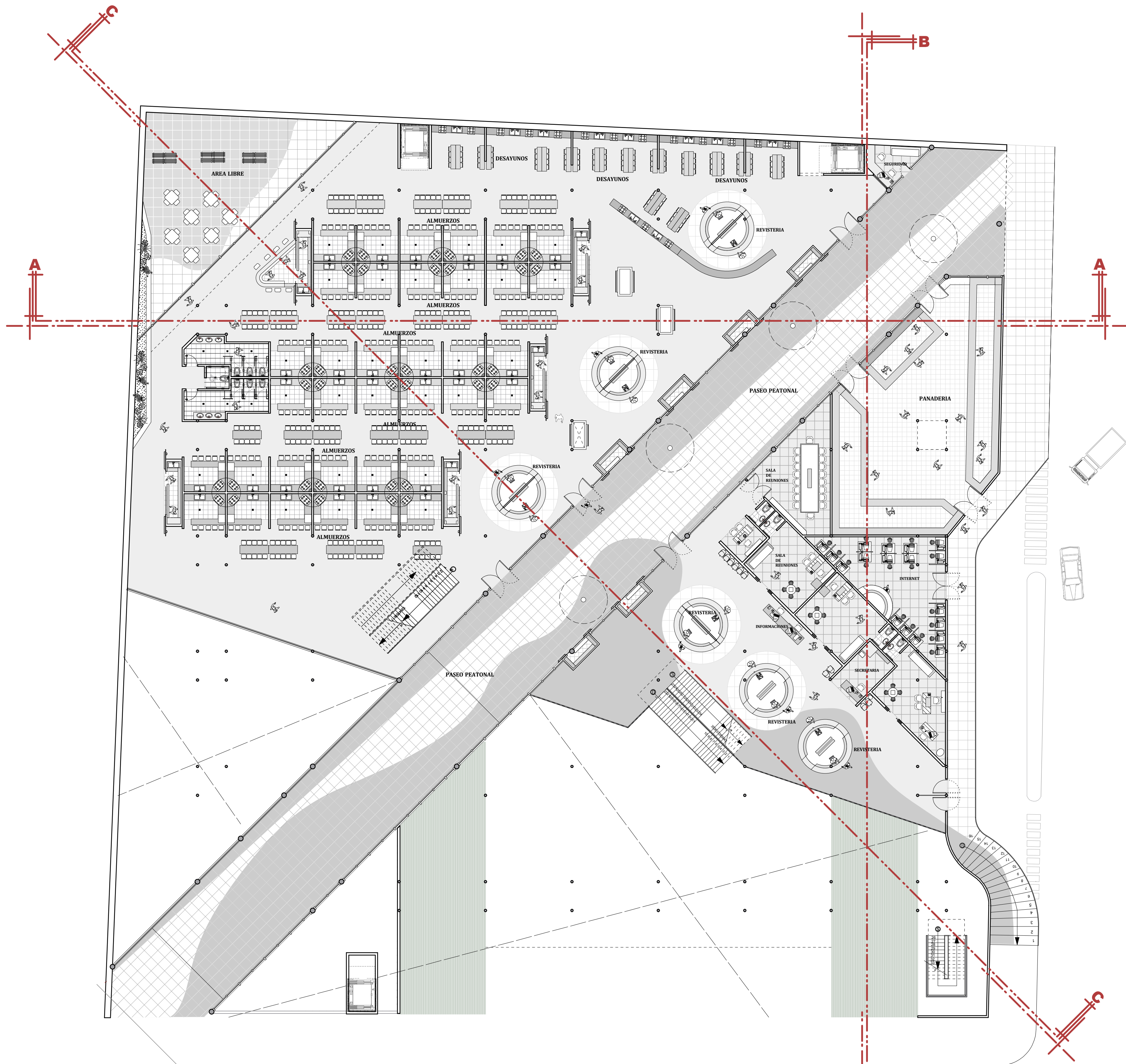
PLANTA PETONAL (EQUIPADA)
