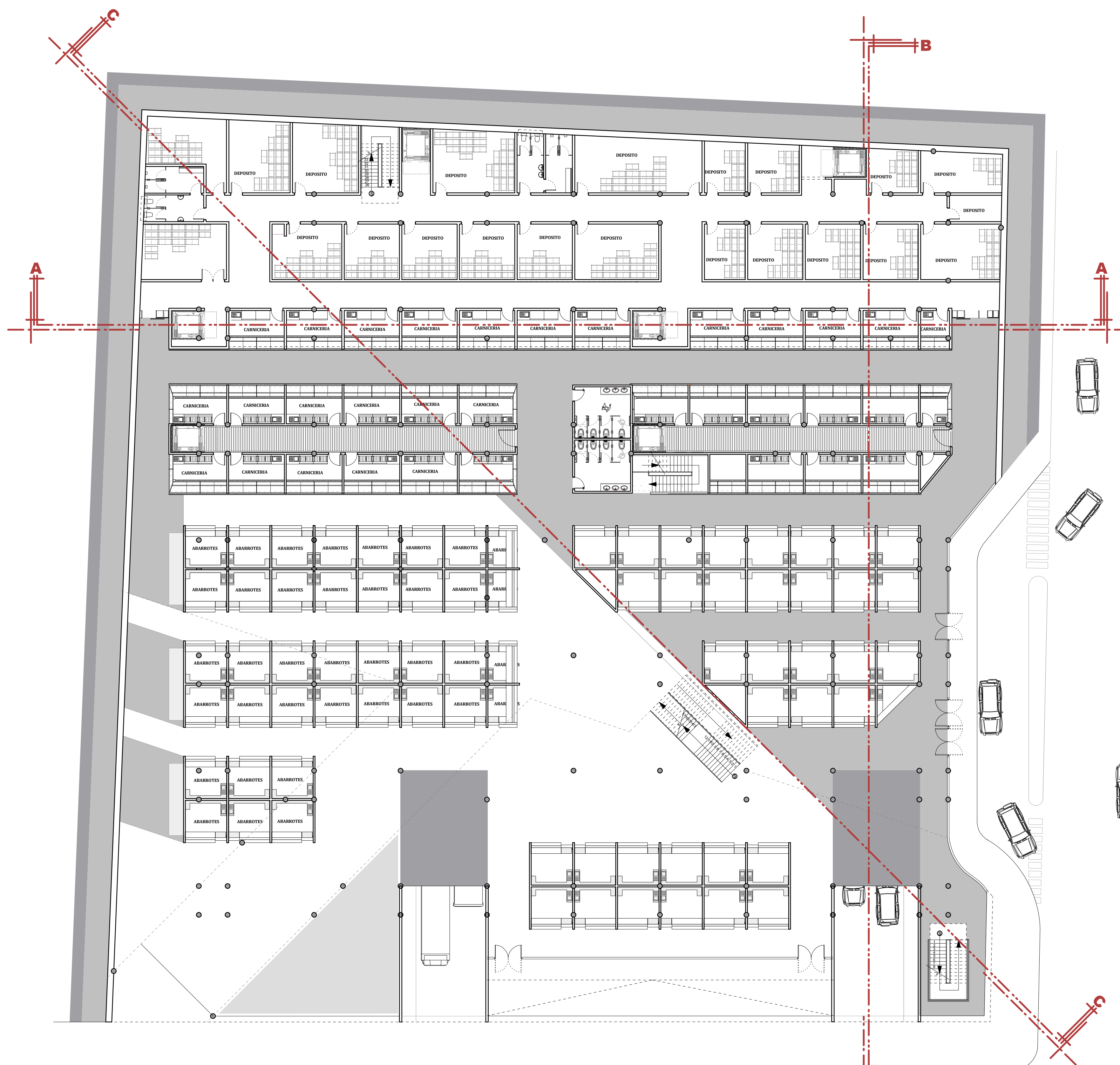
PLANTA SUB-SOTANO (EQUIPADA)
