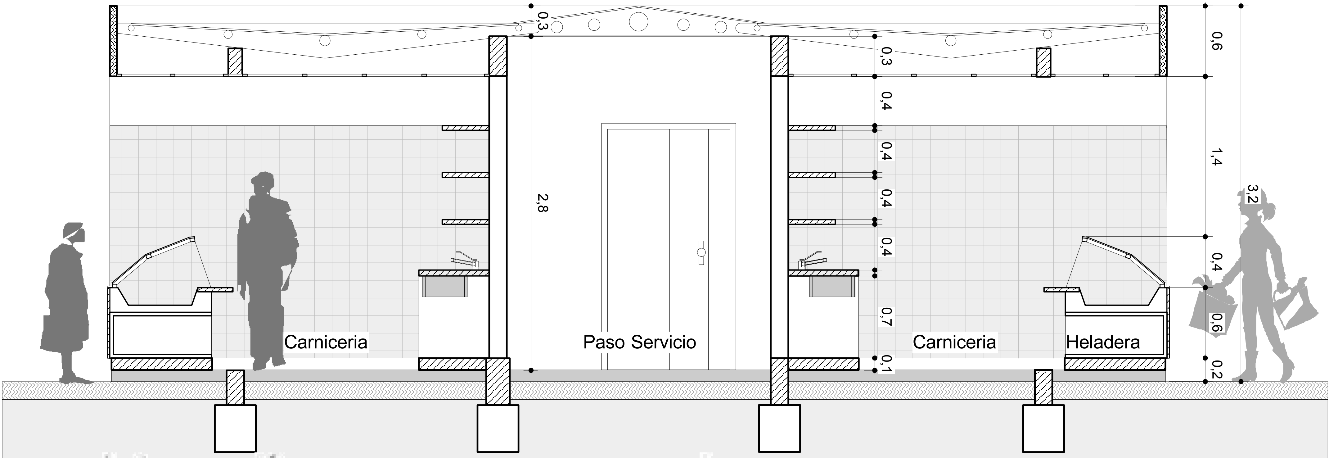
CORTE TRANSVERSAL.
