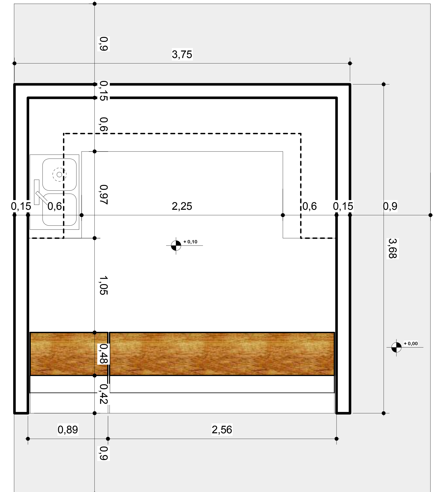
PLANTA ACOTADA ESC. 1:20
