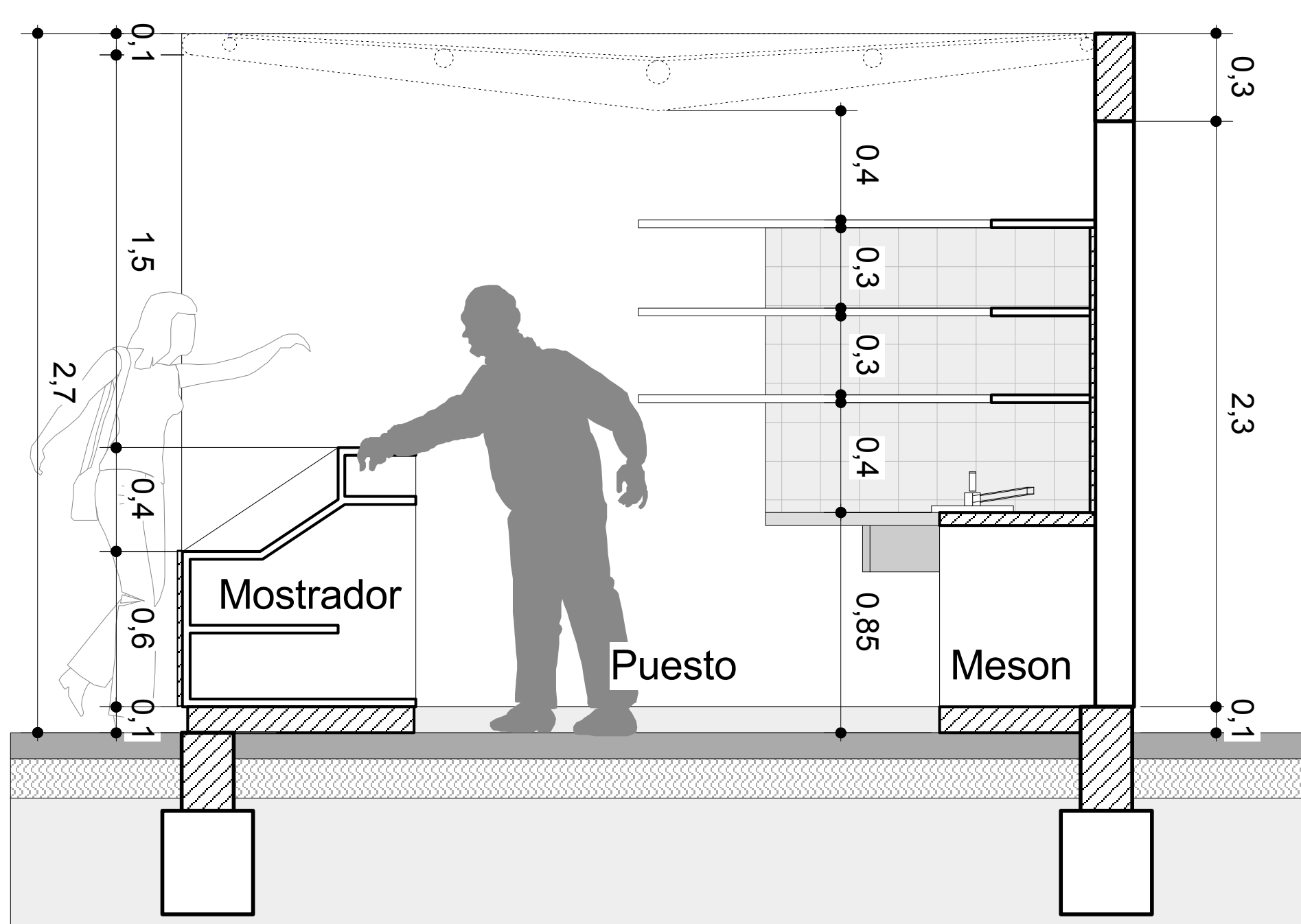
CORTE TRANSV.
