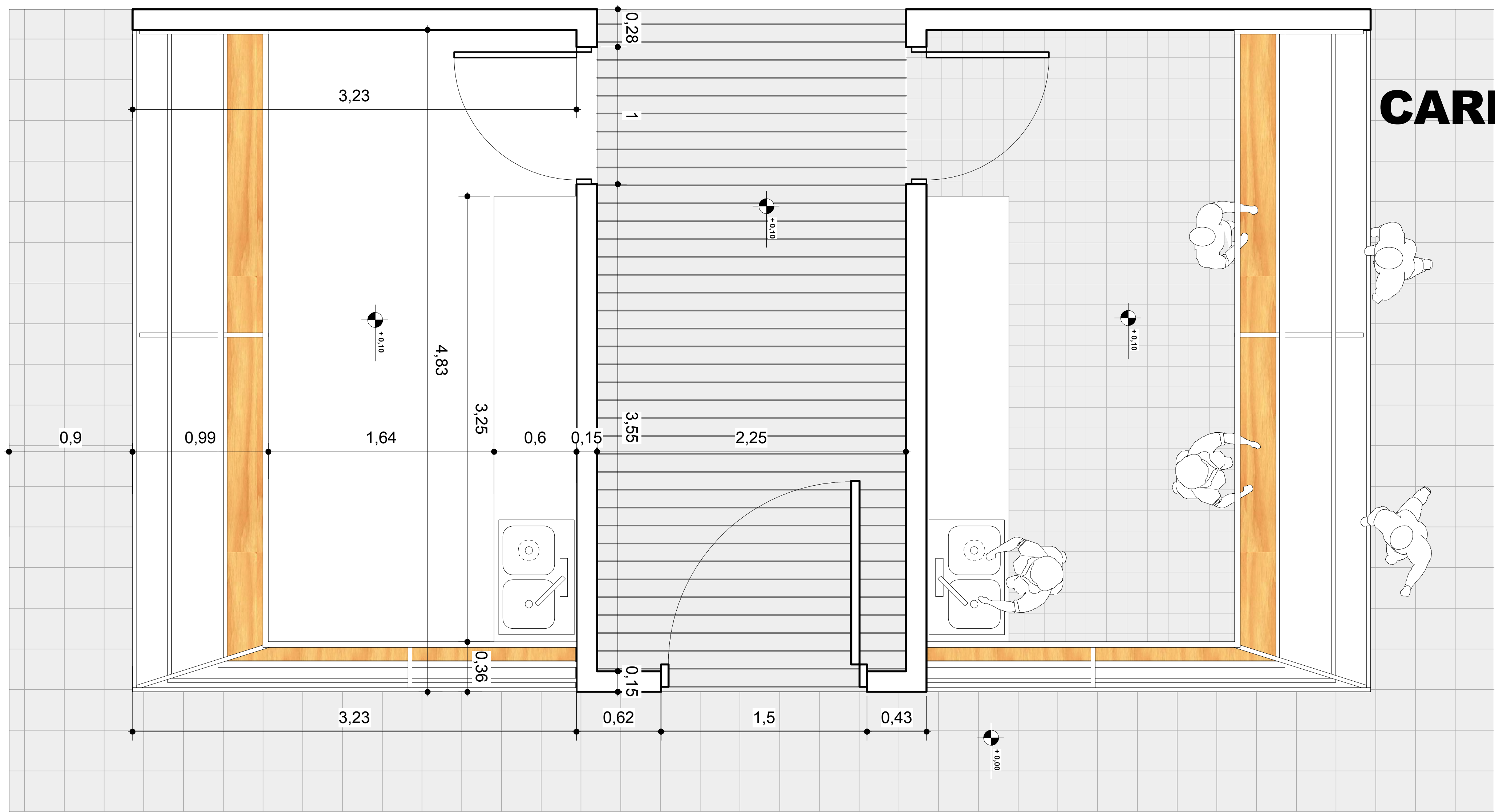
PLANTA ACOTADA ESC. 1:20
