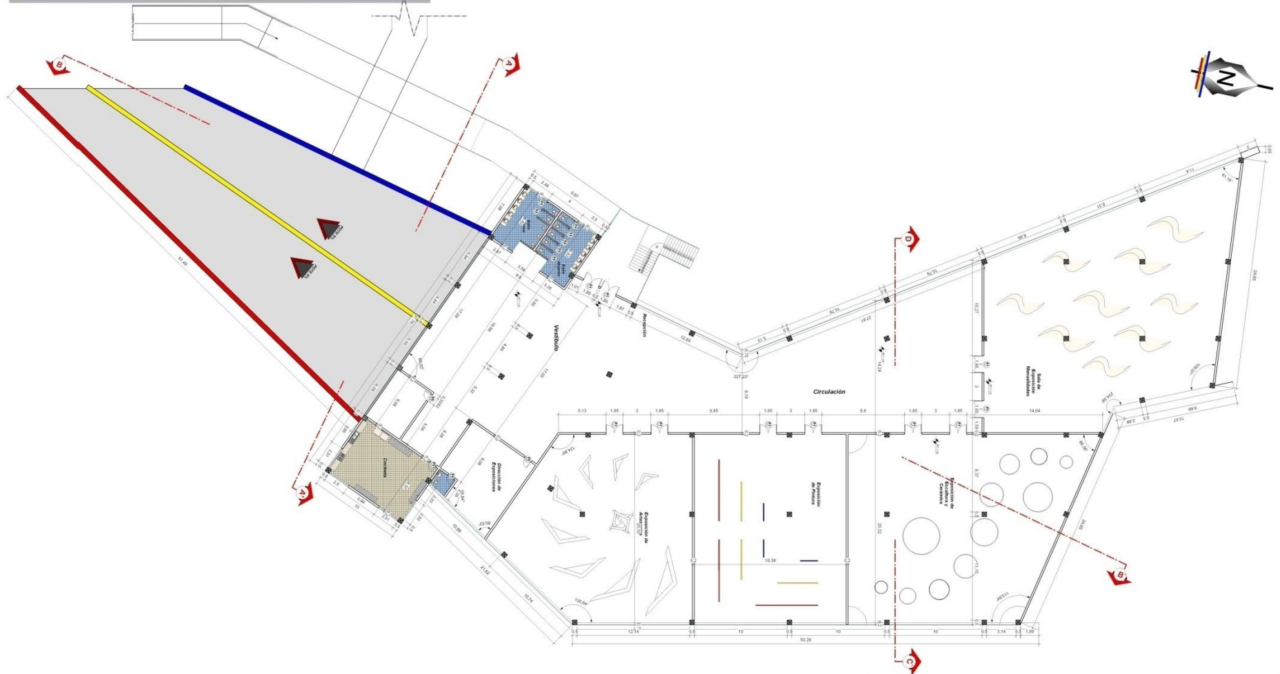
PLANTA SEGUNDO PISO ACOTADA BLOQUE EDUCATIVO - ADMINISTRATIVO
