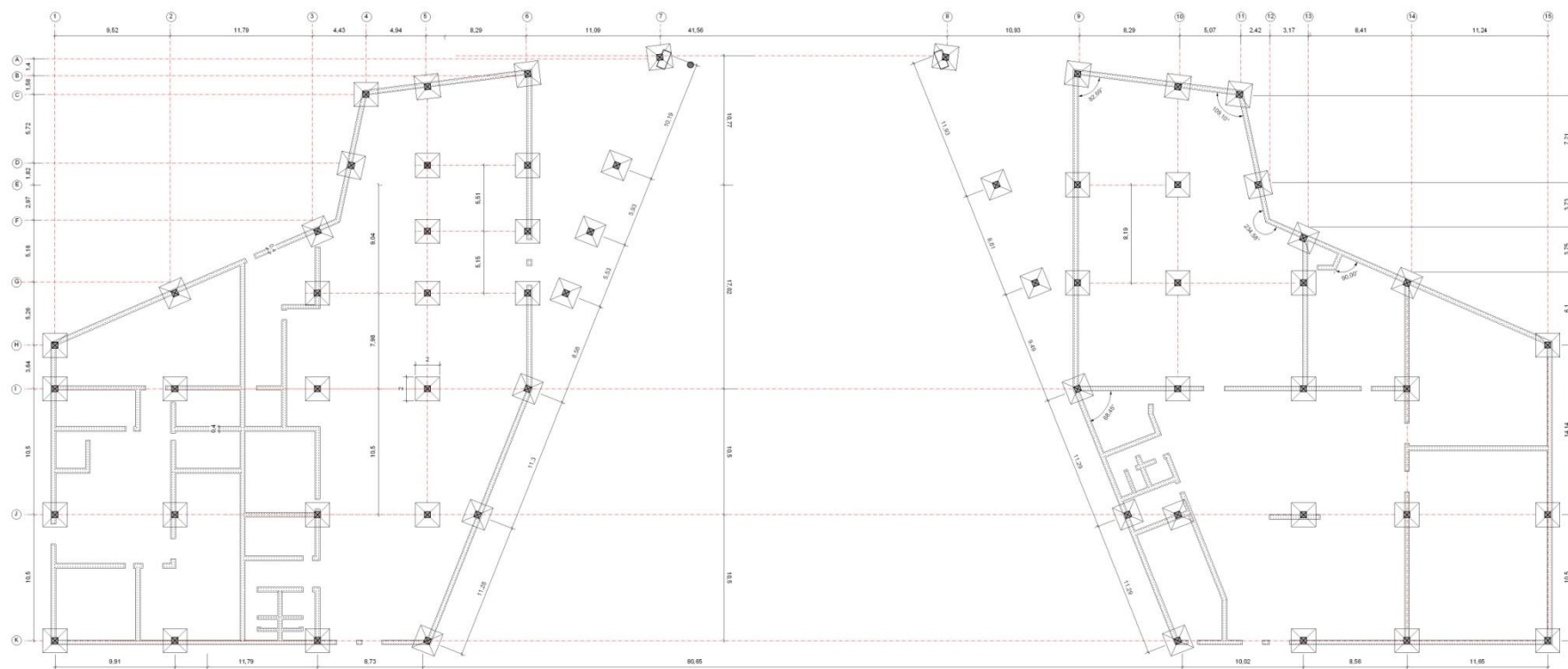
PLANTA DE CIMIENTOS
