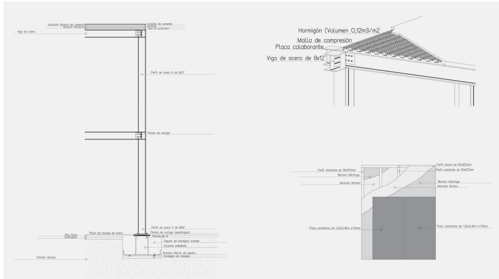
Figura 65 Corte de borde (acero)
