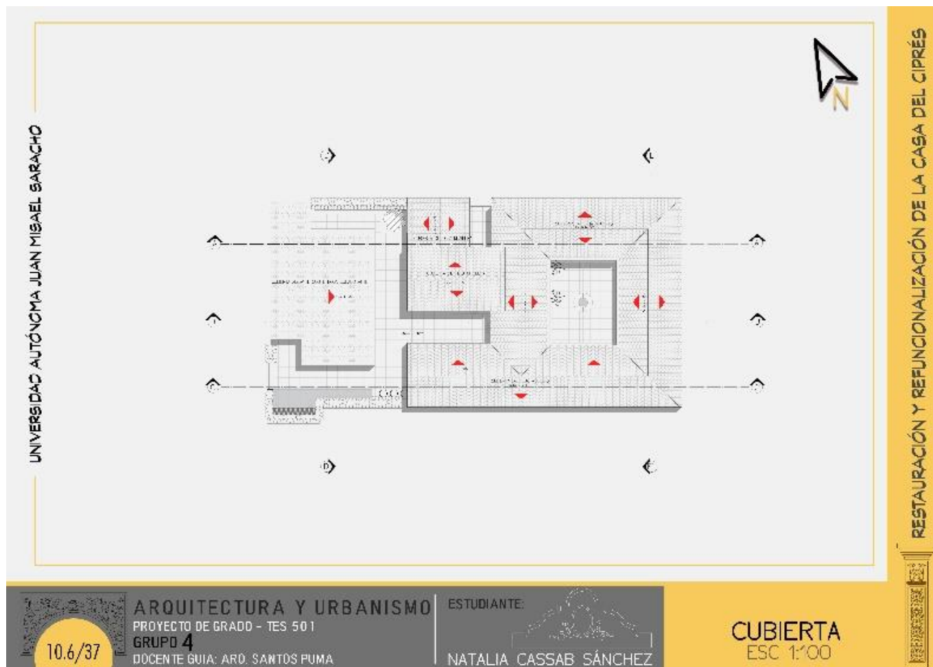
Figura 61 Plano de cubiertas
