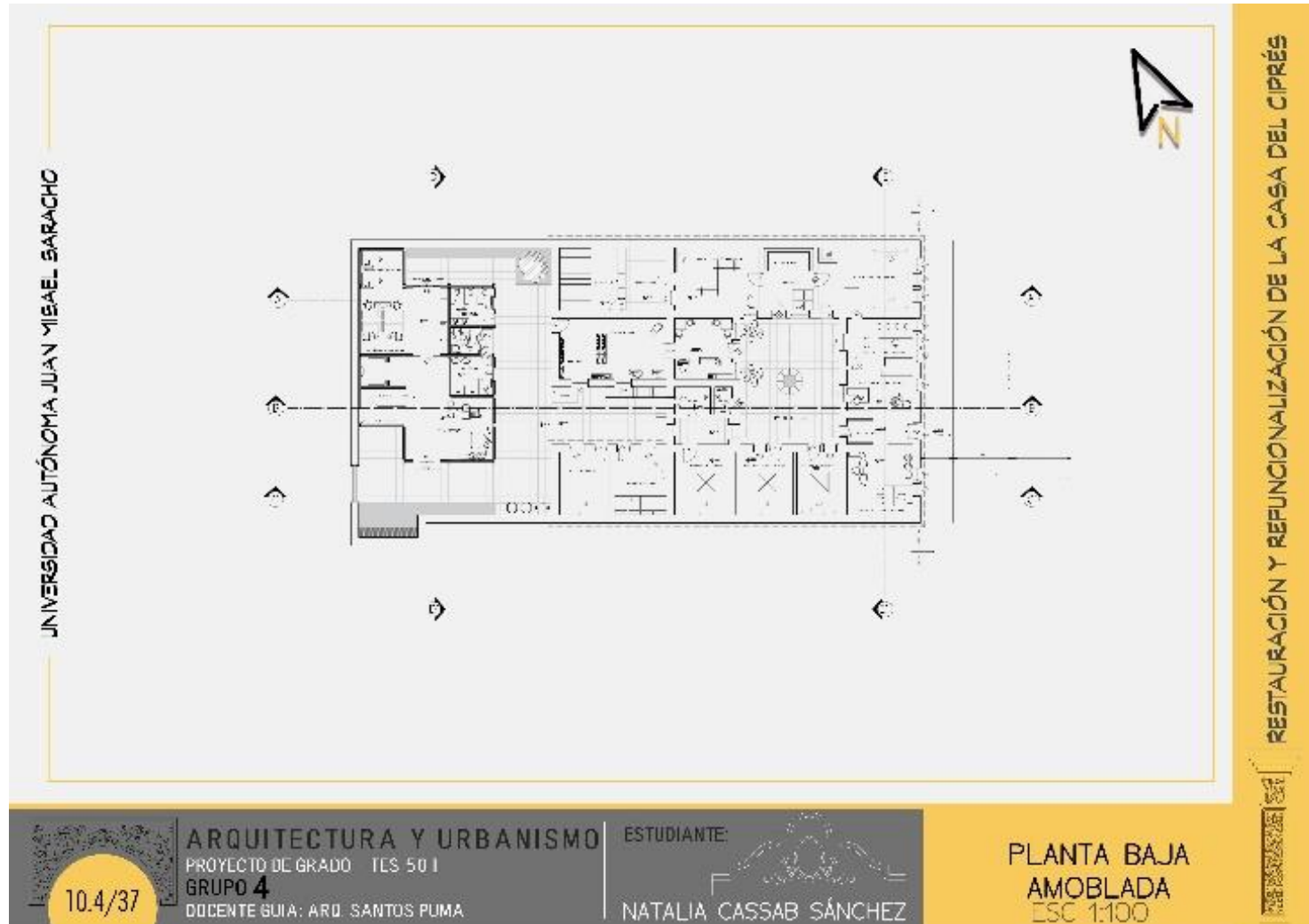
Figura 59 Planta baja amoblada
