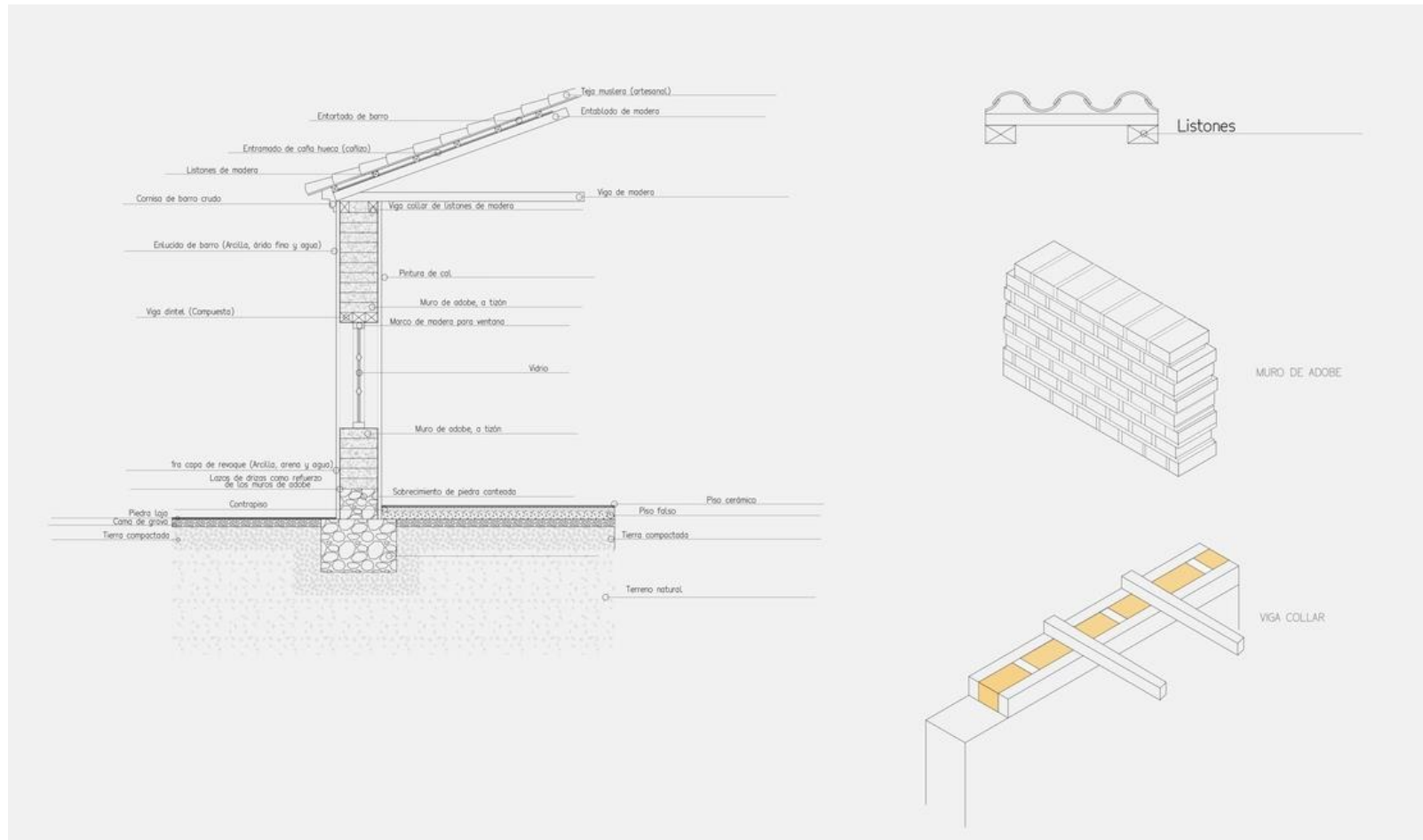
Figura 64 Corte de borde (adobe)
