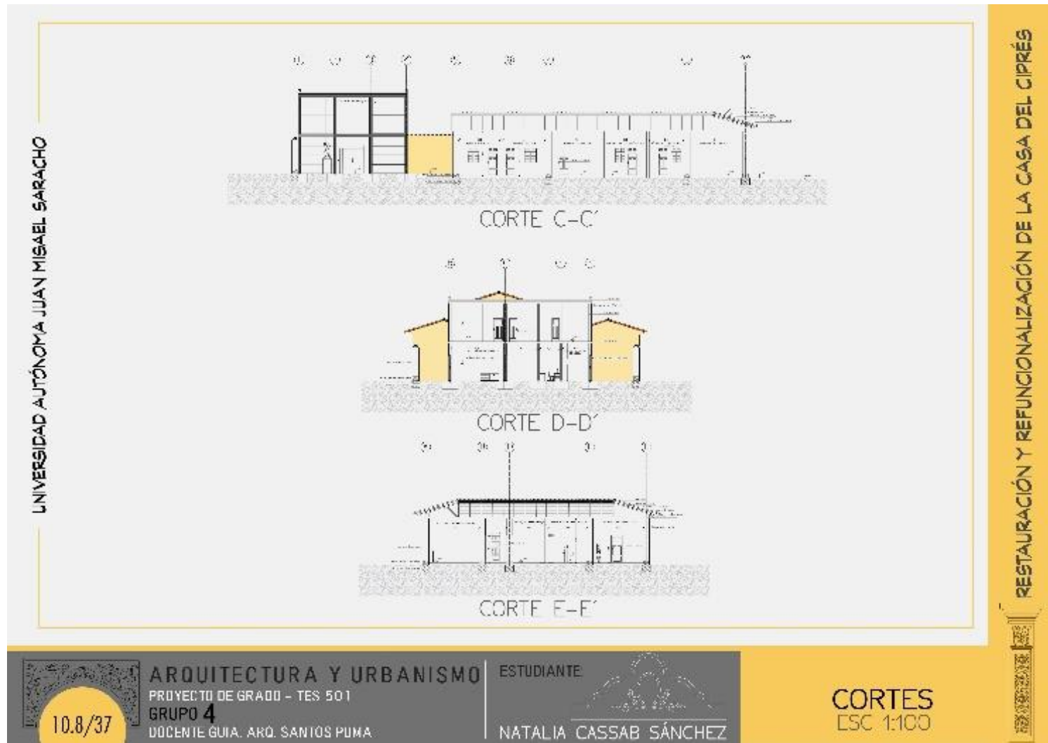
Figura 63 Cortes transversales
