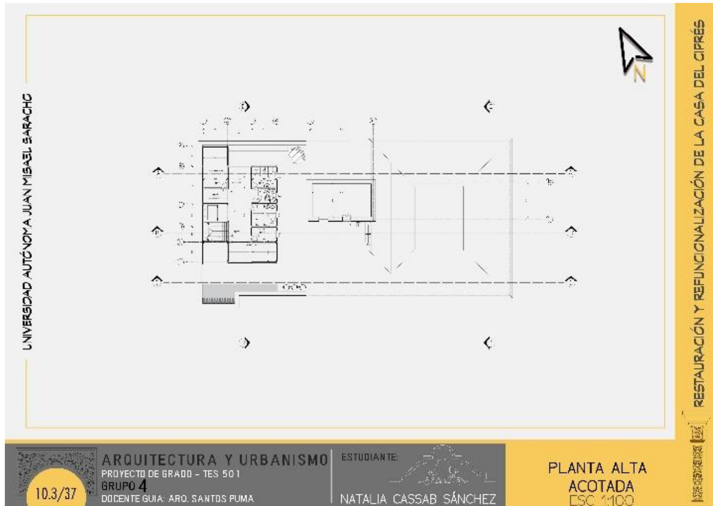
Figura 58 Planta alta acotada
