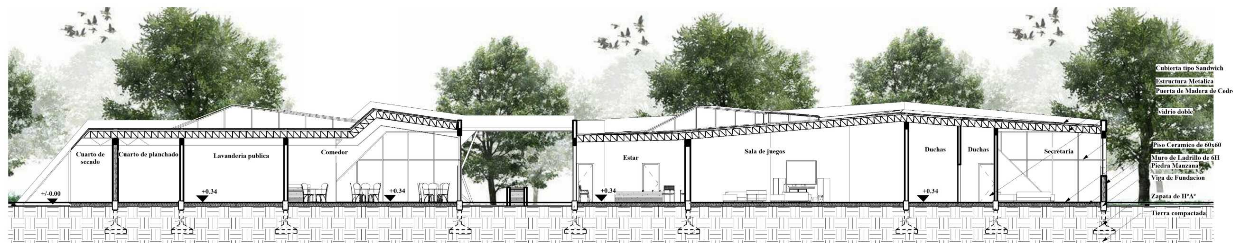
CORTE C-C"
