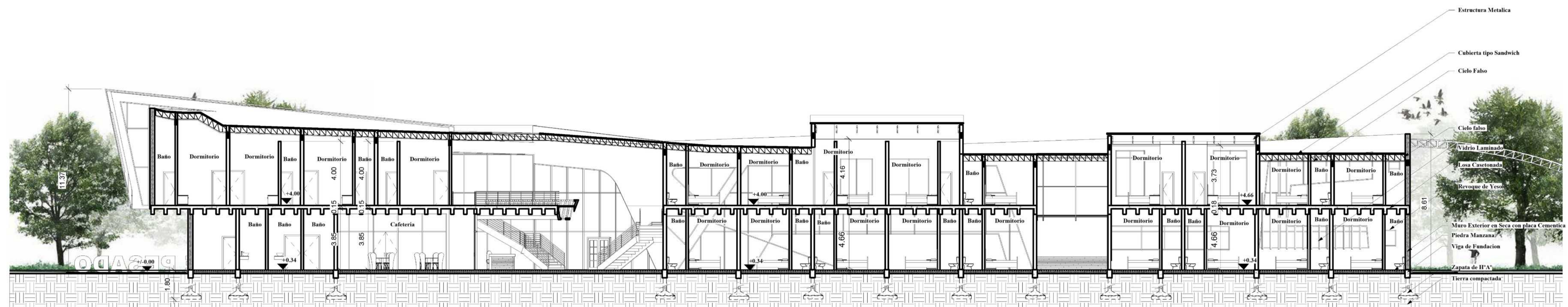
CORTE A-A"
