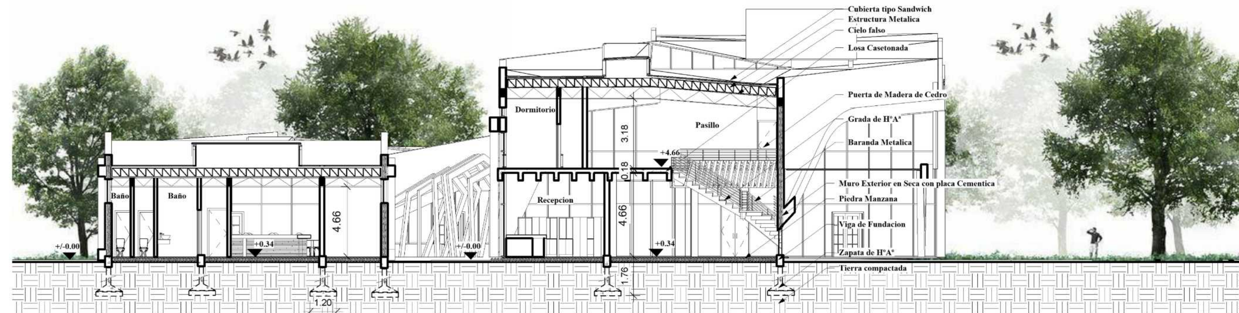
CORTE B-B"
