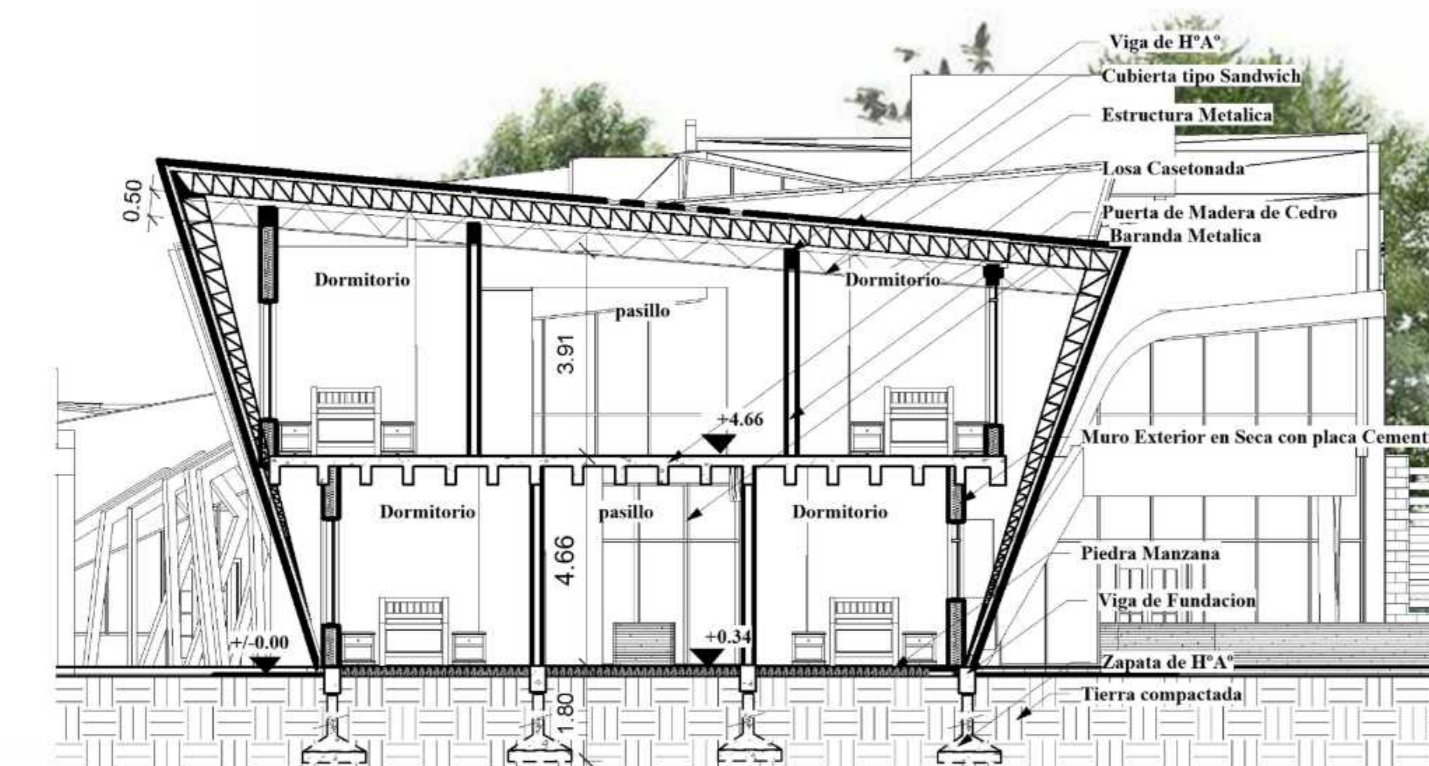
CORTE D-D"
